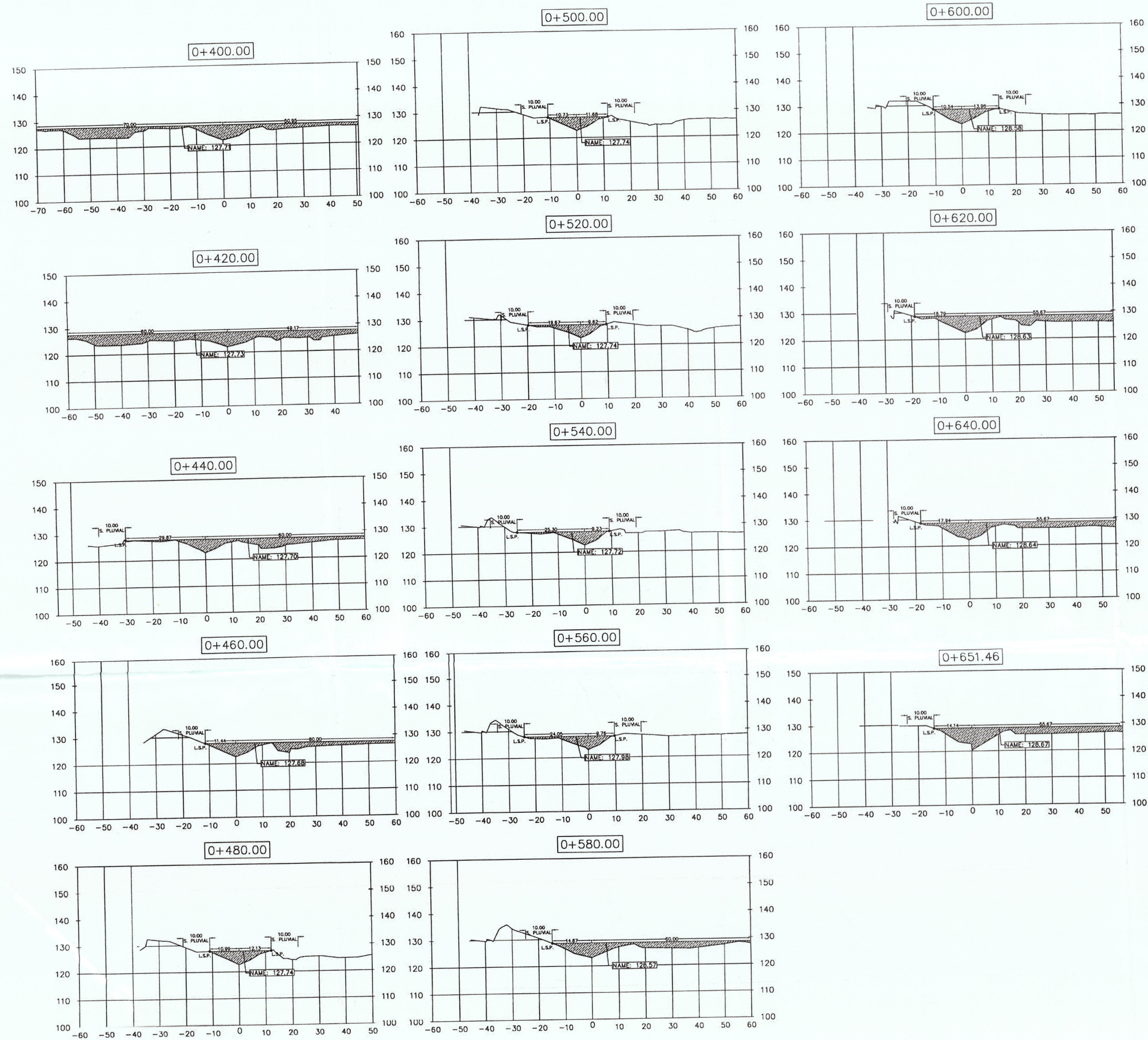
SECCIONES TRANSVERSALES ESCALA: 1:750
