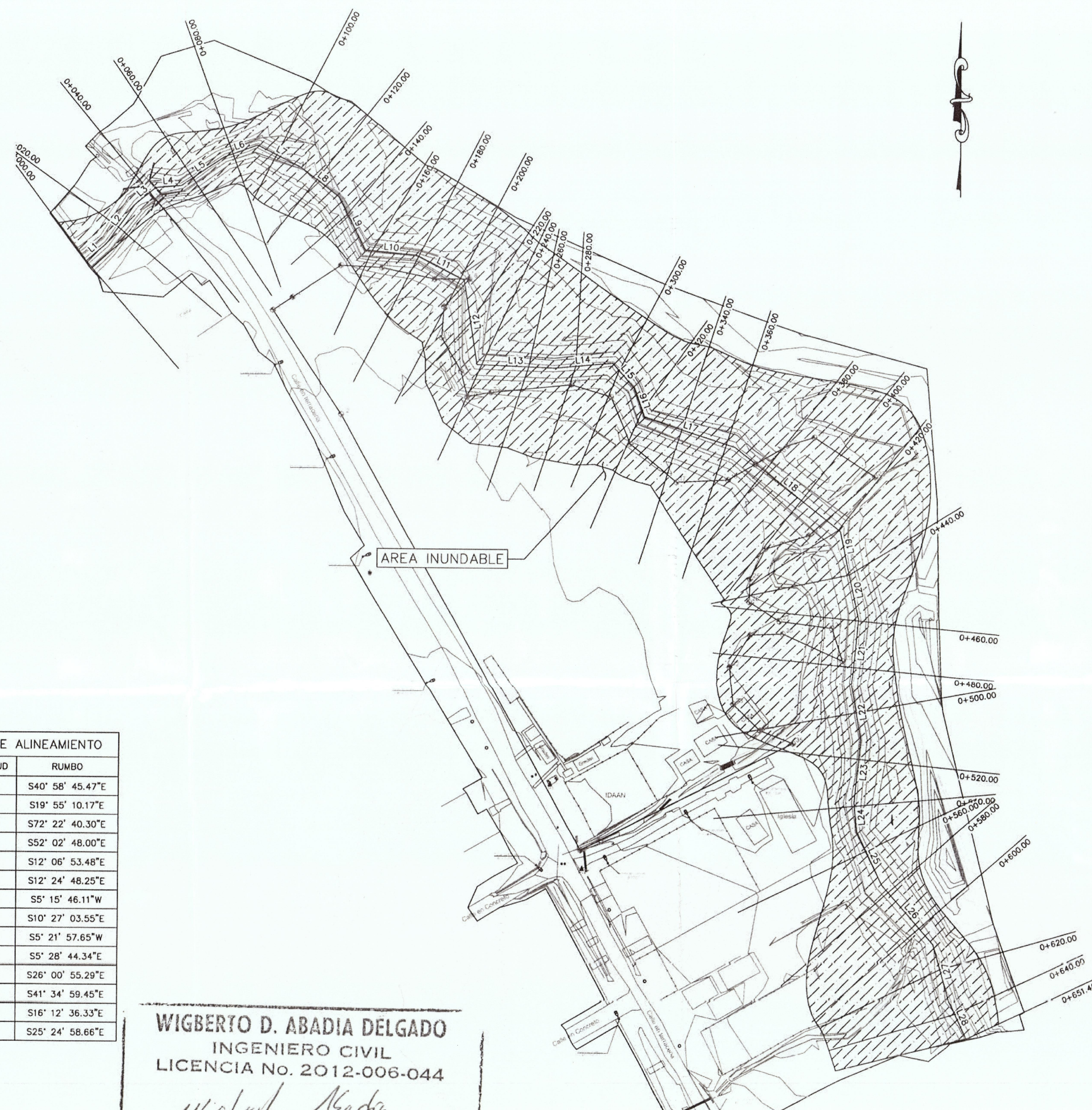
PLANTA GENERAL DEL POLIGONO DE ESTUDIO ESCALA 1:1000
