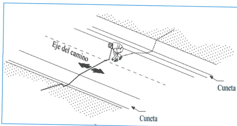
Diseño de zanjas o cunetas de tierra sin revestimiento a construir en los caminos
