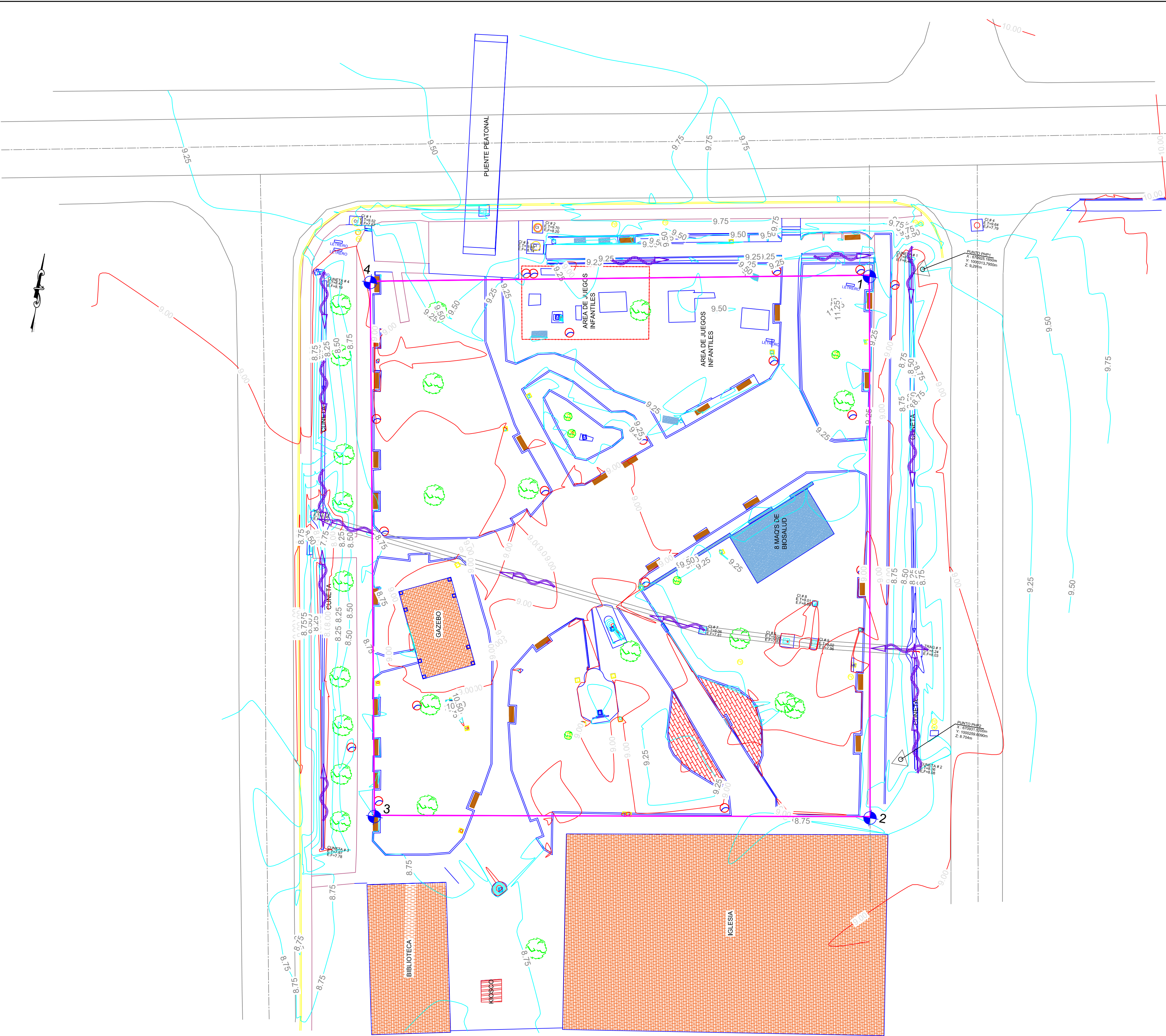
LOCALIZACION GENERAL ESC. 1:250
