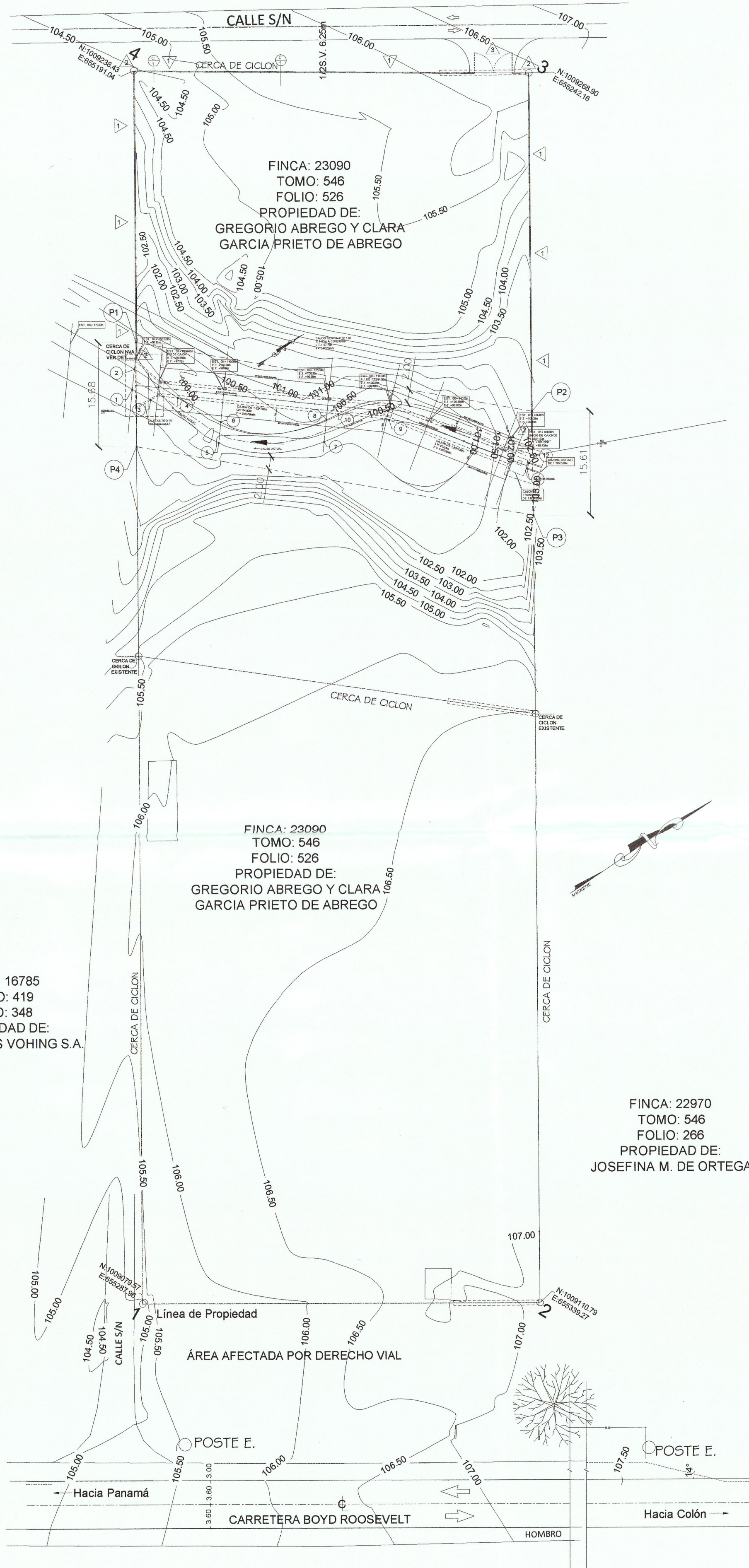
PLANTA GENERAL ESCALA 1:400
