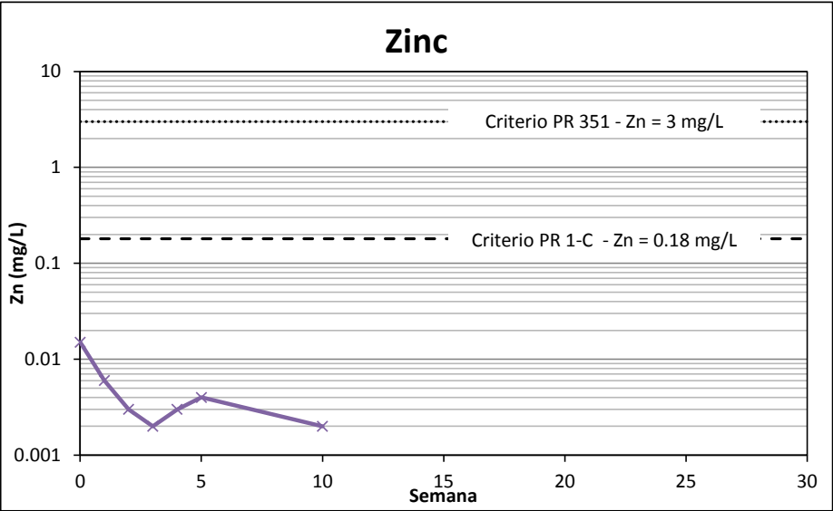
Figura 6-9 Resultados de Celdas de Humedad para Muestra 2014-CG-057 Proyecto Cerro Quema
