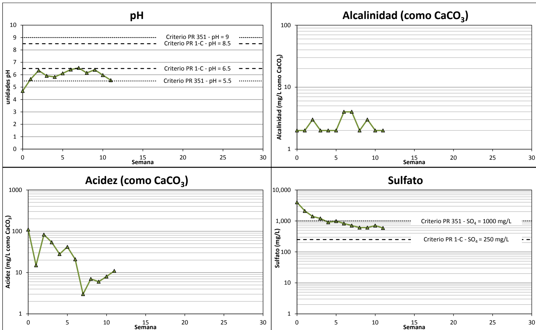
Figura 6-8 Resultados de Celdas de Humedad para Muestra 2014-CG-055 Proyecto Cerro Quema
