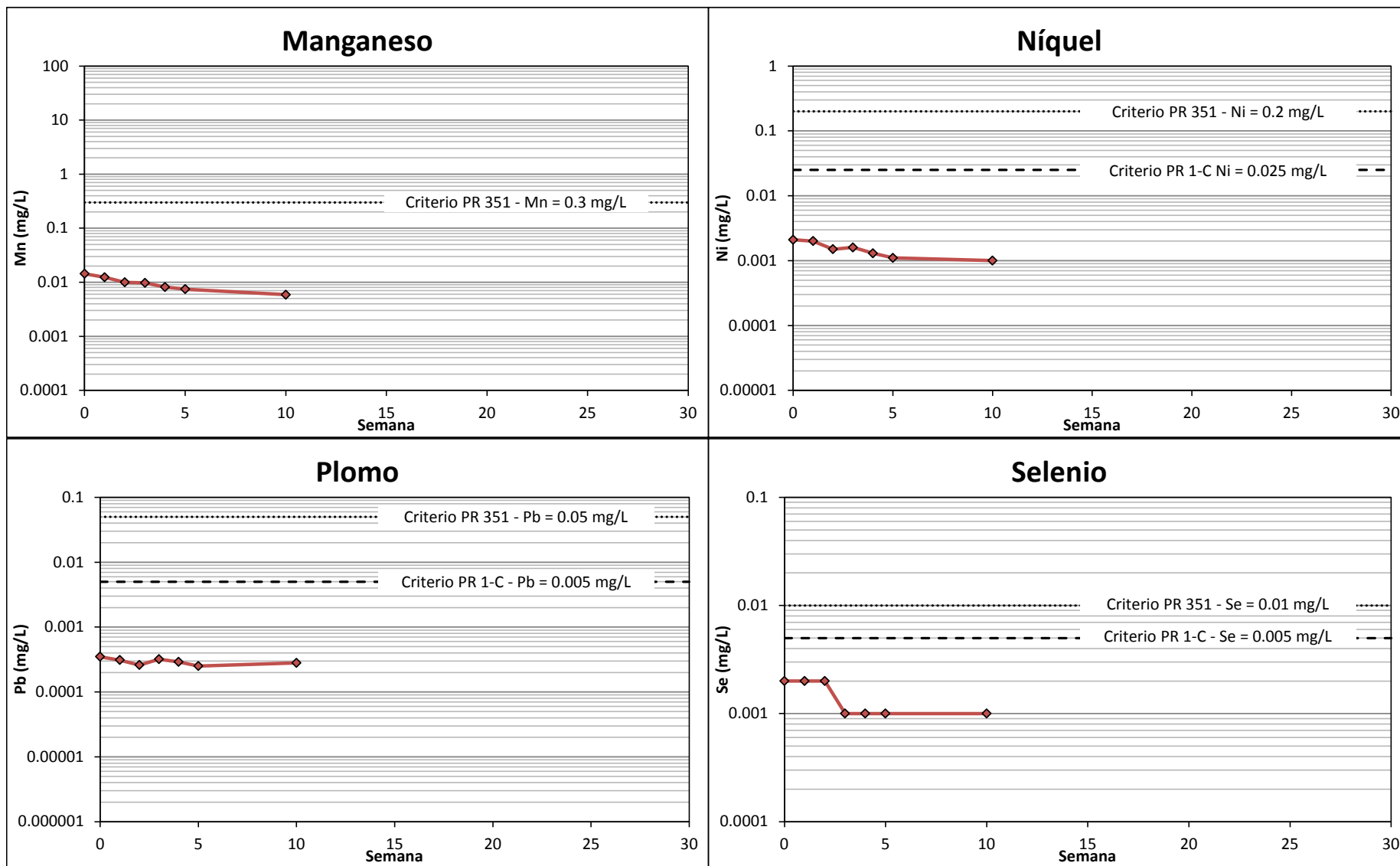
Figura 6-7 Resultados de Celdad de Humedad para Muestra 2014-CG-053 Proyecto Cerro Quema
