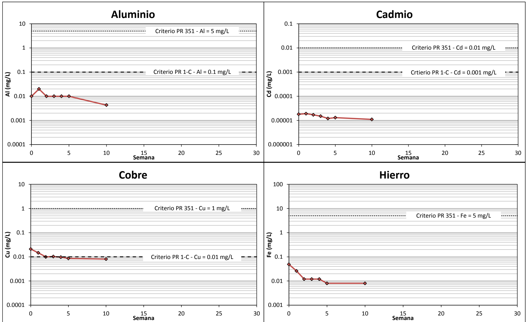
Figura 6-7 Resultados de Celdas de Humedad para Muestra 2014-CG-053 Proyecto Cerro Quema
