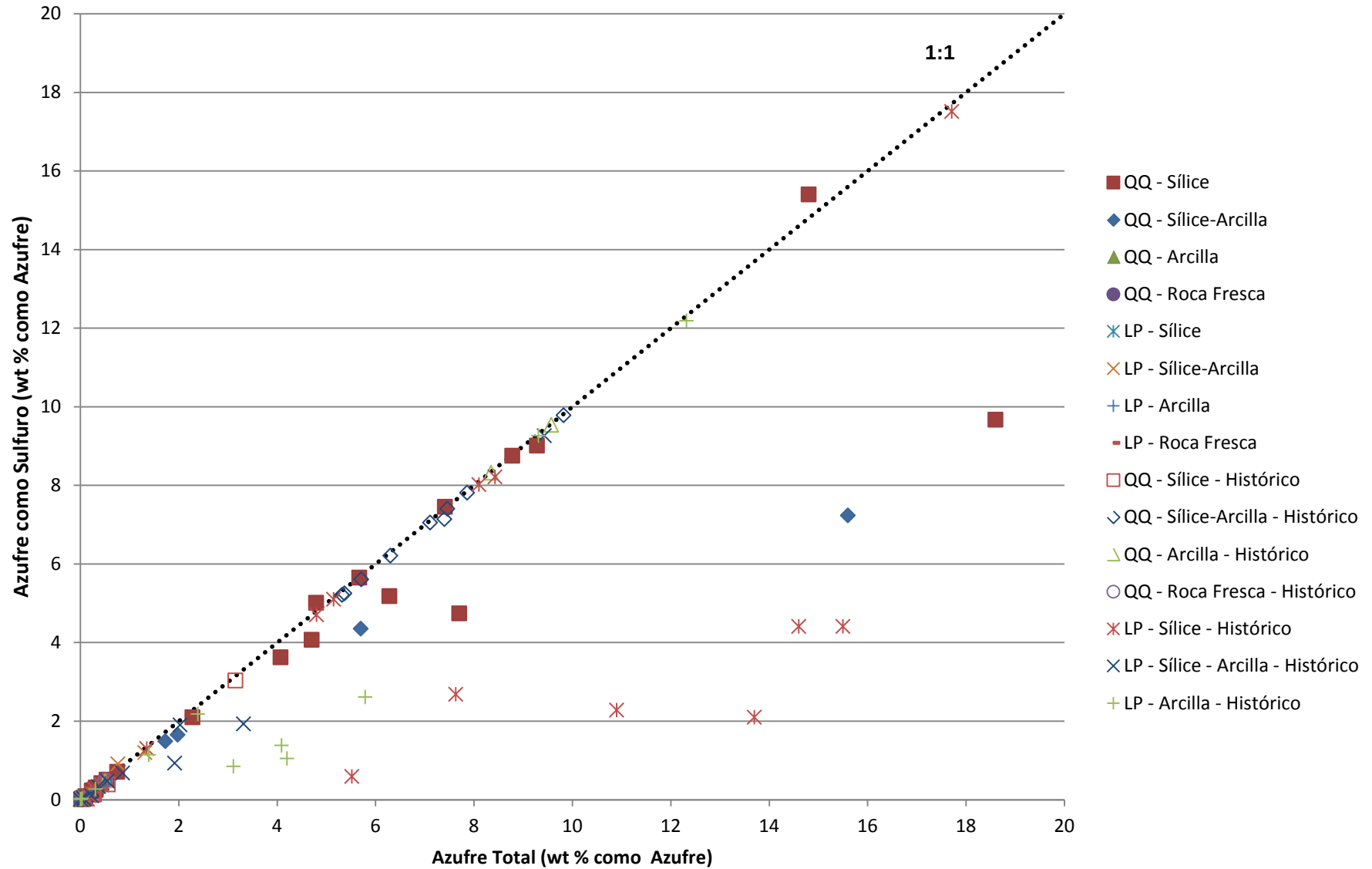
Figura 6-2 Azufre Total vs Azufre como Sulfuro Proyecto Cerro Quema
