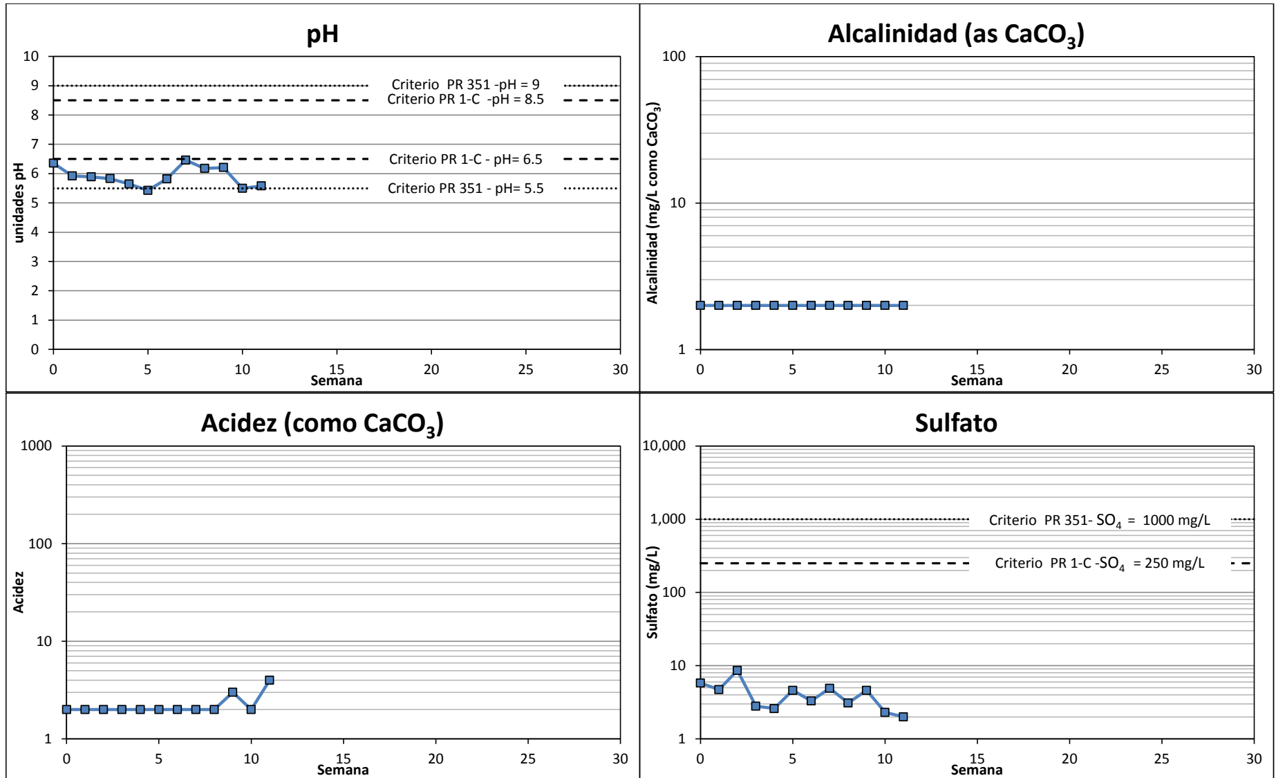
Figura 6-6 Resultados de Celda de Humedad para Muestra 2014-CG-041 Proyecto Cerro Quema
