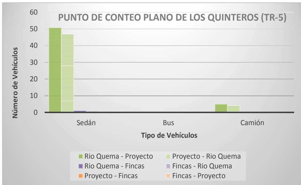
Gráfico 4-10: Número de Vehículos Promedio Diario según el Sentido de Flujo Vehicular – Plano de los Quinteros
