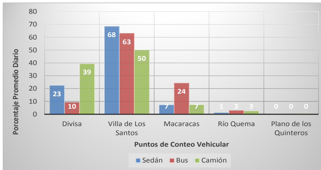
Gráfico 4-11: Porcentaje de Distribución Promedio Diario de Tipo de Vehículos por Punto de Conteo
