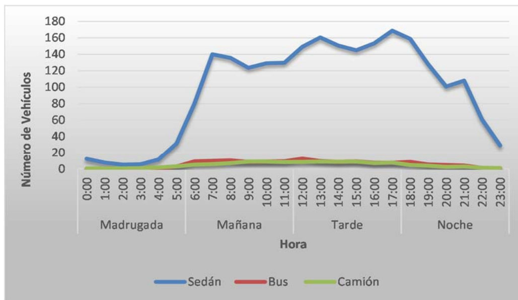
Gráfico 4-14: Distribución Promedio Horaria por Tipo de Vehículo – Macaracas (TR-3)
