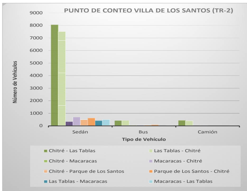
Gráfico 4-7: Número de Vehículos Promedio Diario según el Sentido de Flujo Vehicular – Villa de Los Santos
