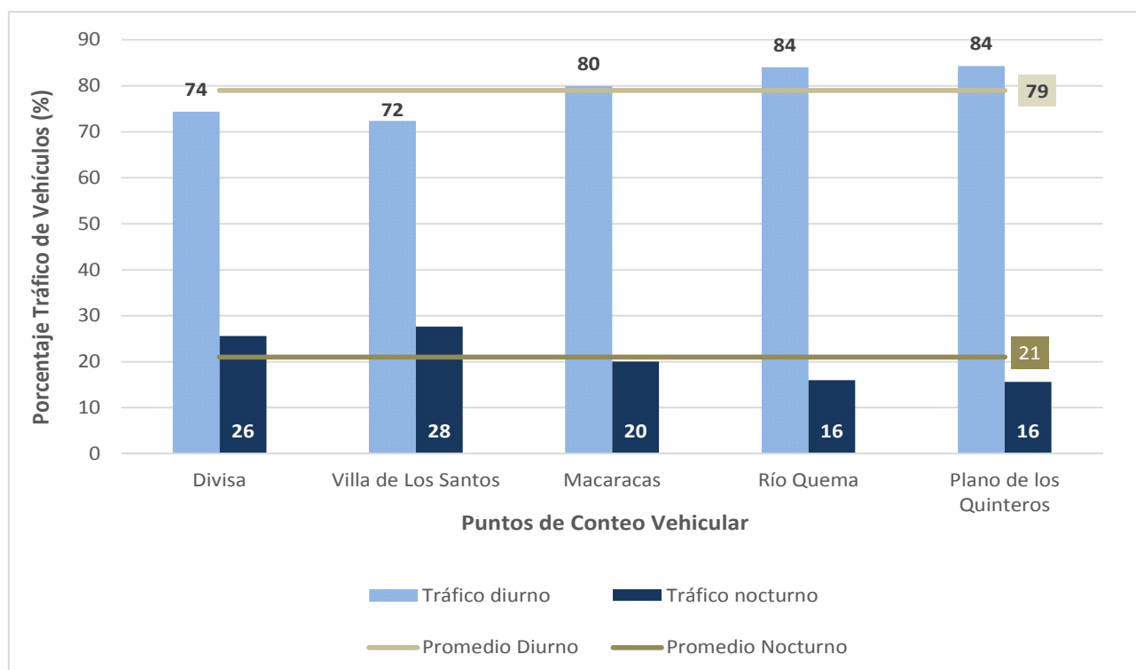
Gráfico 4-4: Porcentaje de Distribución Promedio de Tráfico Vehicular Diurno y Nocturno
