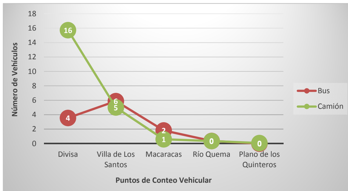
Gráfico 4-3: Volumen de Vehículos Promedio Horario por Punto de Conteo - Buses y Camiones
