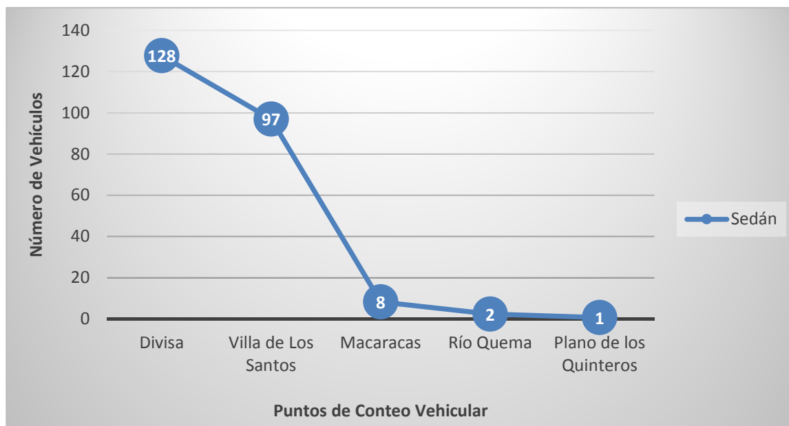
Gráfico 4-2: Volumen de Vehículos Promedio Horario por Punto de Conteo - Sedán
