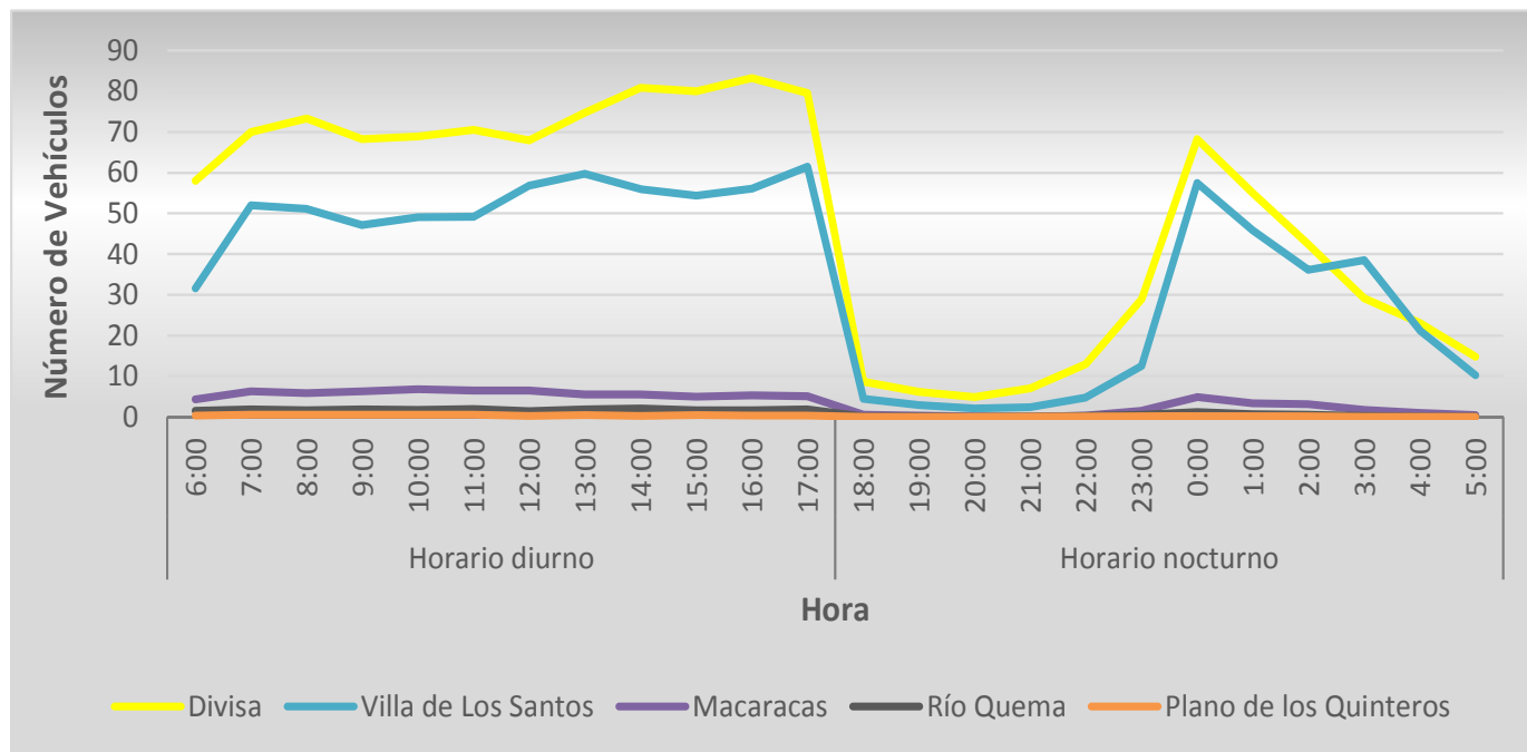
Gráfico 4-5: Distribución Horario de Volumen de Tráfico Promedio por Punto de Conteo
