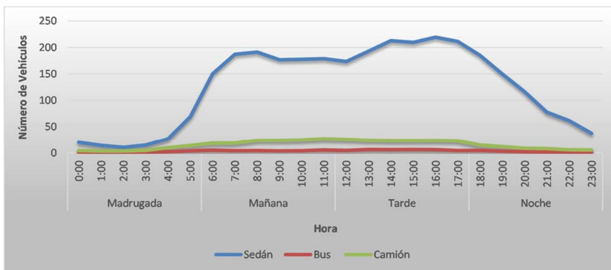
Gráfico 4-12: Distribución Promedio Horaria por Tipo de Vehículo – Divisa (TR-1)
