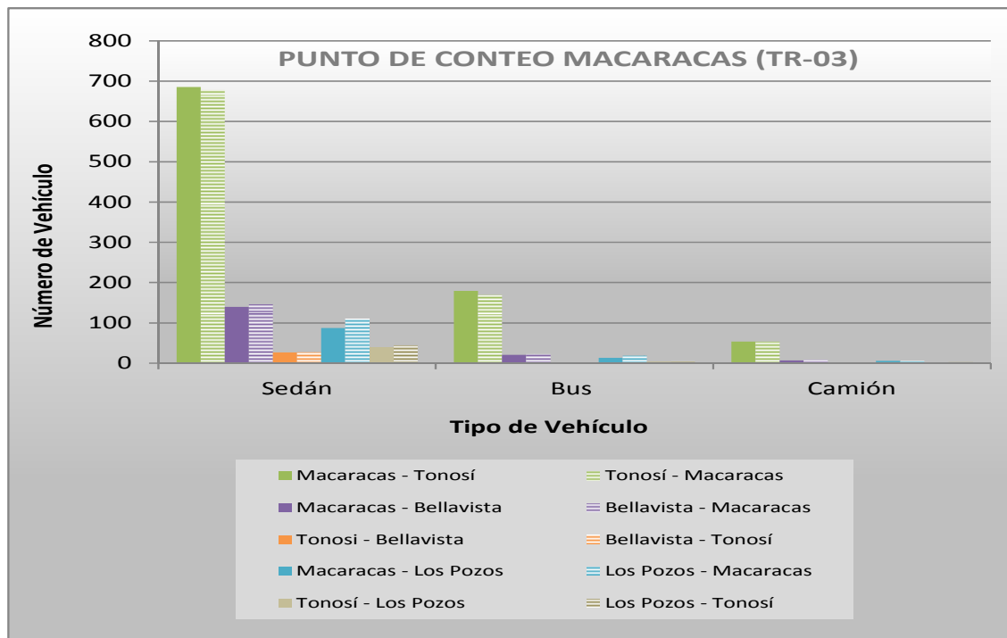
Gráfico 4-9: Número de Vehículos Promedio Diario según el Sentido de Flujo Vehicular – Río Quema
