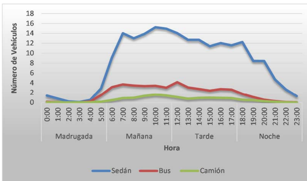
Gráfico 4-14: Distribución Promedio Horaria por Tipo de Vehículo – Macaracas (TR-3)
