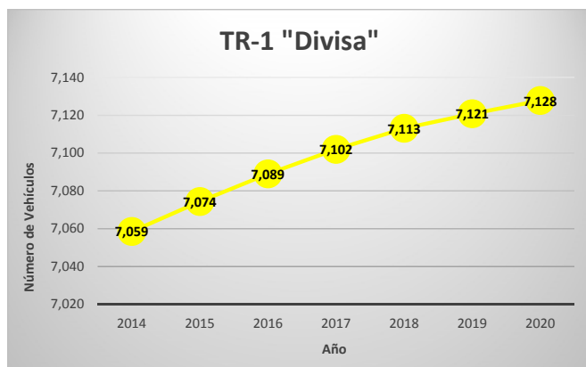
Gráfico 5-1: Proyección de Tráfico Vehicular Anual por cada punto de Conteo
