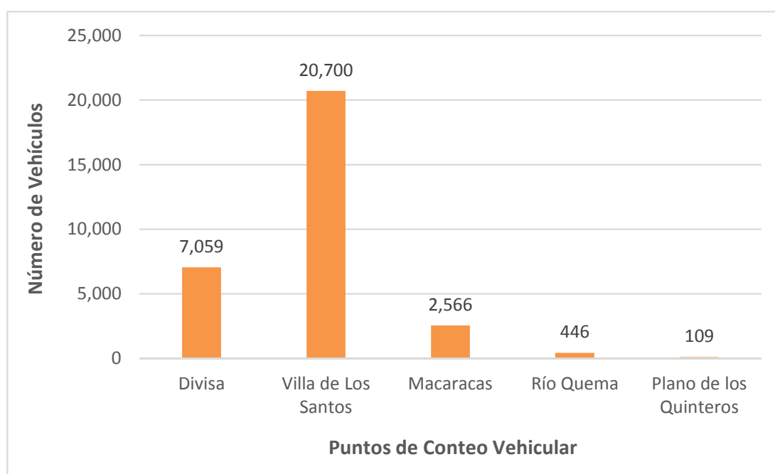
Gráfico 4-1: IMDA por Punto de Conteo
