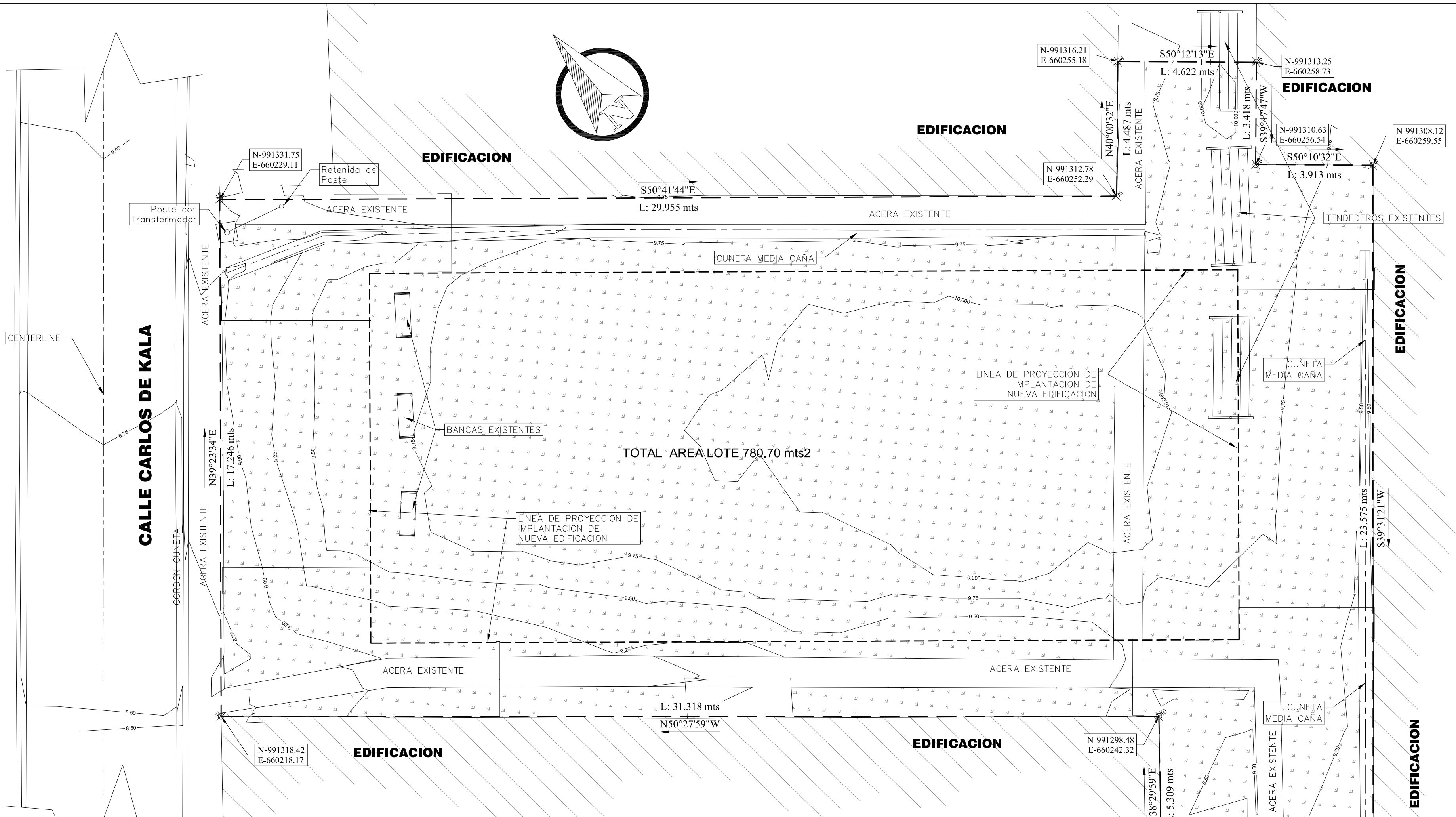
PLANTA DE TOPOGRAFIA ACTUAL ESC. 1:100
