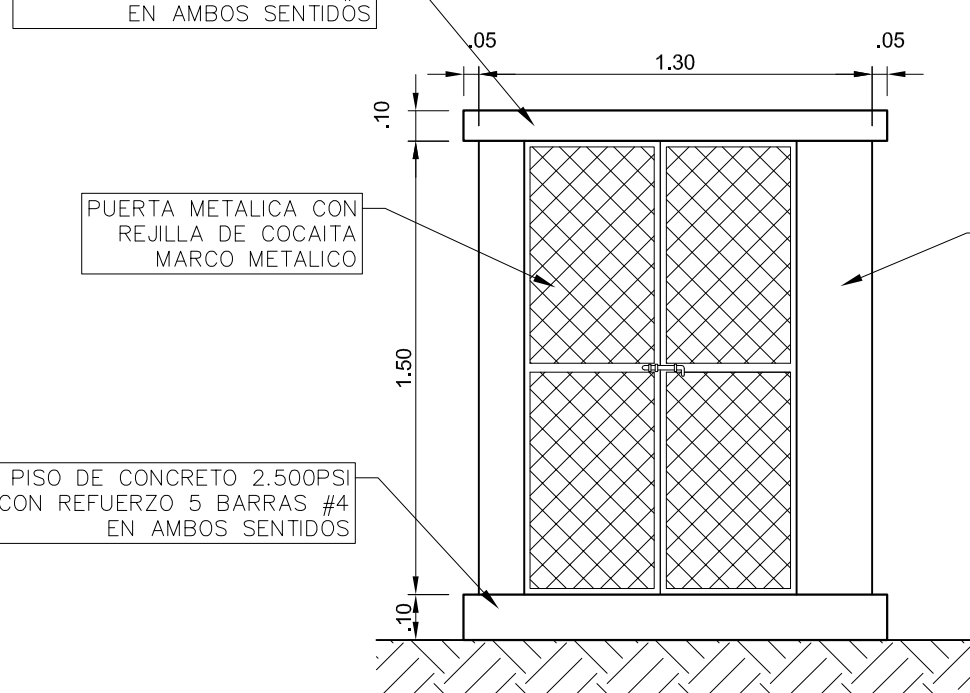
TINAQUERA-ALZADO FRONTAL ESC. 1:25
