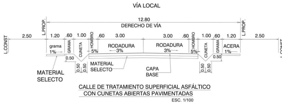
Ilustración No. 1. Secciones de vía
