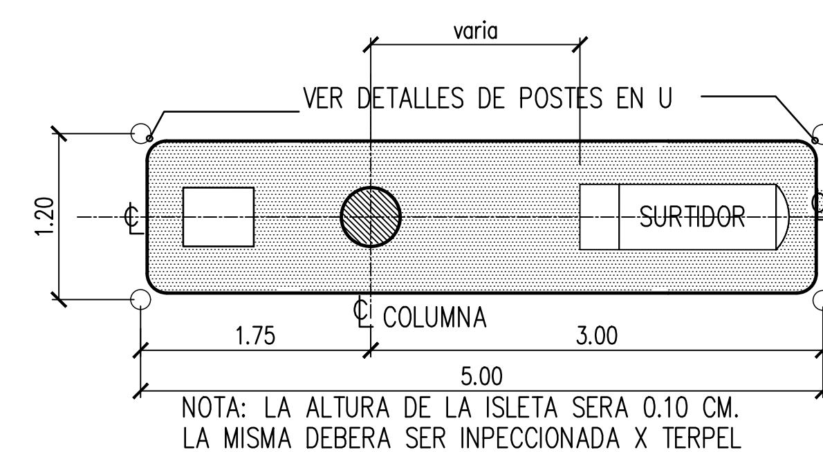
DETALLE DE ISLETAS TÍPICAS ESC. 1:50 Mts.
