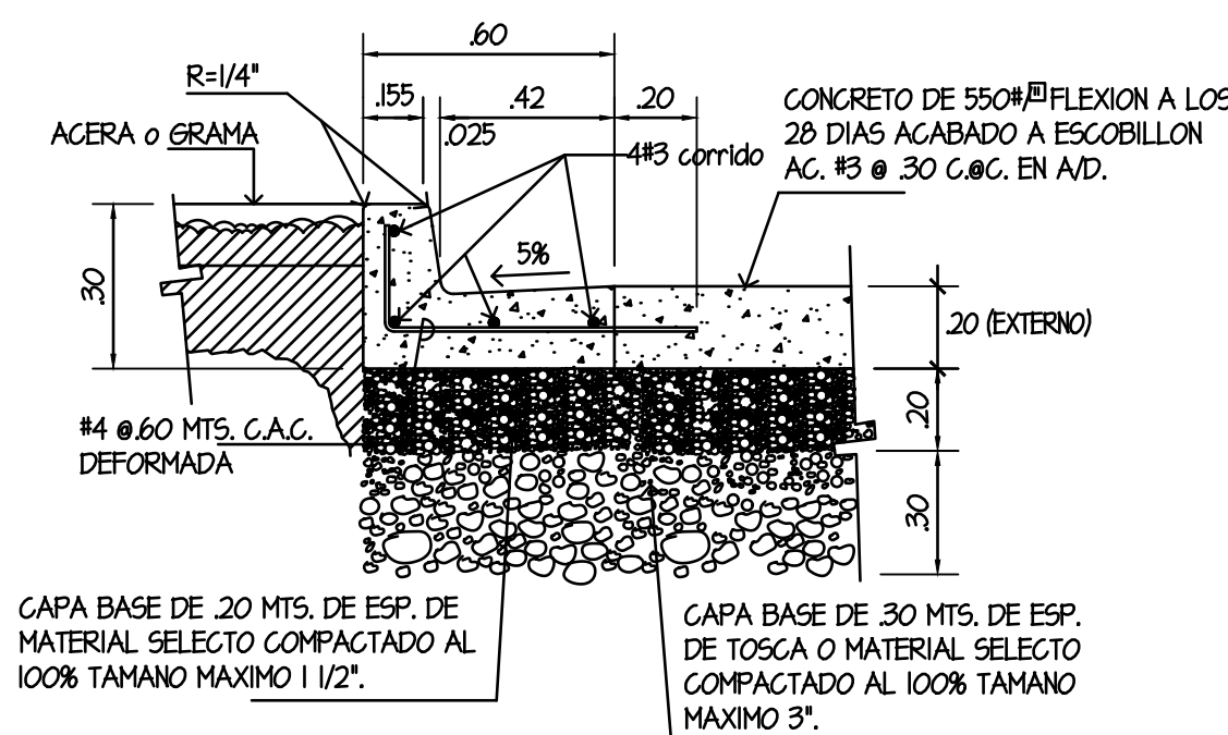
DETALLE 2 ESCALA 1:20 M. CORDON AR-1
