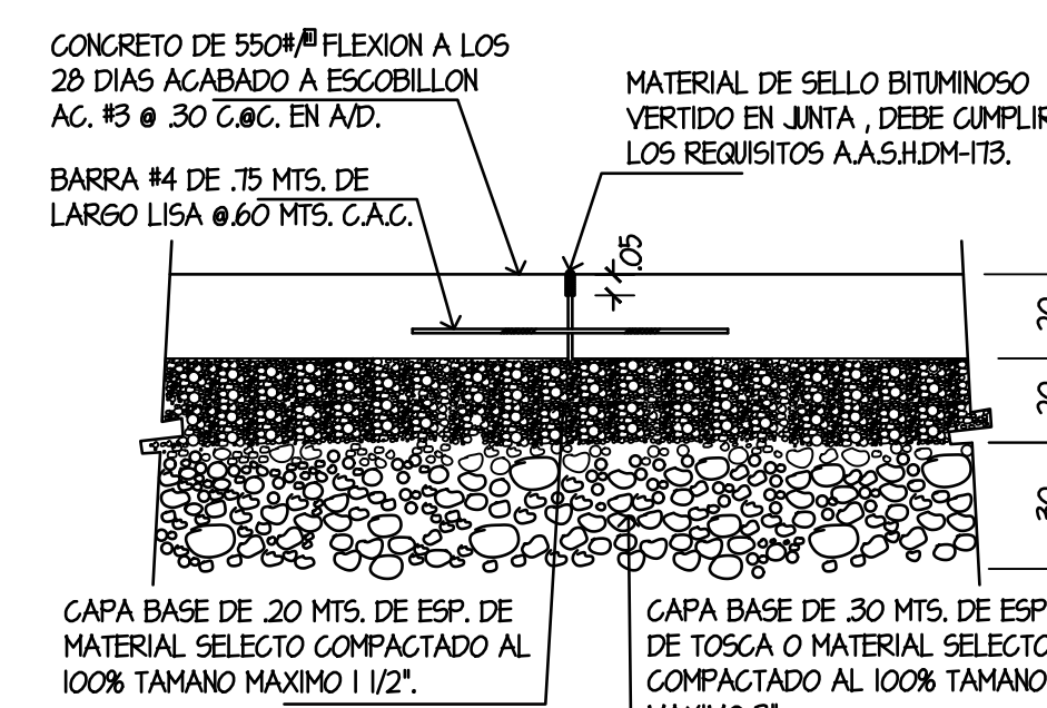
DETALLE ESCALA 1:20 M. JUNTA DE CONSTRUCCION 3 AR-I
