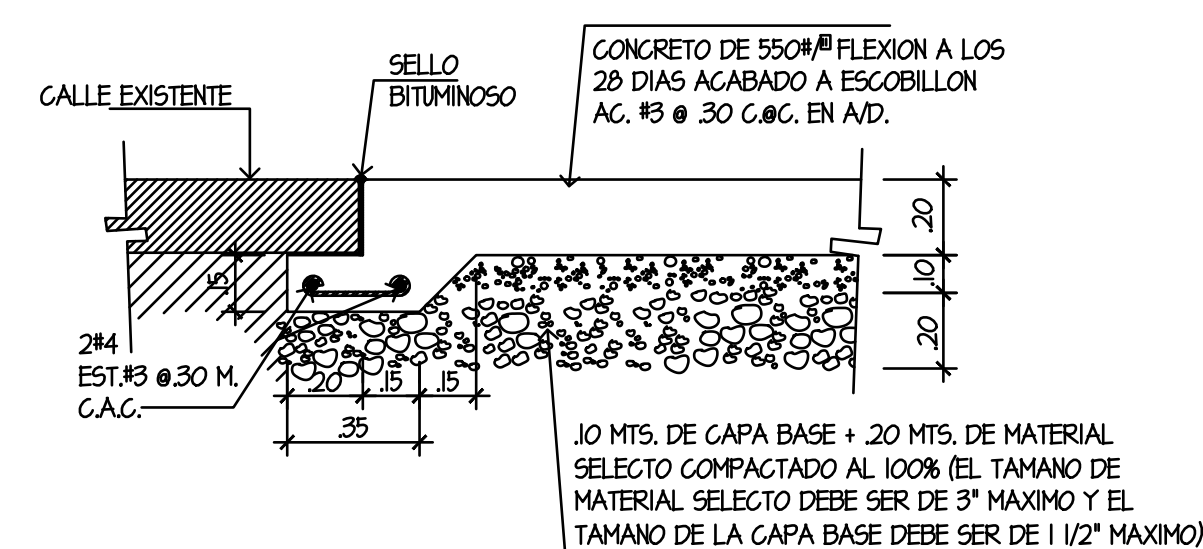
DETALLE ESCALA 1:20 M. DETALLE DE EMPALME DE PAVIMENTO NUEVO CON EXISTENTE 1 AR-1
