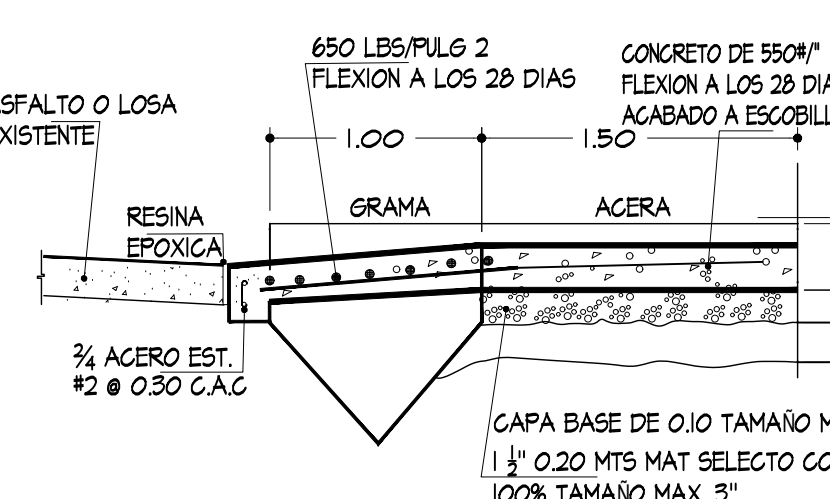
ELEVACION LATERAL IZQUIERDA 1 DETALLE RECOMENDADOS POR EL MOP AR-1 SIN VISC.
