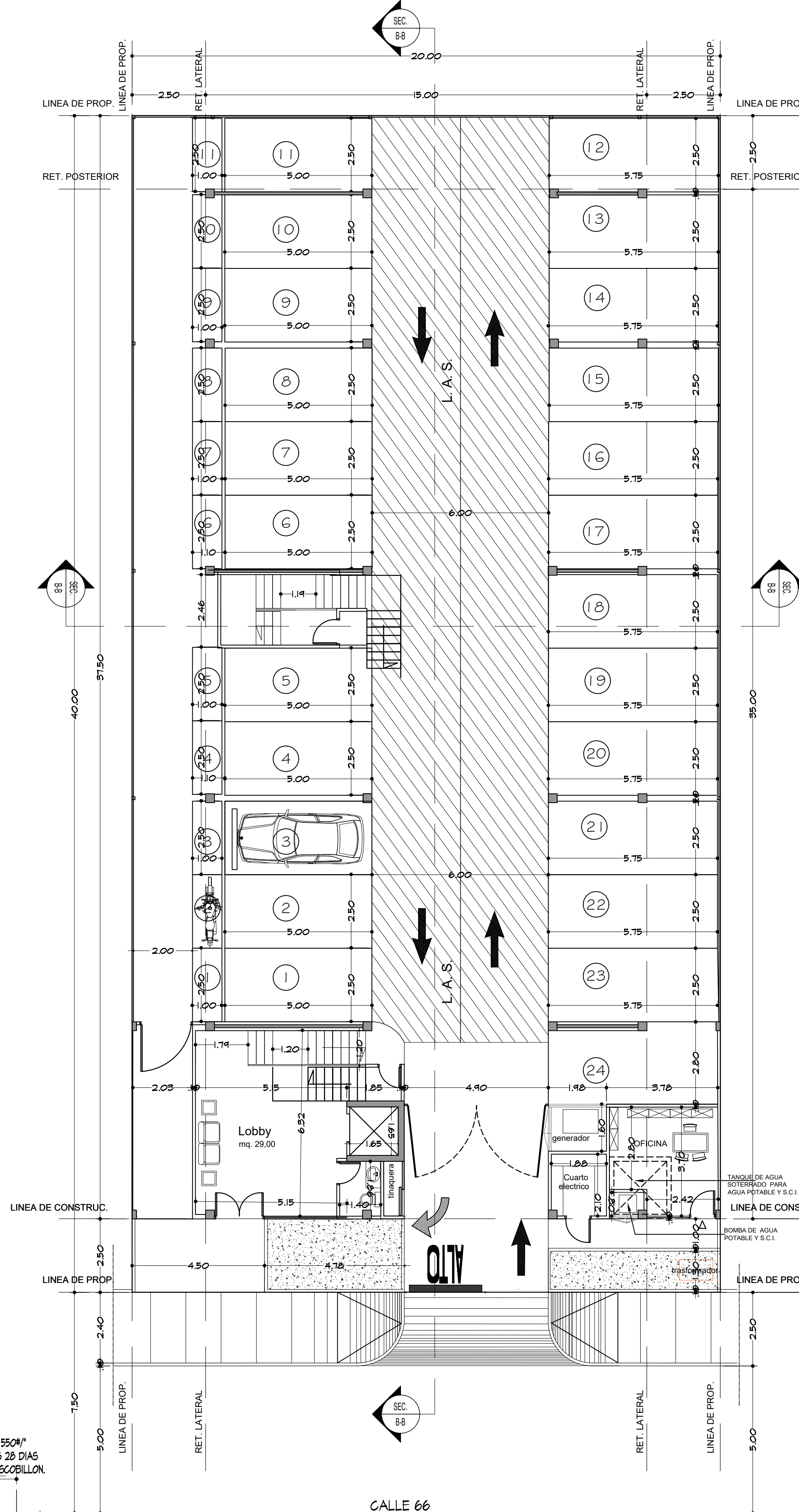
PLANTA ARQUITECTONICA NIVEL 000 ESTACIONAMIENTOS, LOBBY, RECEPCION ESC. 1:110
