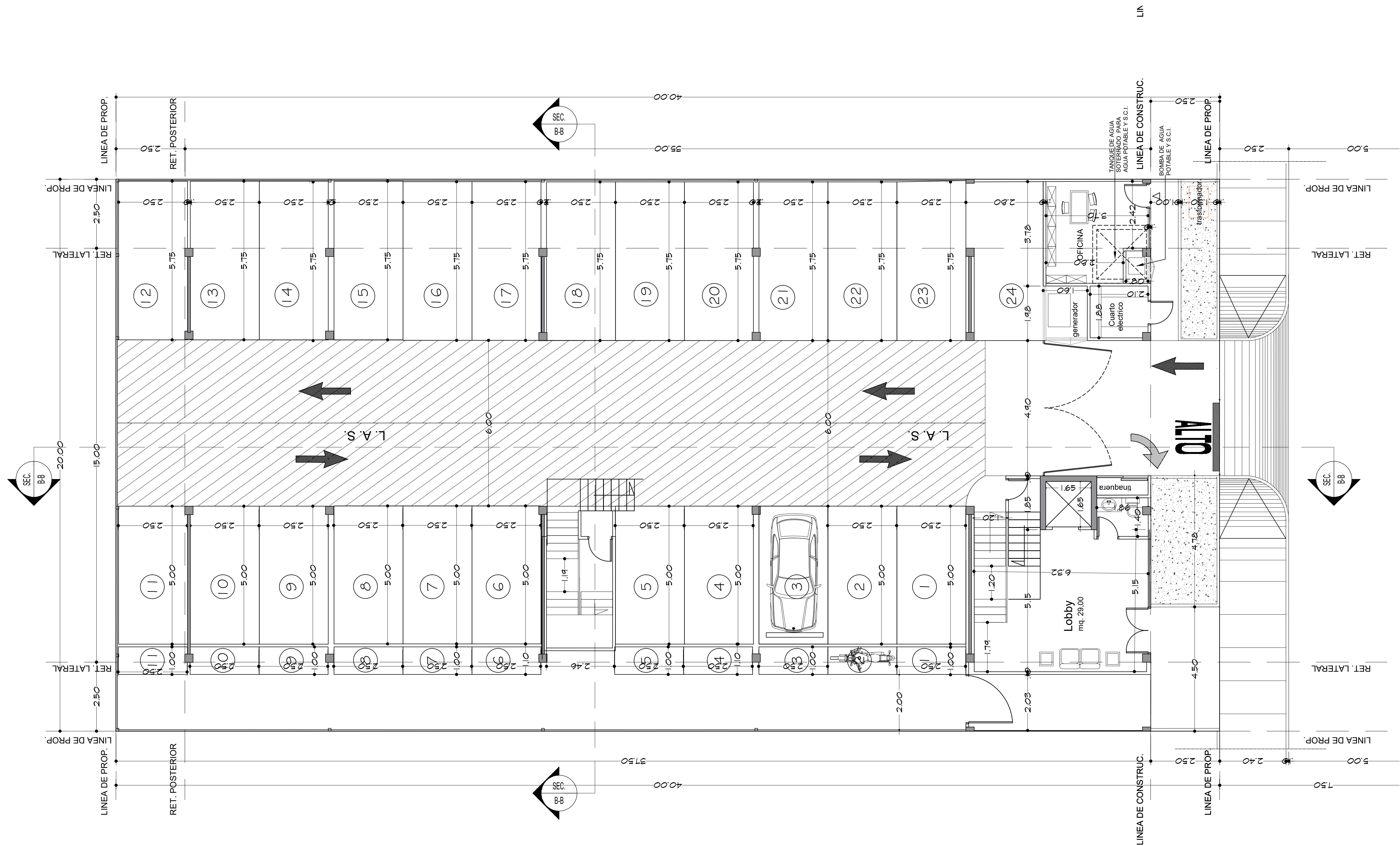
PLANTA ARQUITECTONICA NIVEL 000 ESTACIONAMIENTOS, LOBBY, RECEPCION
