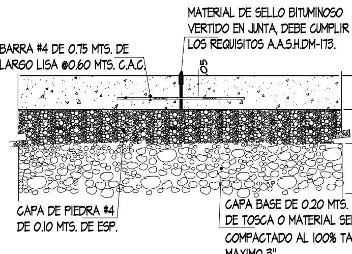
DETALLE DE EMPALME 2 DETALLE RECOMENDADOS POR EL MOP AR-1 SIN VISC.
