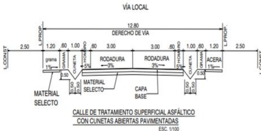
Ilustración No. 1. Secciones de vía
