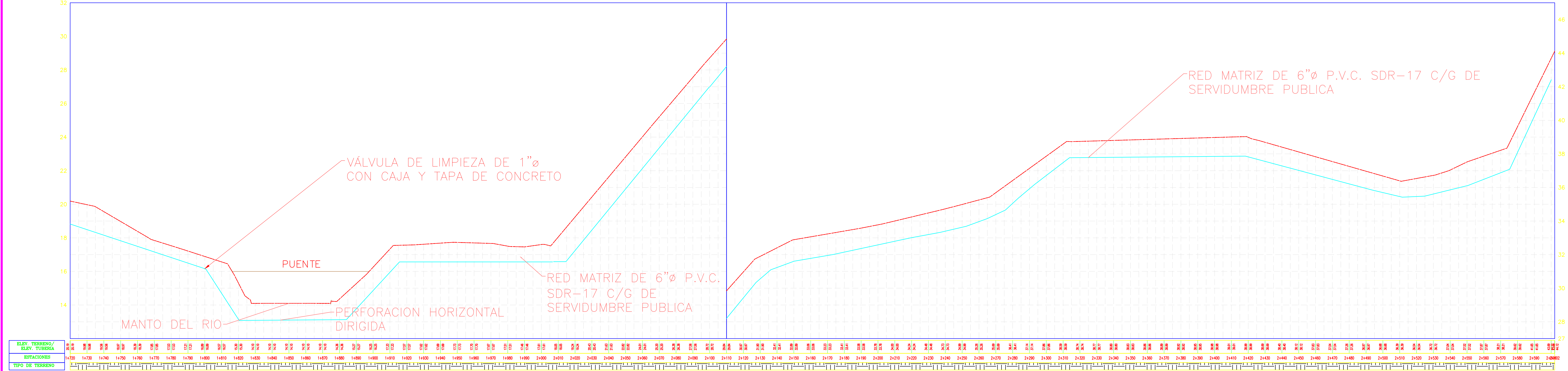
Alineación – (Perfil_Piña–Impulsion)
