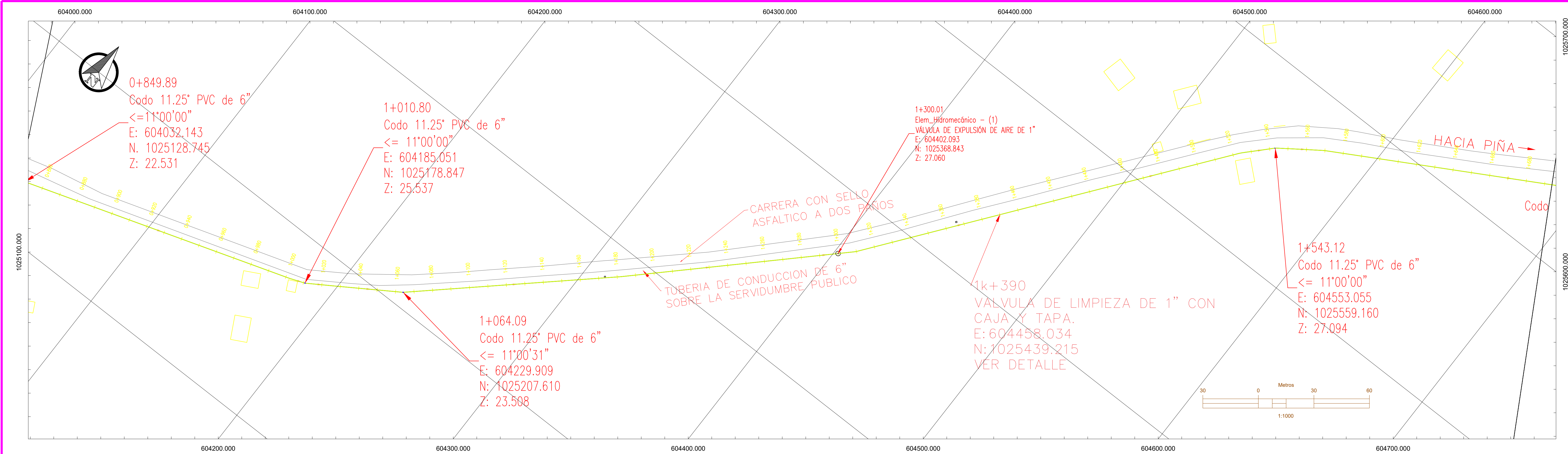
Alineación – (Perfil_Piña–Impulsion)
