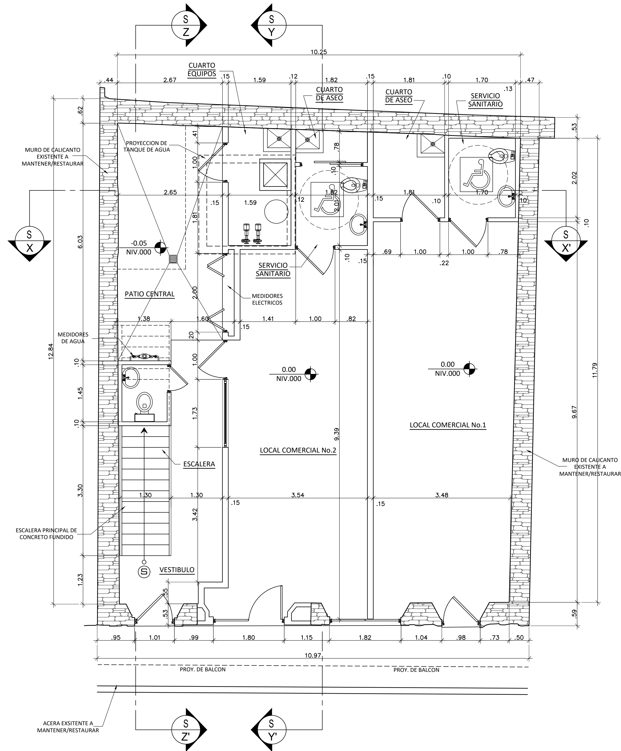
PLANTA ARQUITECTONICA NIV. 000 PROPUESTA
