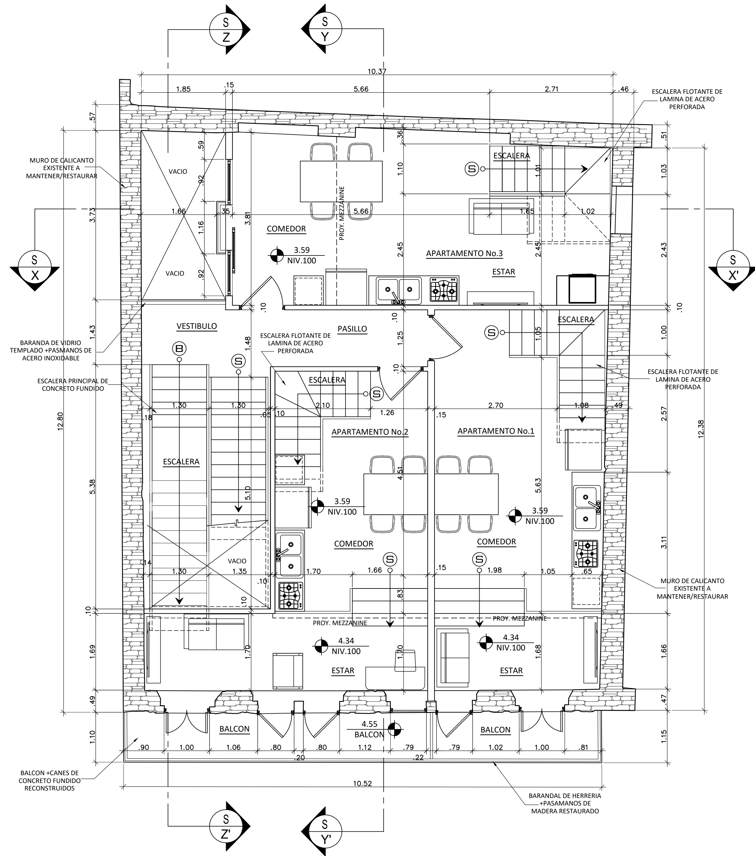
PLANTA ARQUITECTONICA NIV. 100 PROPUESTA
