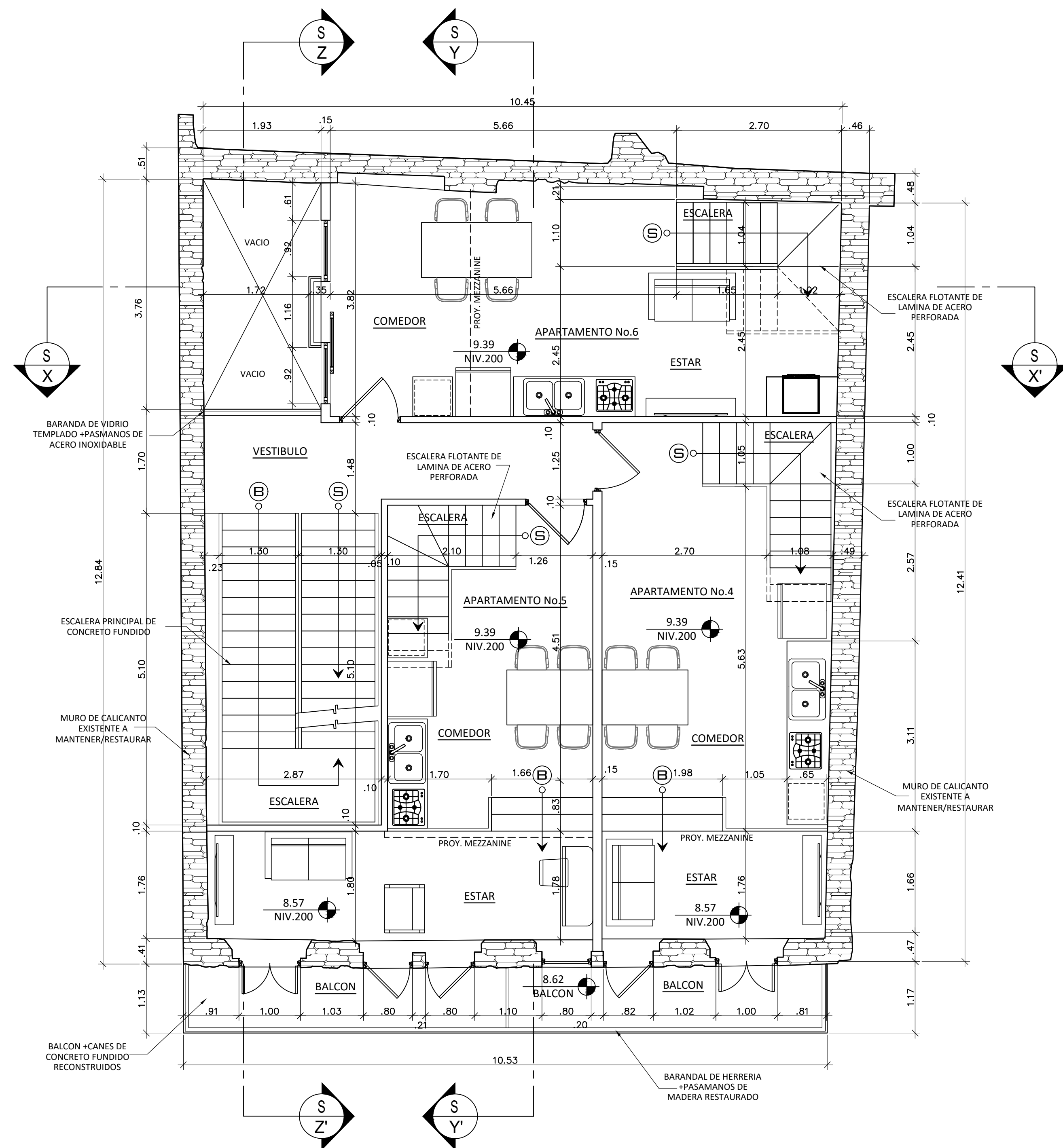
PLANTA ARQUITECTONICA NIV. 200 PROPUESTA
