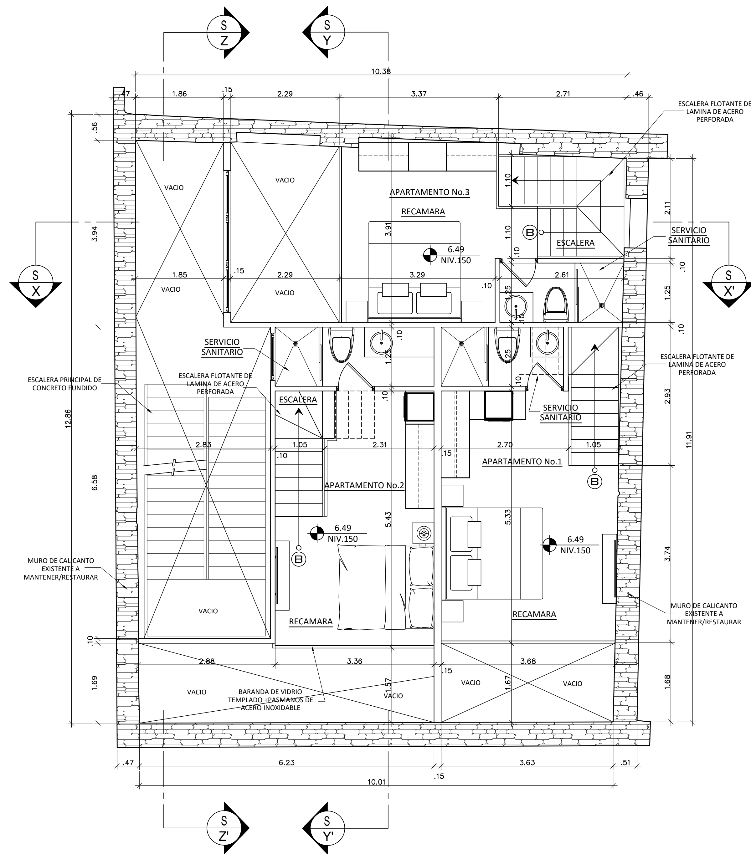
PLANTA ARQUITECTONICA NIV. 150 PROPUESTA
