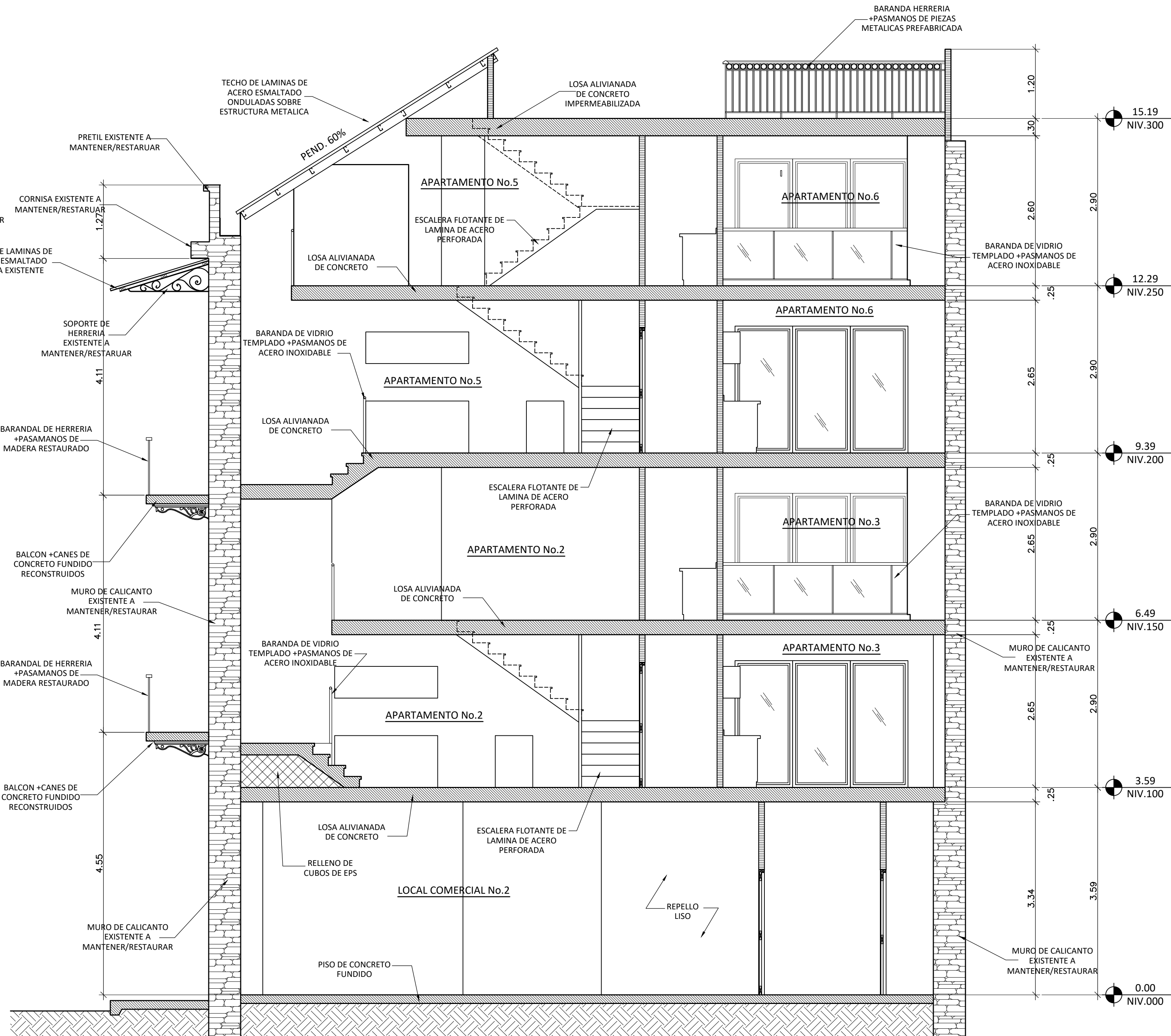
SECCION LONGITUNDINAL Y-Y' PROPUESTA ESCALA 1:50
