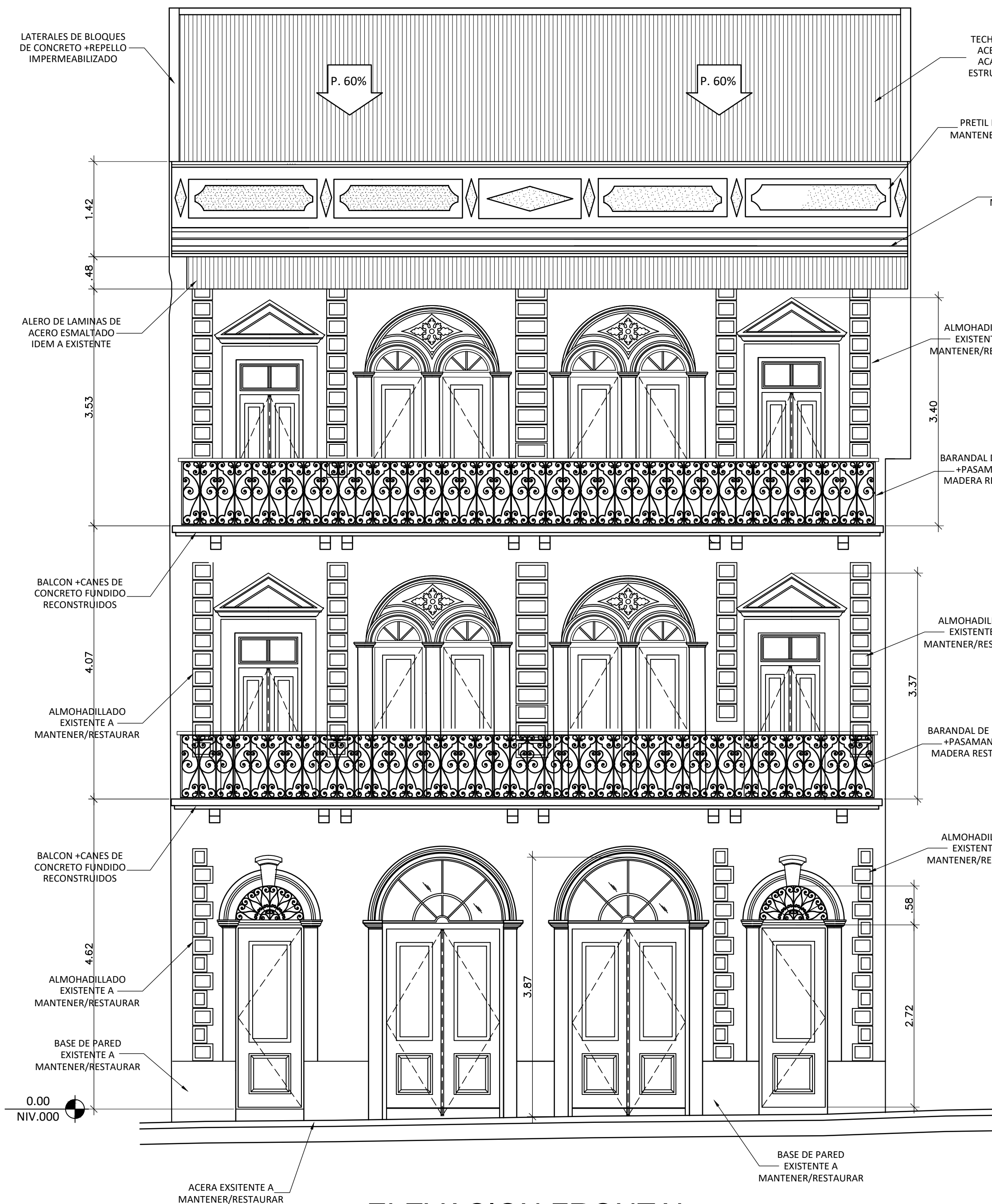
ELEVACION FRONTAL PROPUESTA ESCALA 1:50
