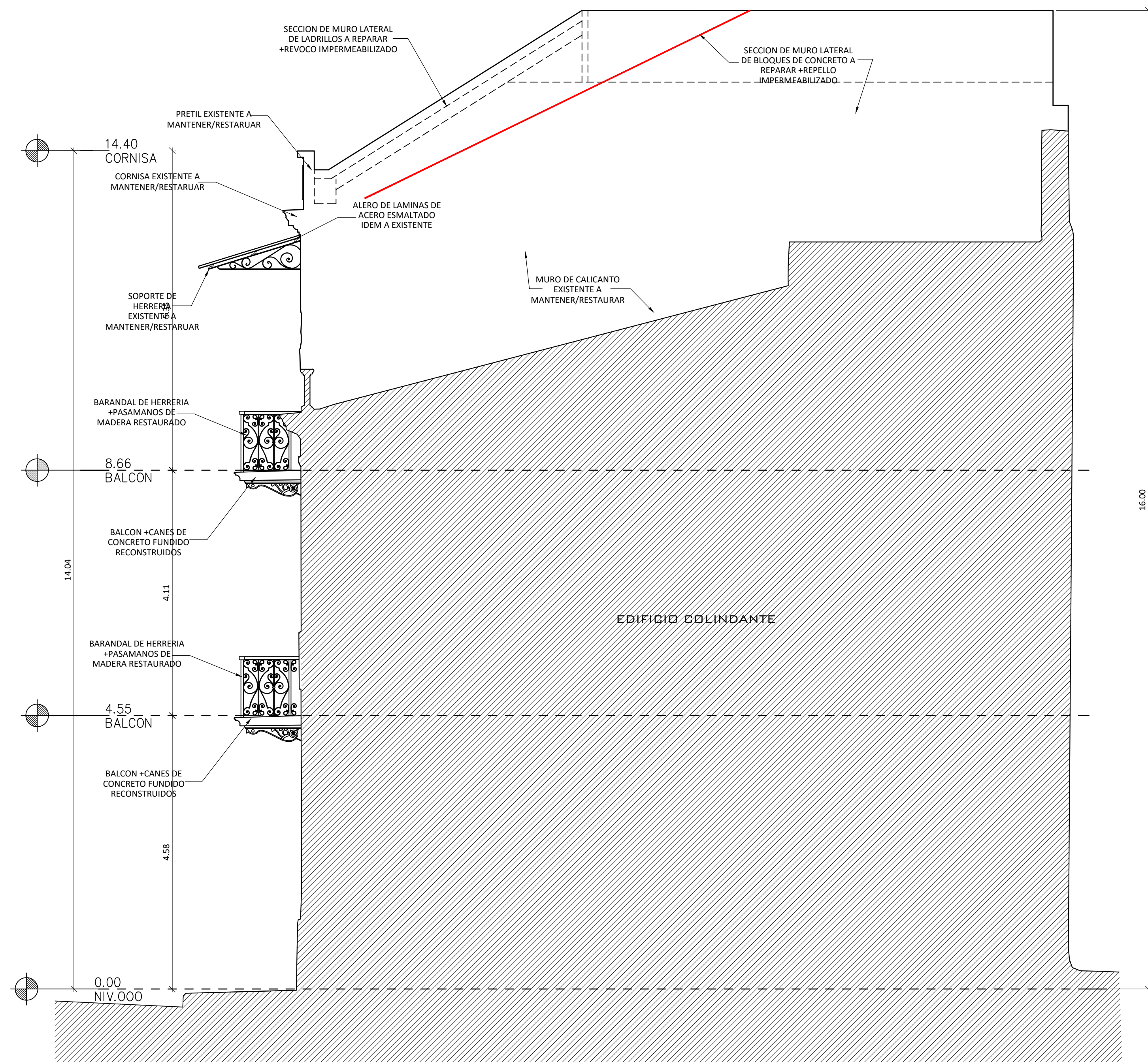
ELEVACION LATERAL DERECHA PROPUESTA
