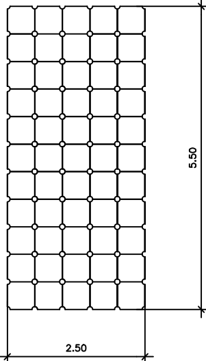
MUELLE MODULAR
