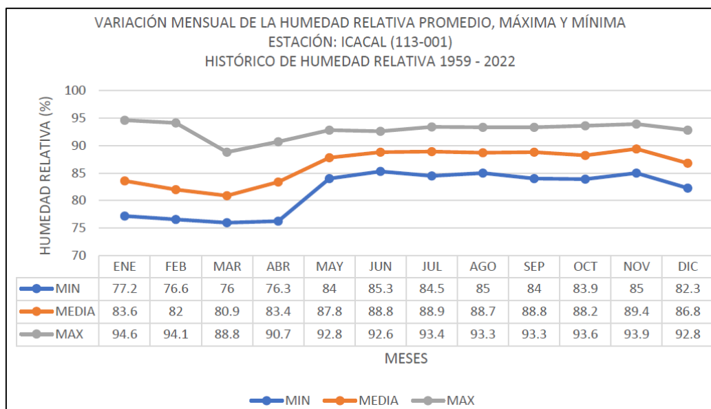
Figura No 5. Estación Icacacal N° 113-001. Humedad Relativa (%) mínima, promedio y máxima, periodo 1959-2022.
