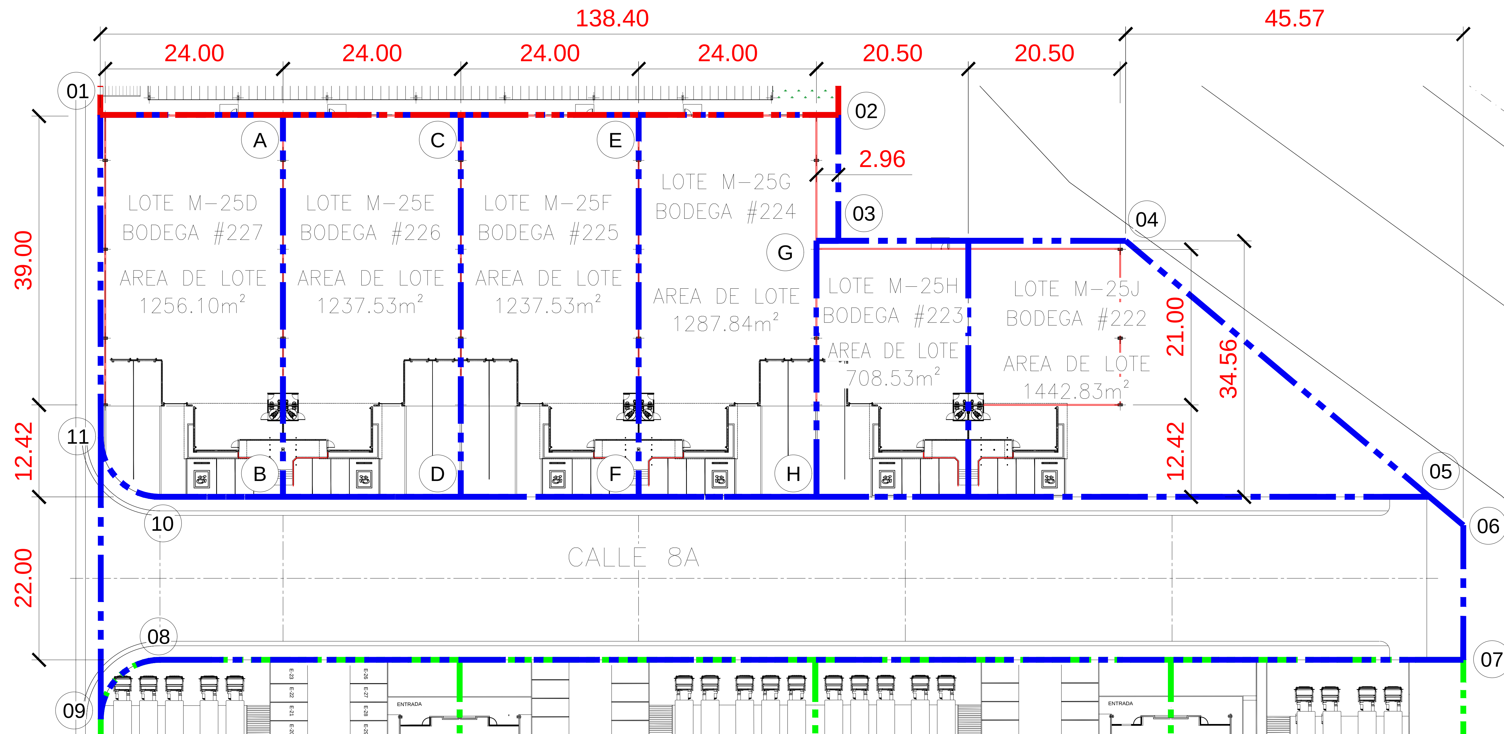
PLANTA GENERAL ESC.: S/E
