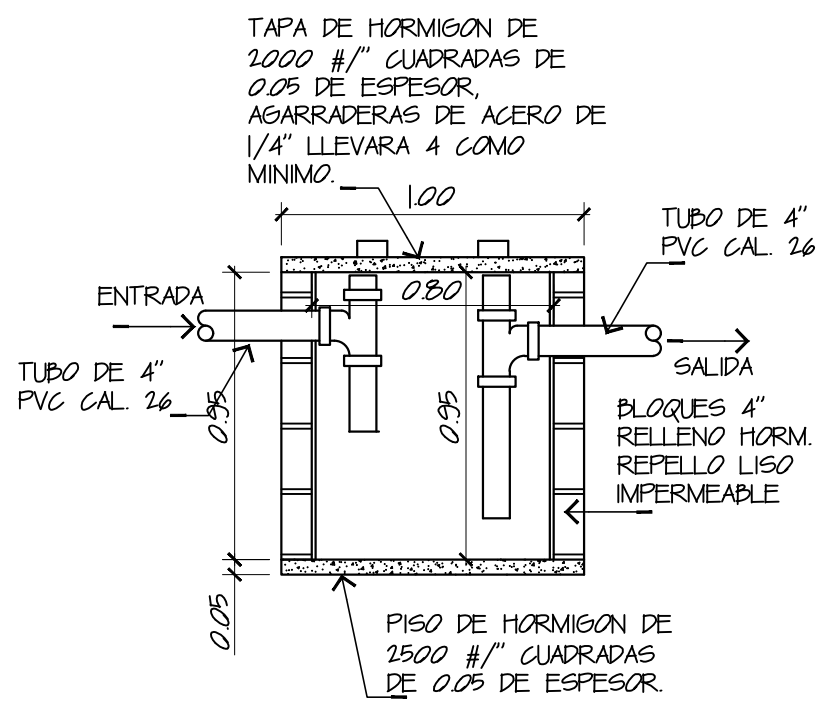
DETALLE DE GRASERA ESC.: 1/25
