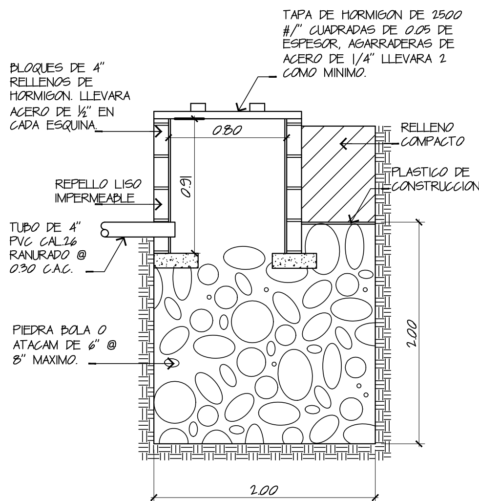
DETALLE DE POZO CIEGO ESC.: 1/25
