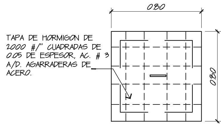
PLANTA DE CAMARA DE INSPECCION ESC.: 1/25
