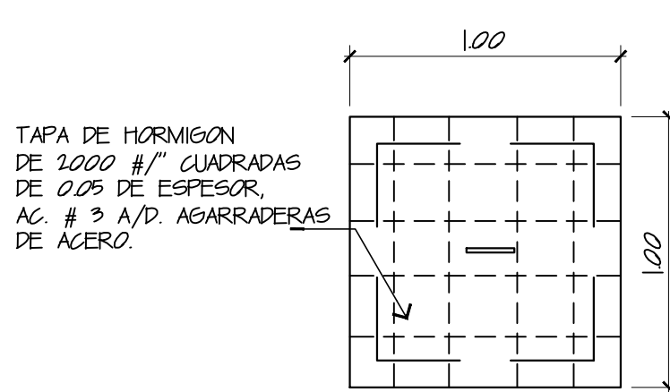
PLANTA DE GRASERA ESC.: 1/25
