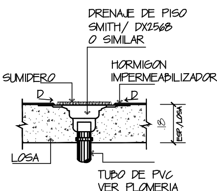
DETALLE SUMIDERO DE PISO ESC.: 1/25
