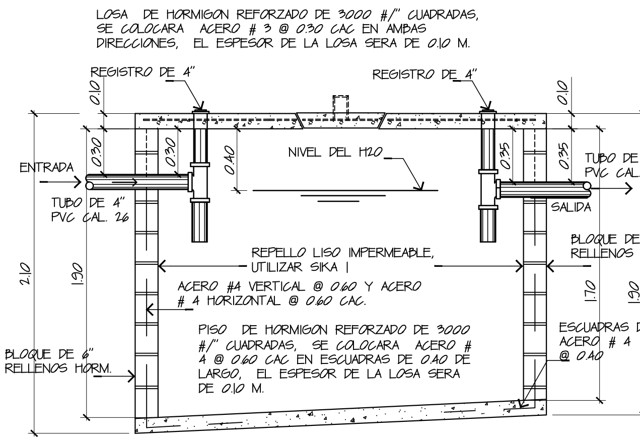
SECCION DE TANQUE SEPTICO ESC.: 1/25
