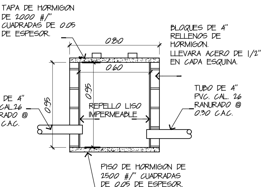
CAMARA DE INSPECCION ESC.: 1/25
