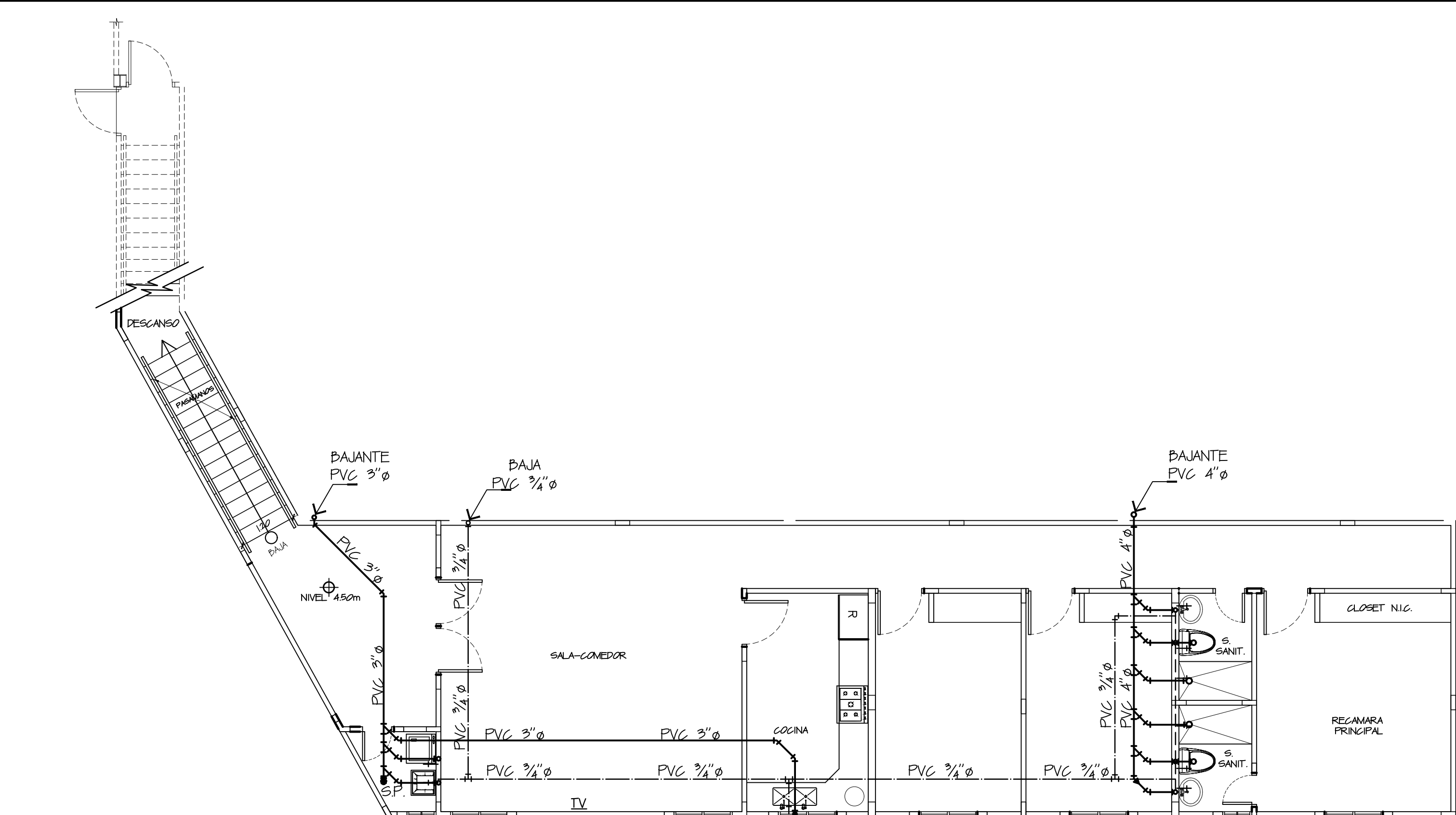
PLOMERIA PLANTA ALTA DE RESIDENCIA ESC.: 1/75
