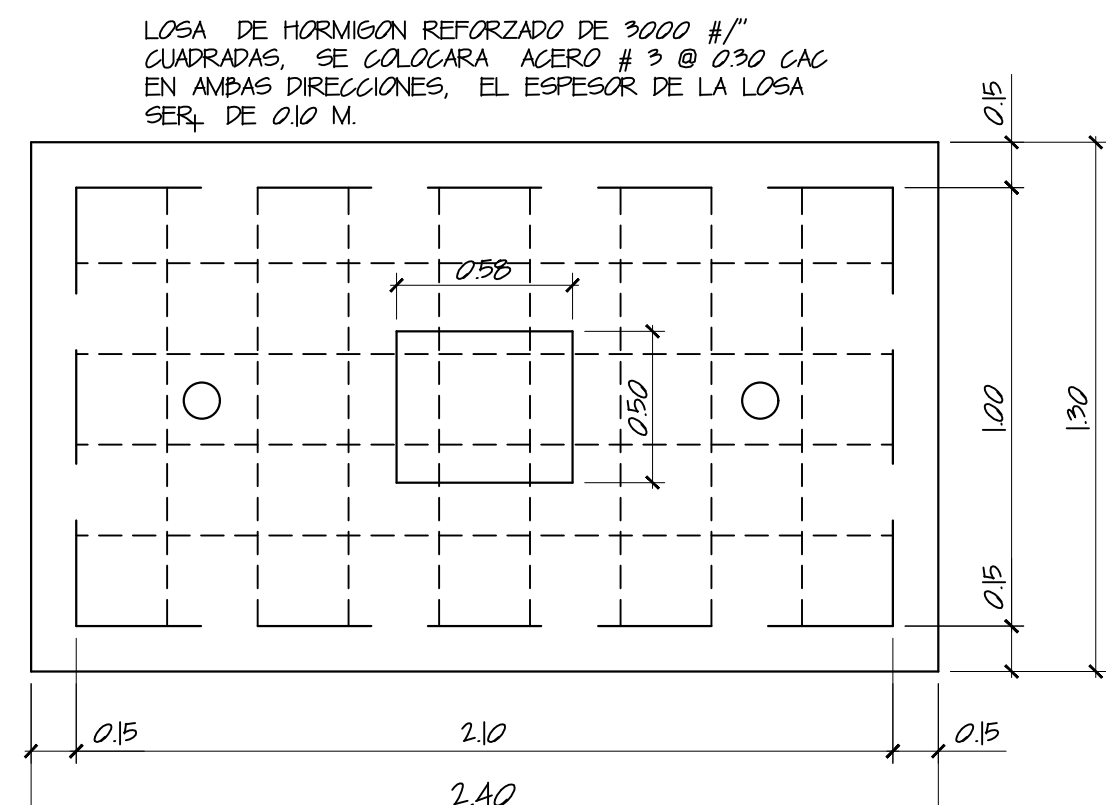
PLANTA DE TANQUE SEPTICO ESC.: 1/25
