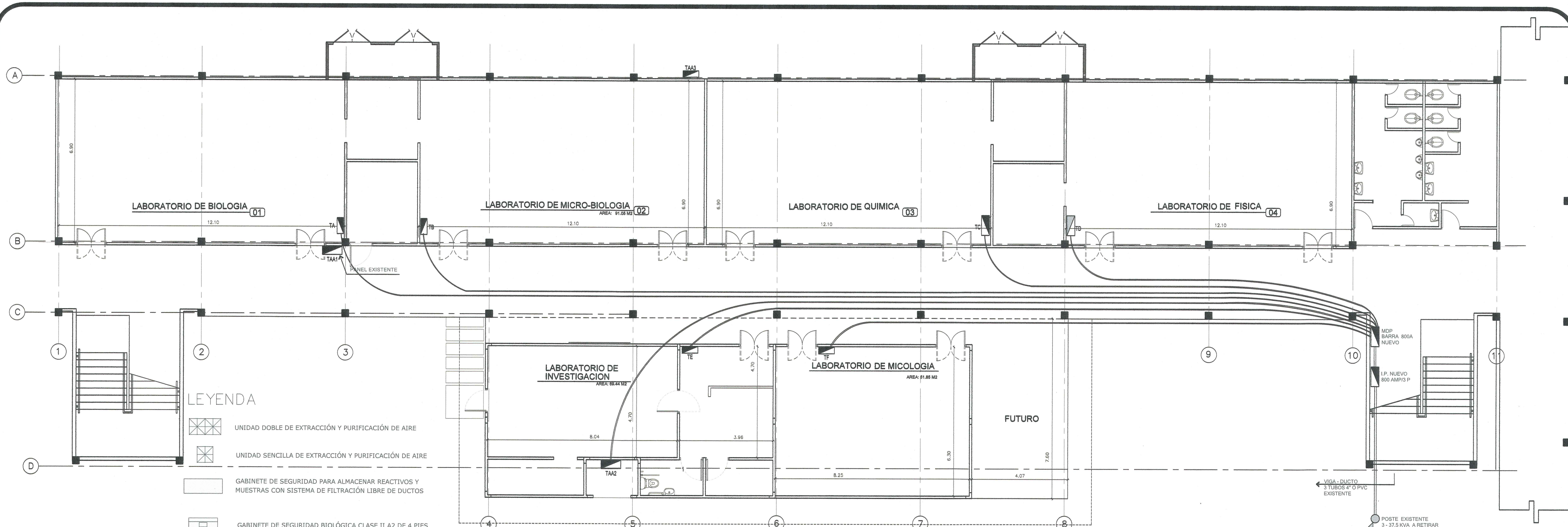
PLANTA RECORRIDO DE MDP A TABLEROS ELECTRICO ESC. 1:75
