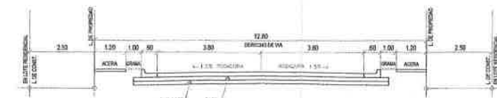
SECCION TIPICA DE VIAS LOCALES (12.80 M)
