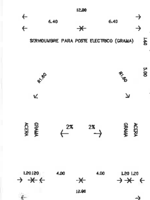
DETALLE DE MARTILLO - 12.80 mts S / ESC.
