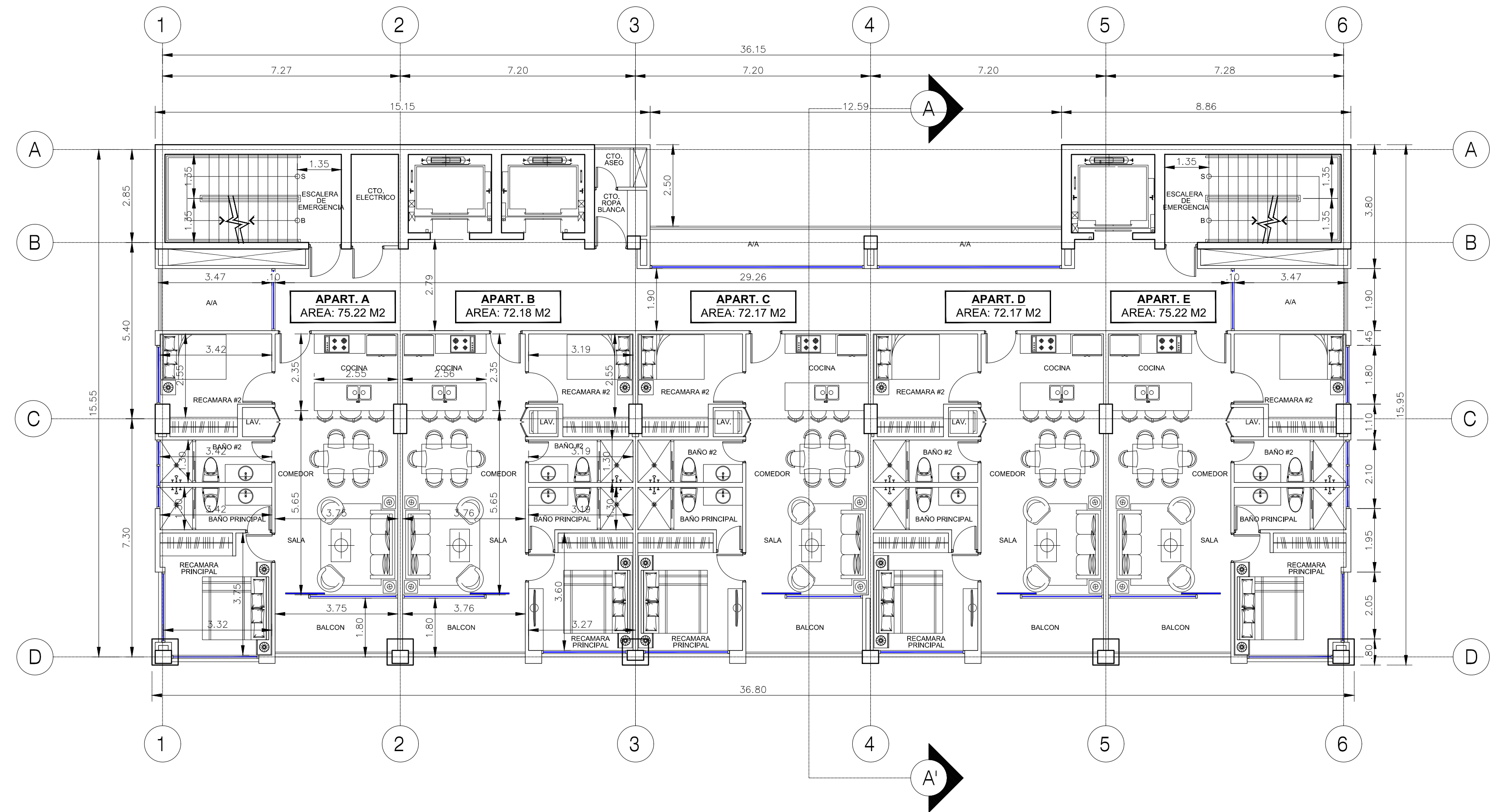
PLANTA ARQUITECTONICA NIVEL 100 @ 1300 ESCALA: 1:100
