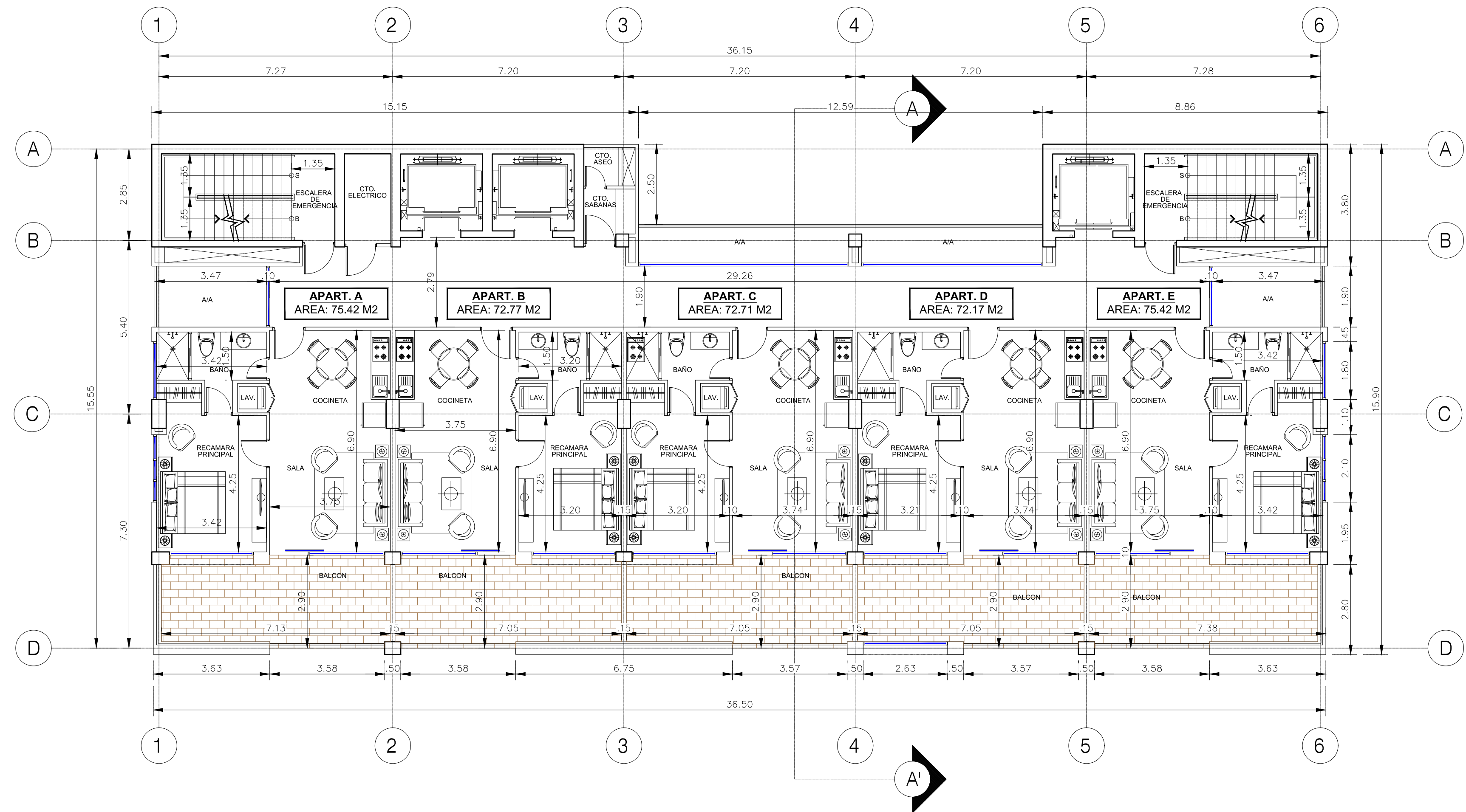
PLANTA ARQUITECTONICA NIVEL 1400 ESCALA: 1:100
