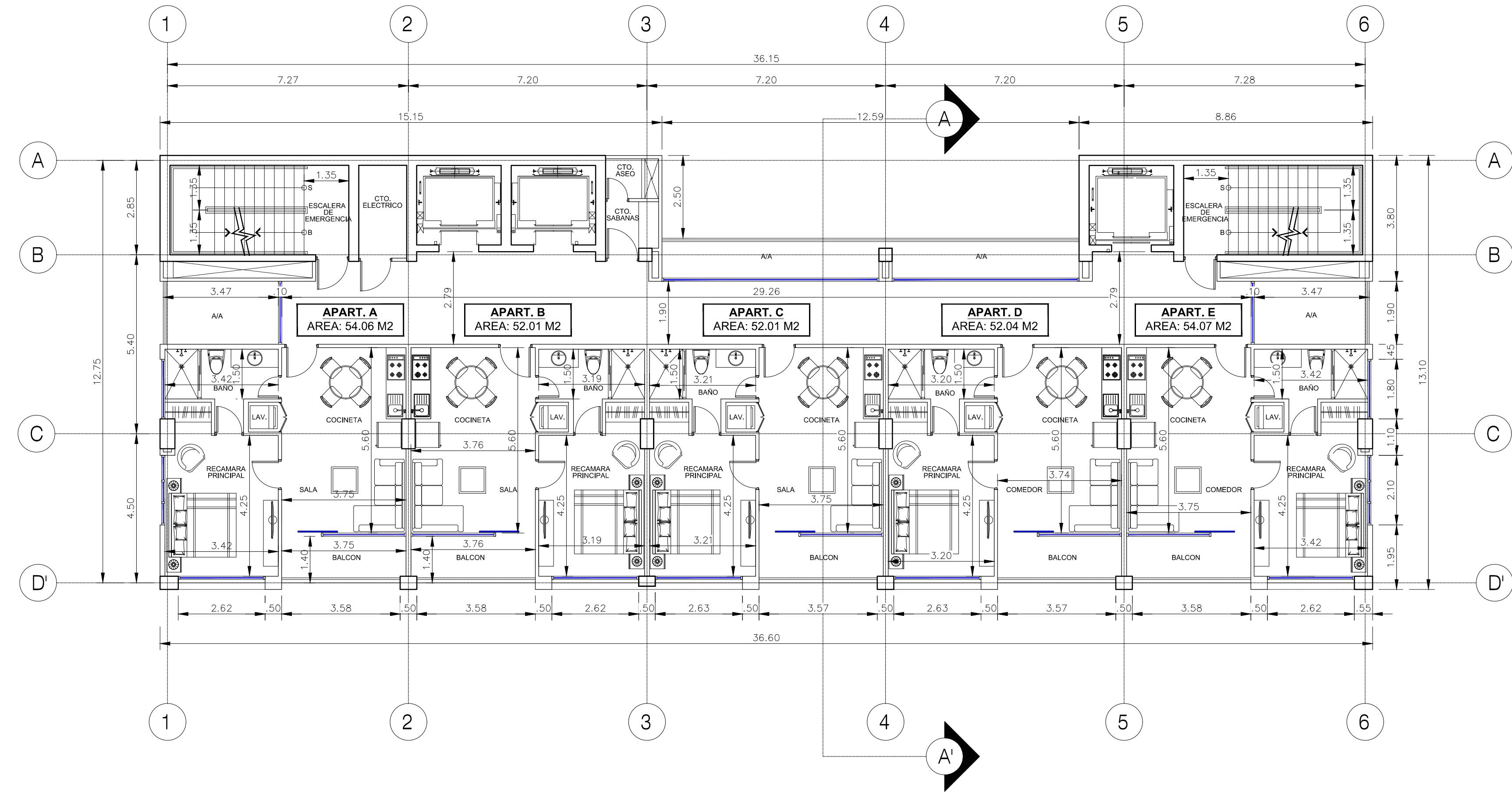
PLANTA ARQUITECTONICA NIVEL 1500 @ 2600 ESCALA: 1:100
