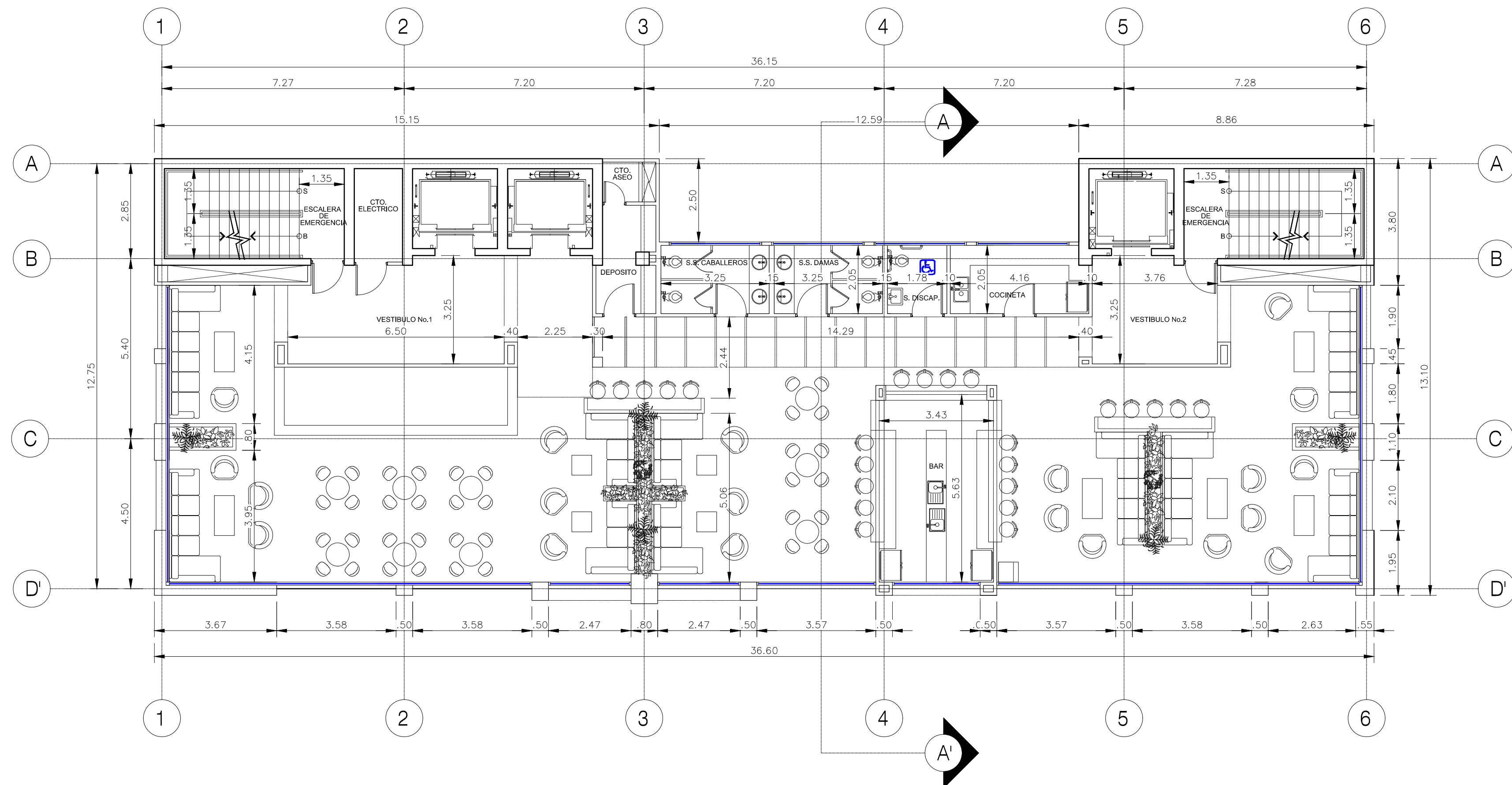
PLANTA ARQUITECTONICA NIVEL 2700 - ROOF TOP ESCALA: 1:100
