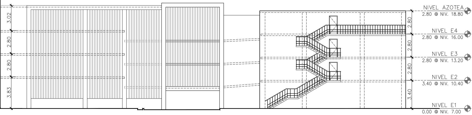
ELEVACION LAT. IZQUIERDA
