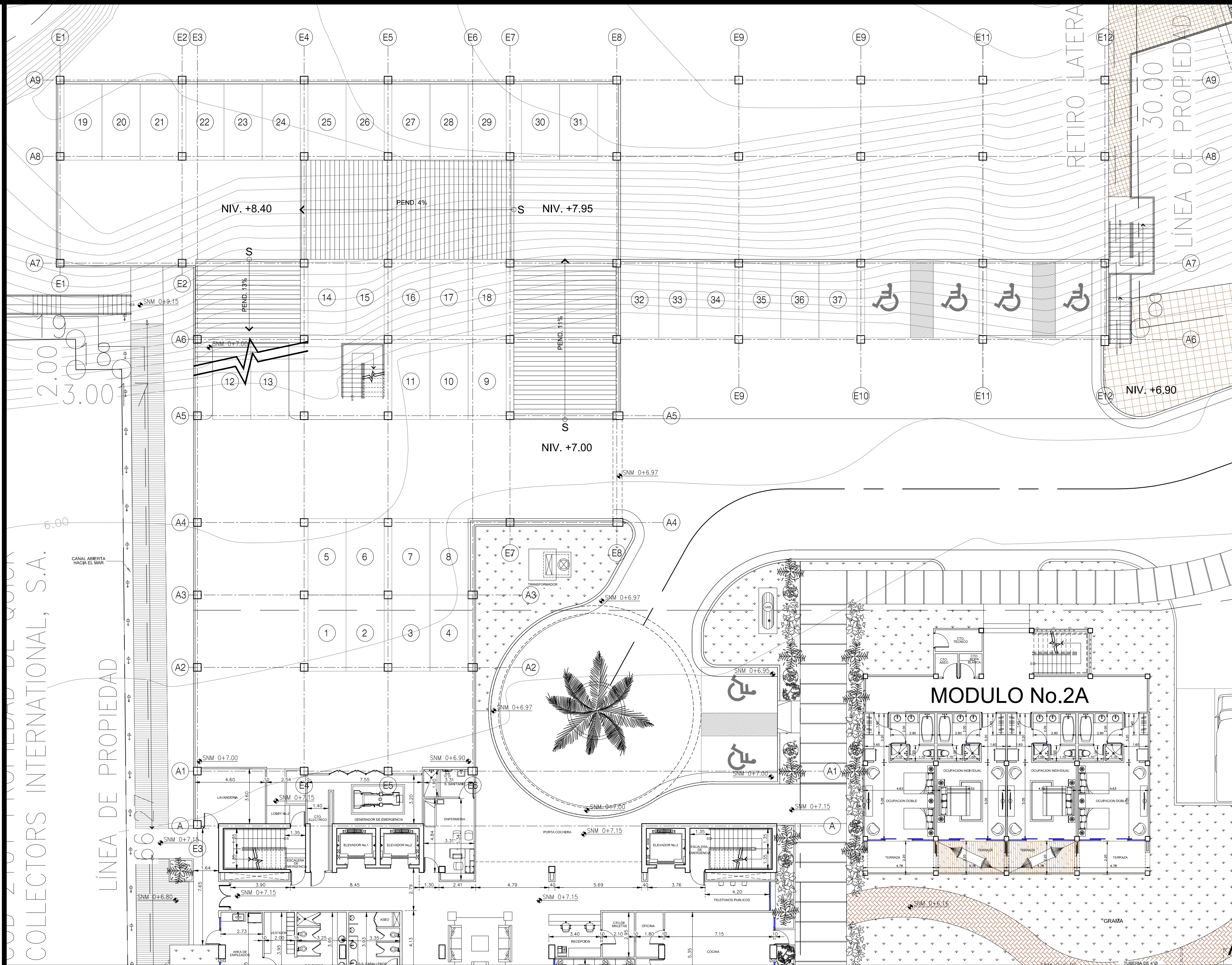
PLANTA ARQUITECTONICA - EDIF. DE ESTACIONAMIENTOS - NIVEL E1
