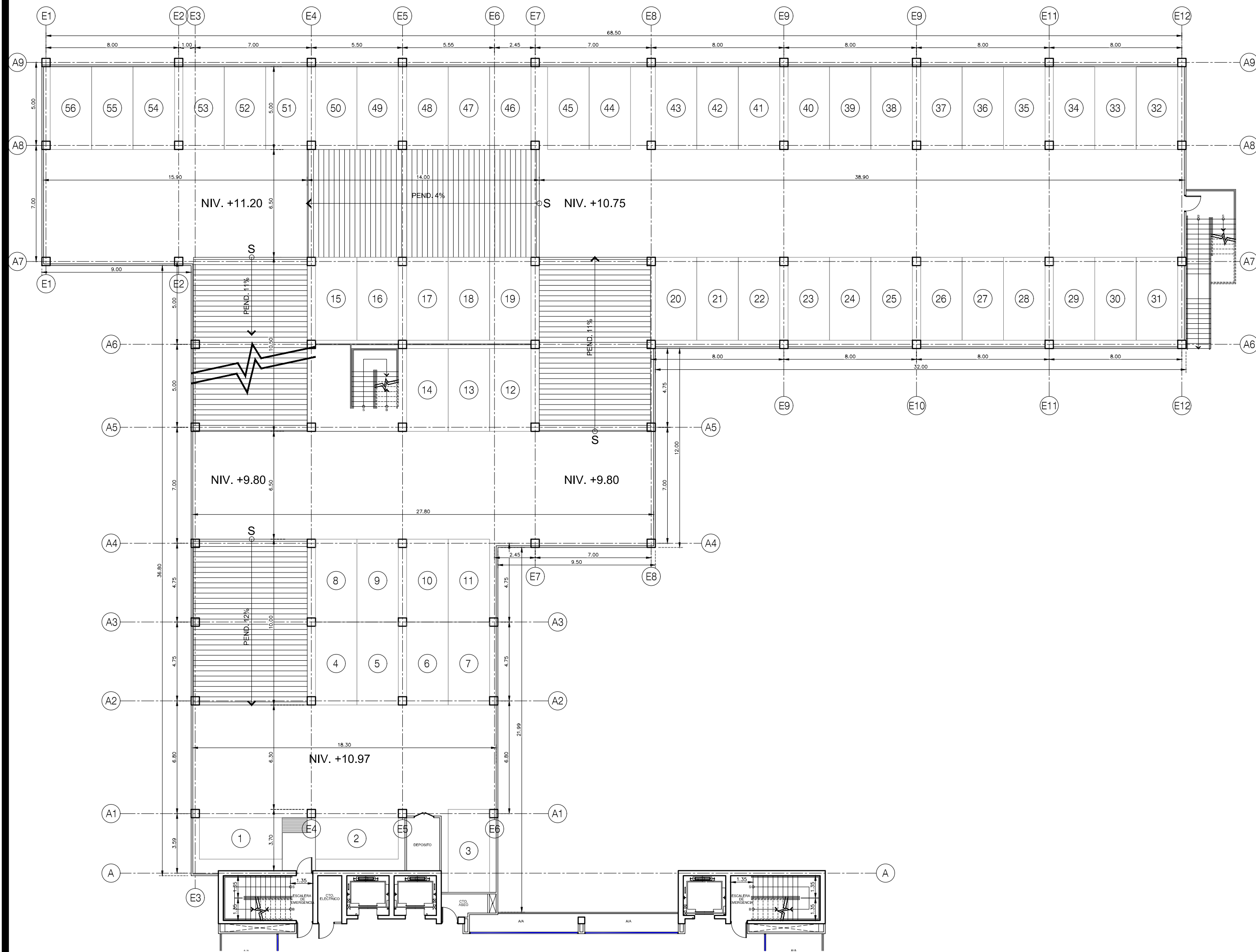
PLANTA ARQUITECTONICA - EDIF. ESTACIONAMIENTOS - NIVEL E2 ESCALA: 1:200
