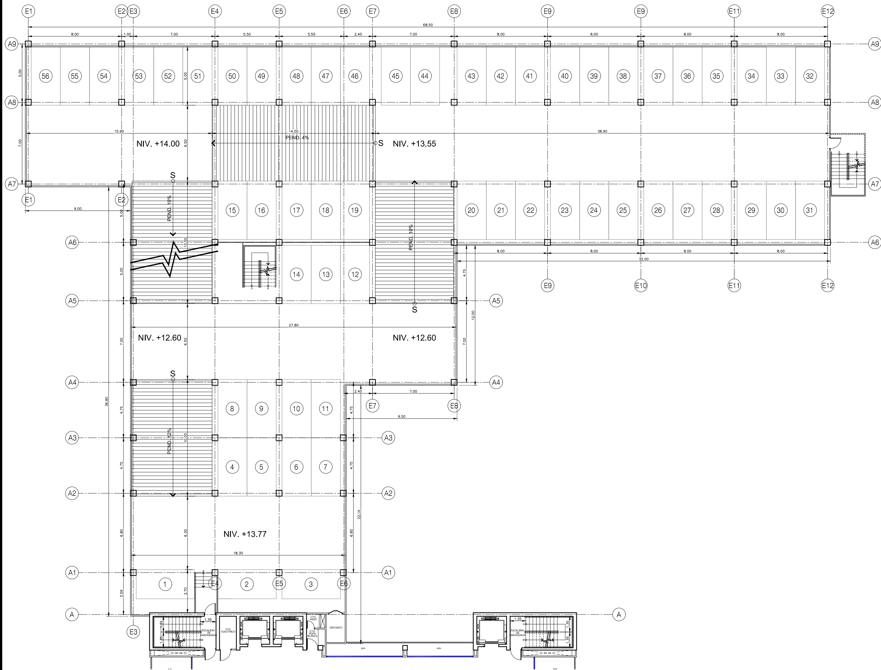
PLANTA ARQUITECTONICA - EDIF. ESTACIONAMIENTOS - NIVEL E3 ESCALA: 1:200
