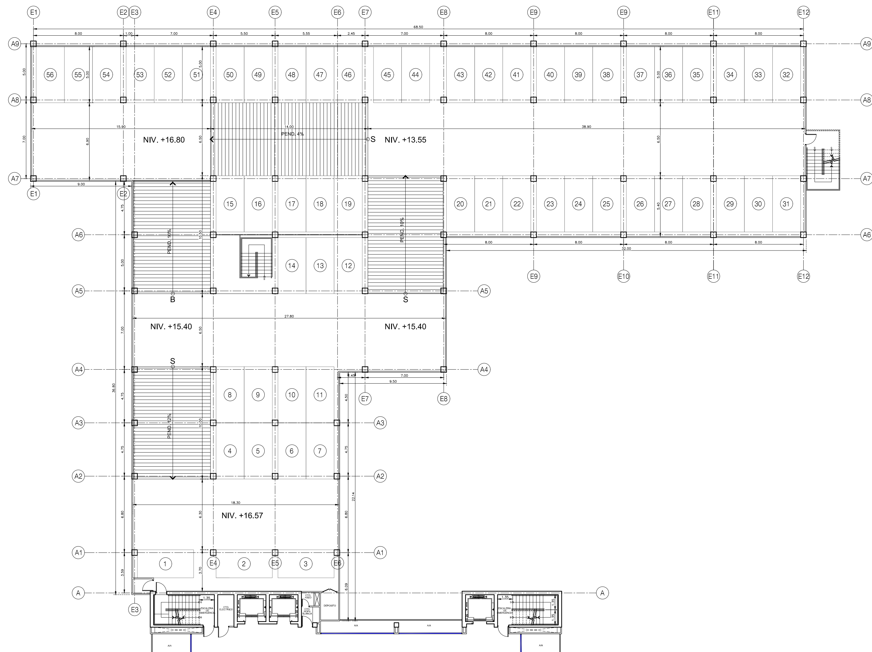
PLANTA ARQUITECTONICA - EDIF. ESTACIONAMIENTOS - NIVEL E4
