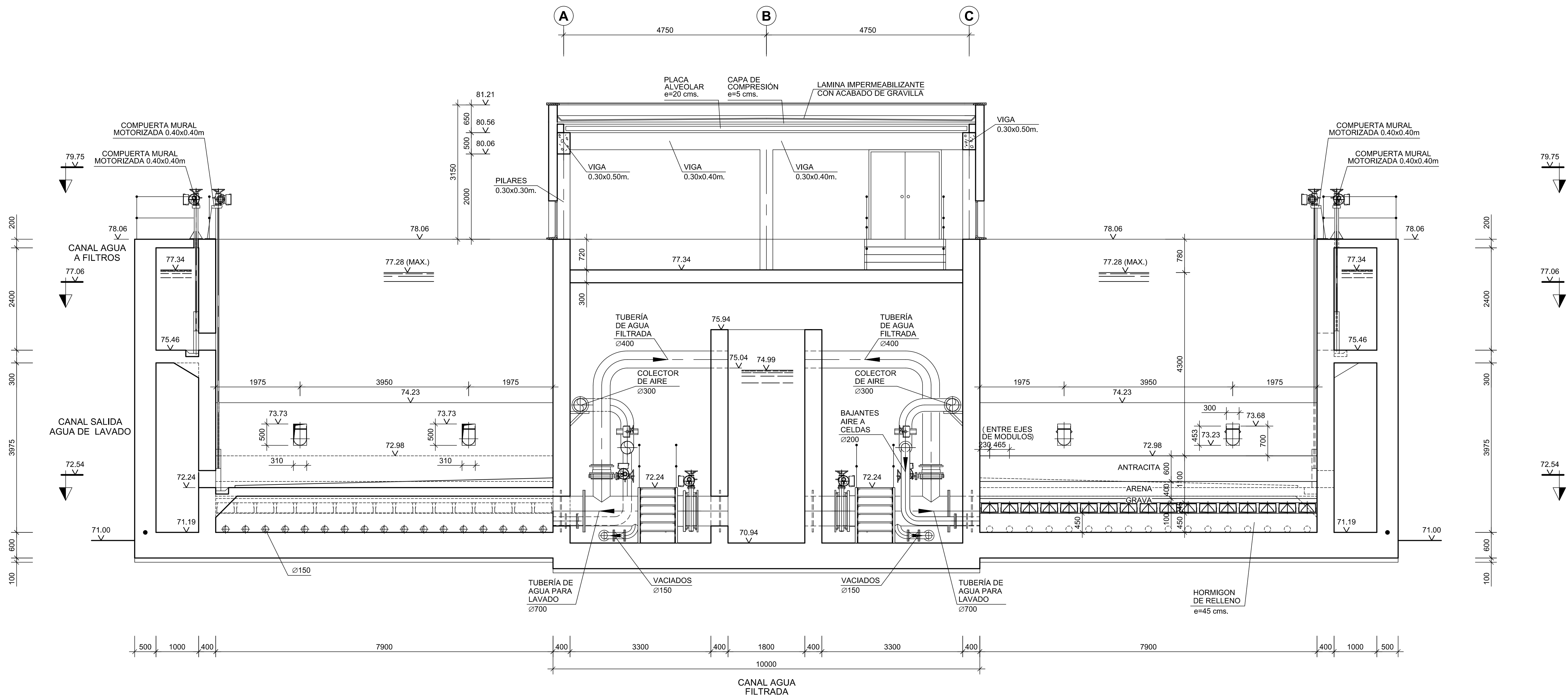
SECCIÓN E-E ESCALA 1:100
