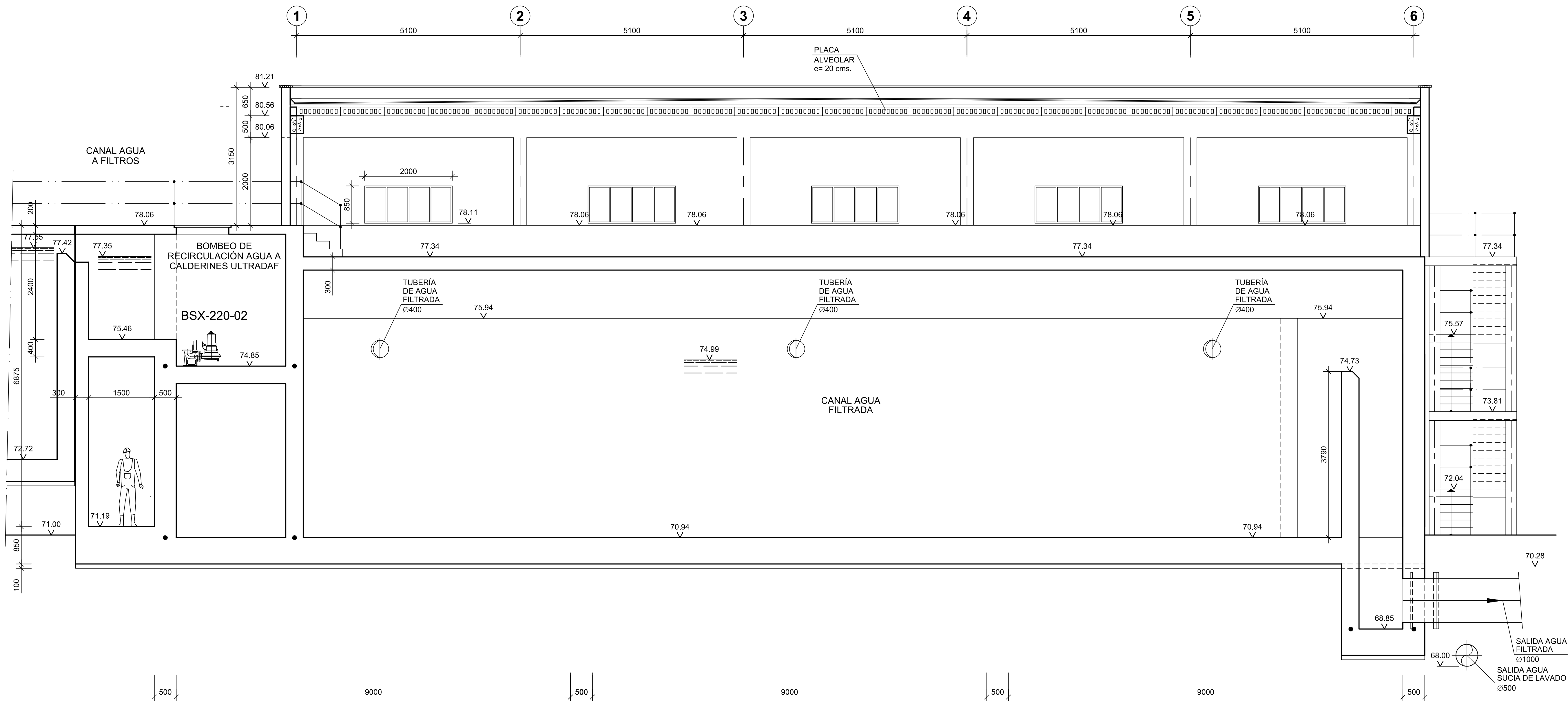
SECCIÓN C-C ESCALA 1:100
