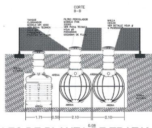
DETALLES DE PLANTA DE TRATAMIENTO EXISTENTE ESCALA: S/E
