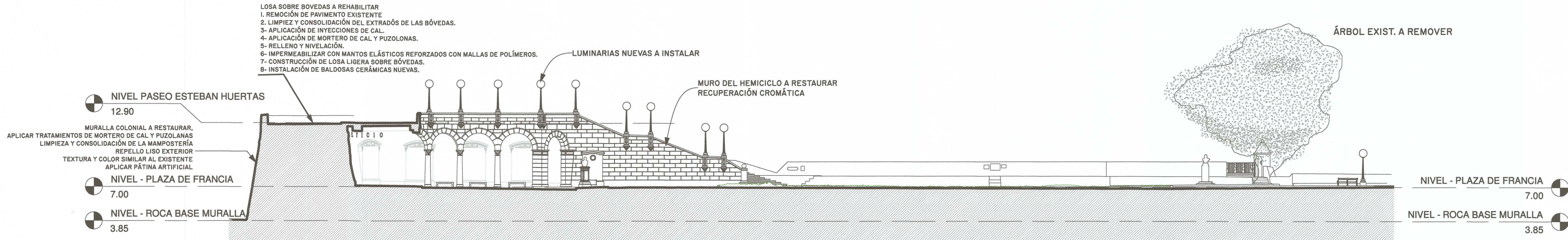
1 SECCION LONGITUDINAL SUR - NORTE 1 : 200
