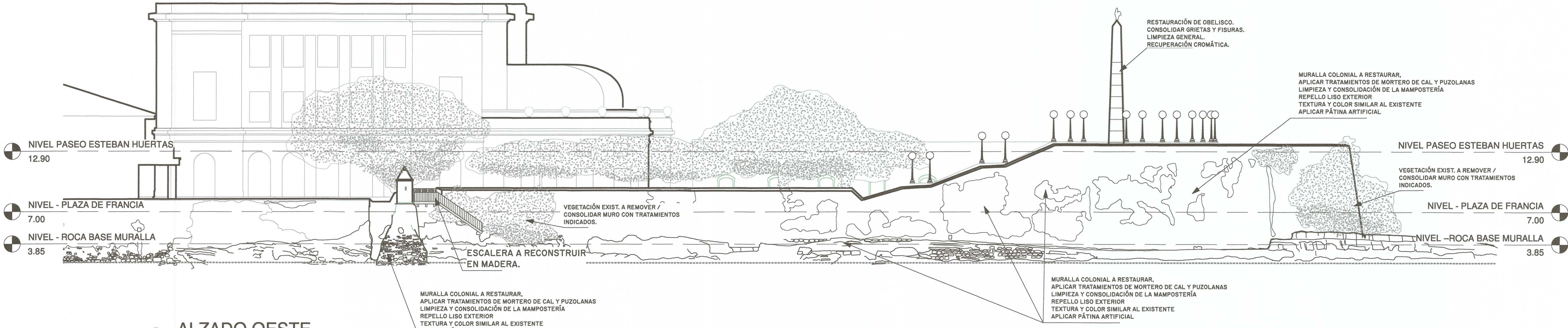
2 ALZADO OESTE 1 : 200
