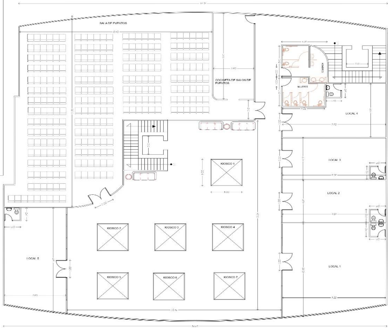
PLANTA ARQUITECTÓNICA SEGUNDO NIVEL ESC. 1:100
