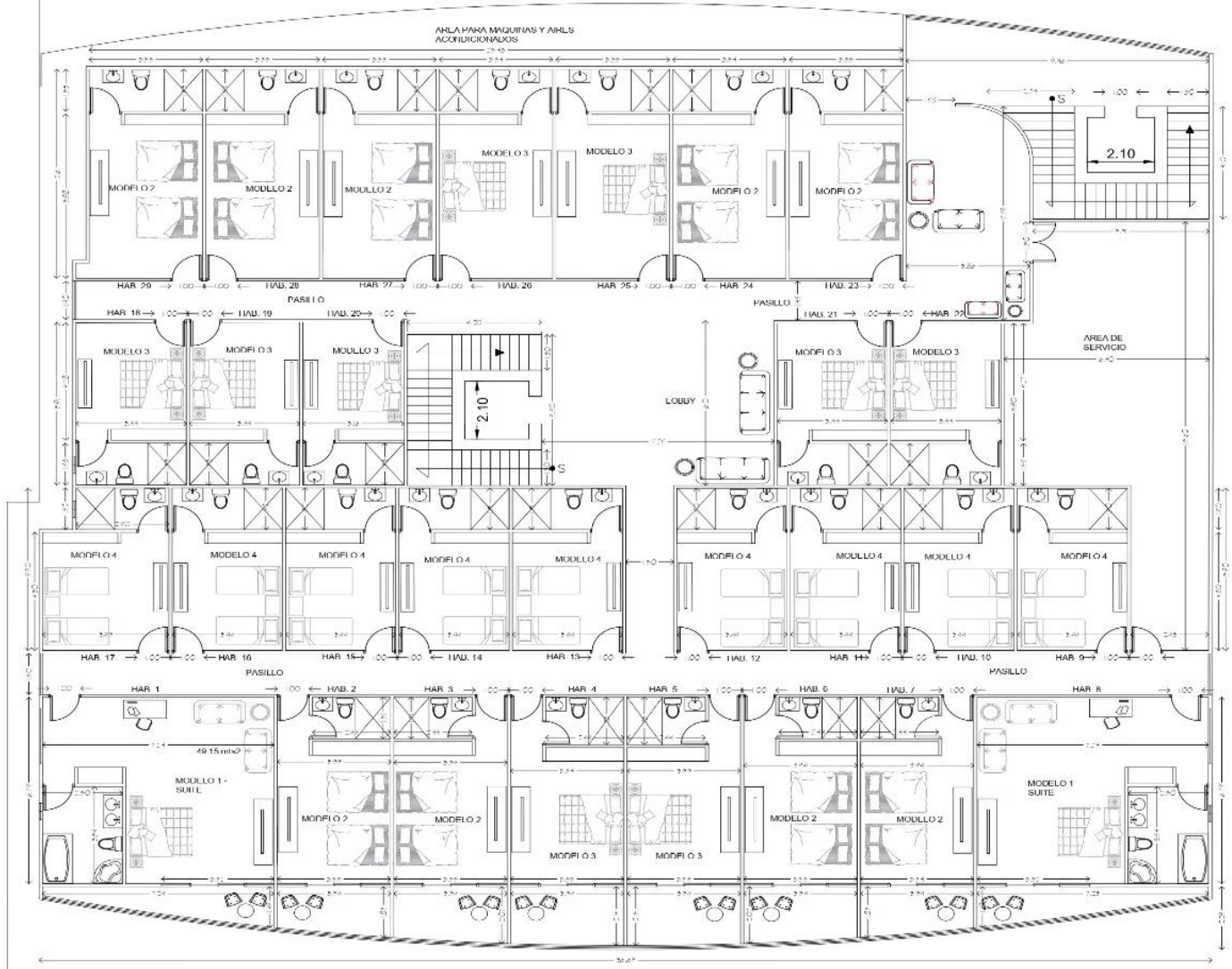
PLANTA ARQUITECTÓNICA TERCER NIVEL ESC. 1:100
