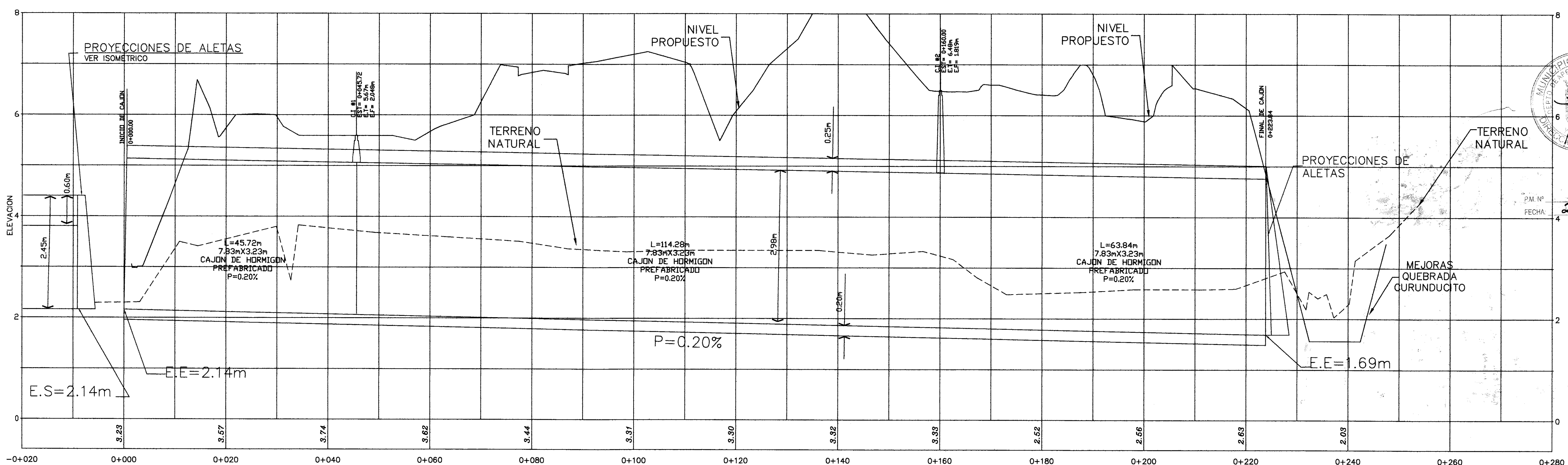
Secciones de Mejoras a la Quebrada Curunducito Esc: 1:1000
