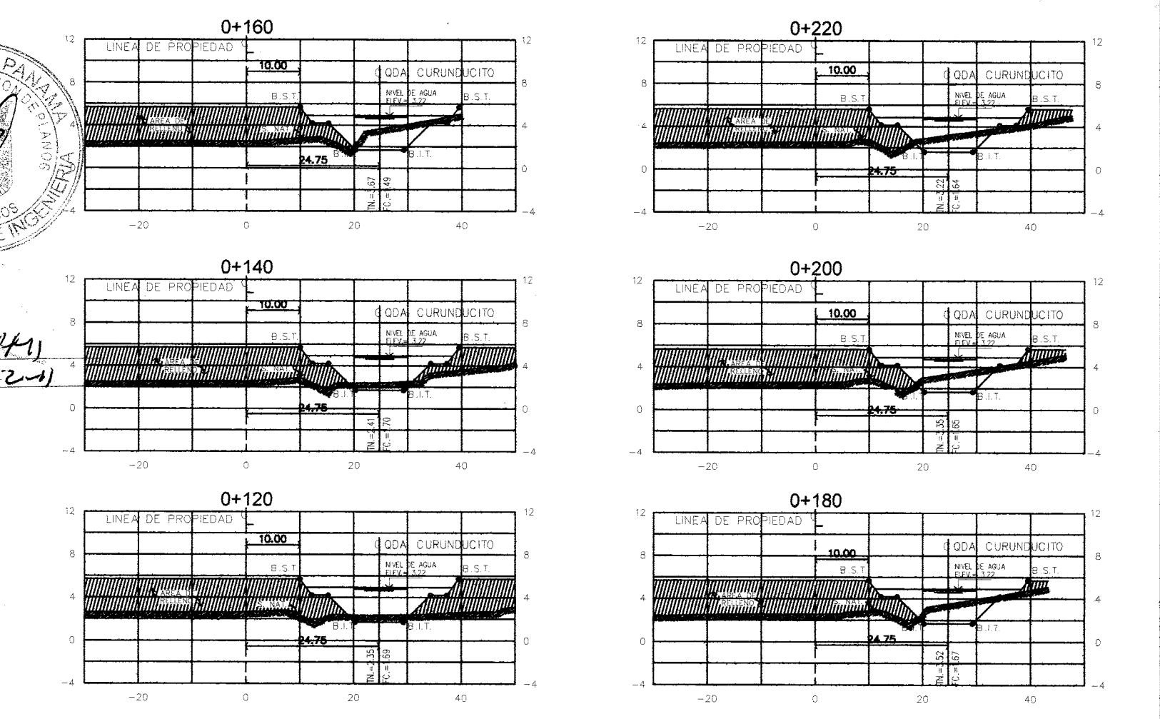
Secciones de Mejoras a la Quebrada Curunducito Esc: 1:1000
