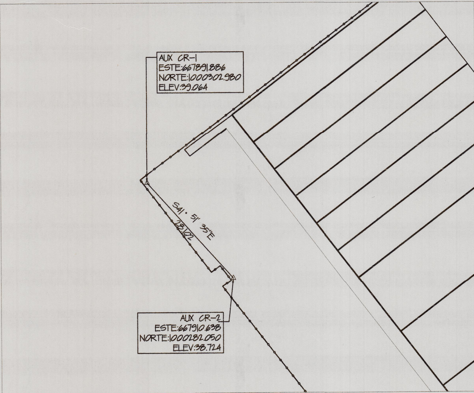
DETALLE DE AMARRE ESCALA: 1:500
