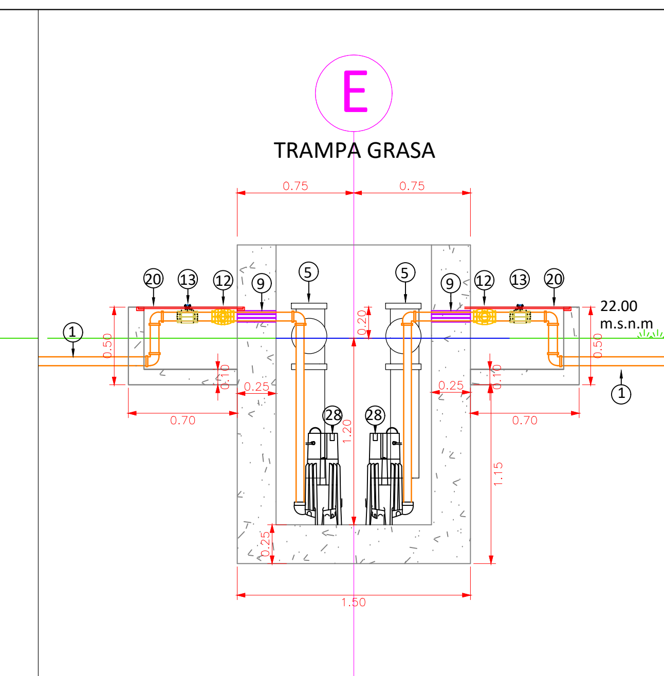
VISTA DE CORTE iii Esc. 1:25
