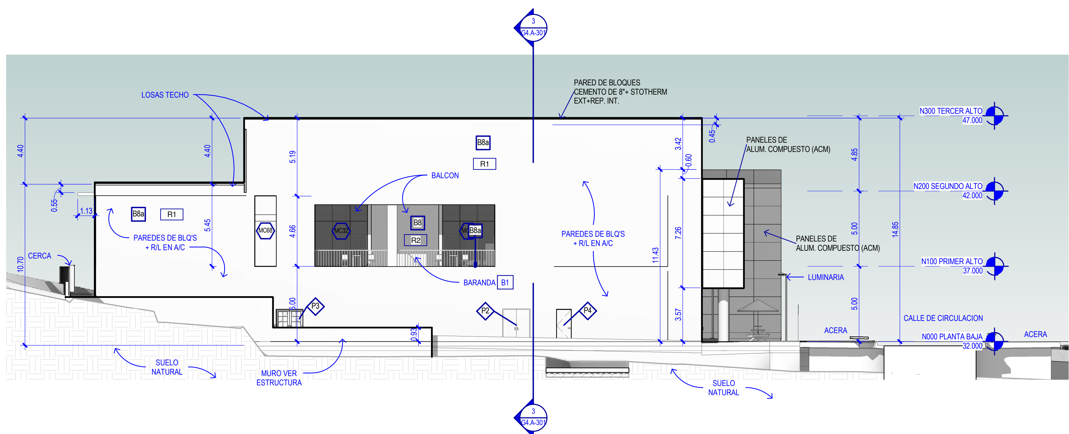
2 ELEVACION EXTERIOR - ESTE 1:150
