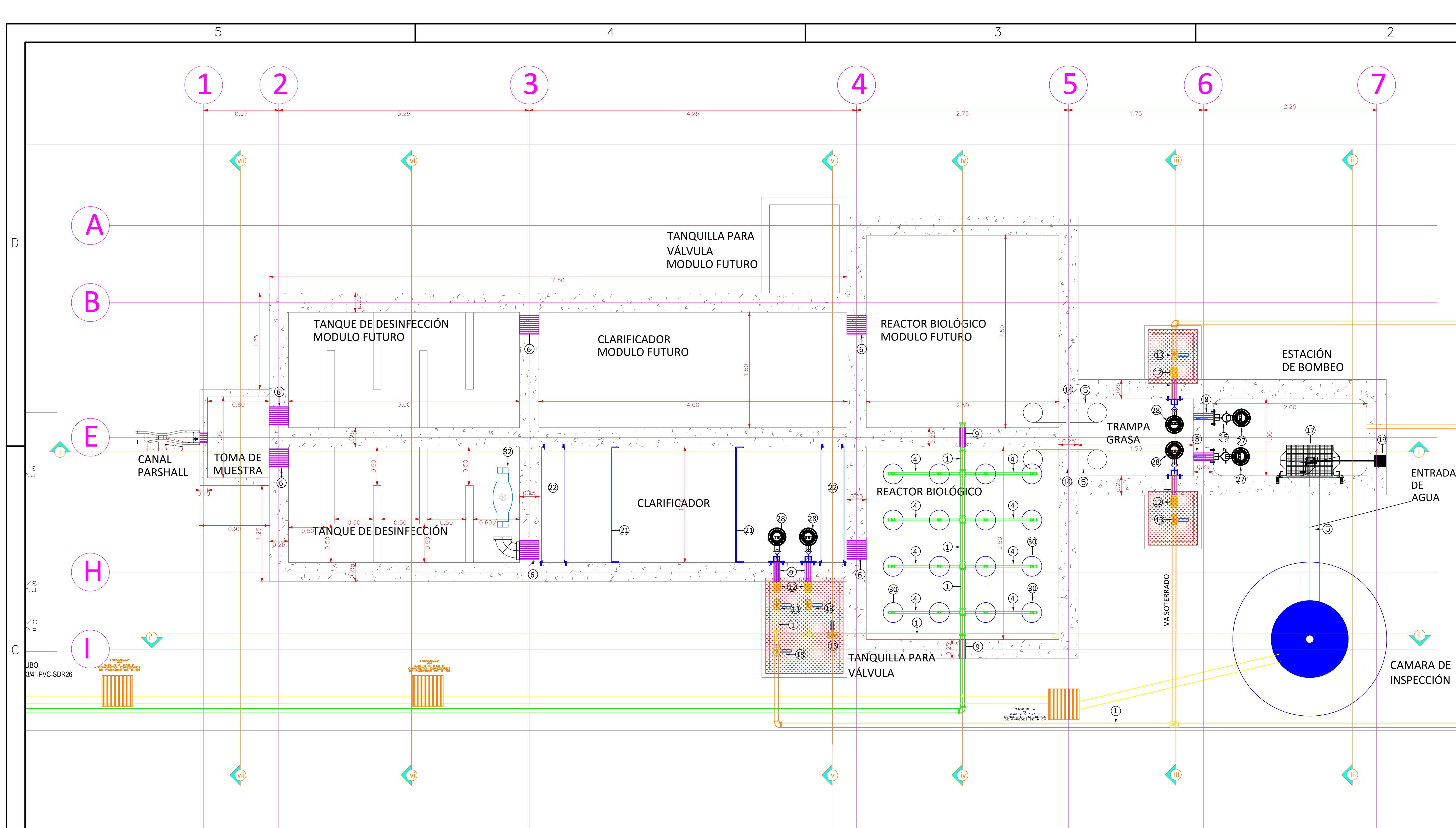
VISTA DE PLANTA Esc. 1:25
