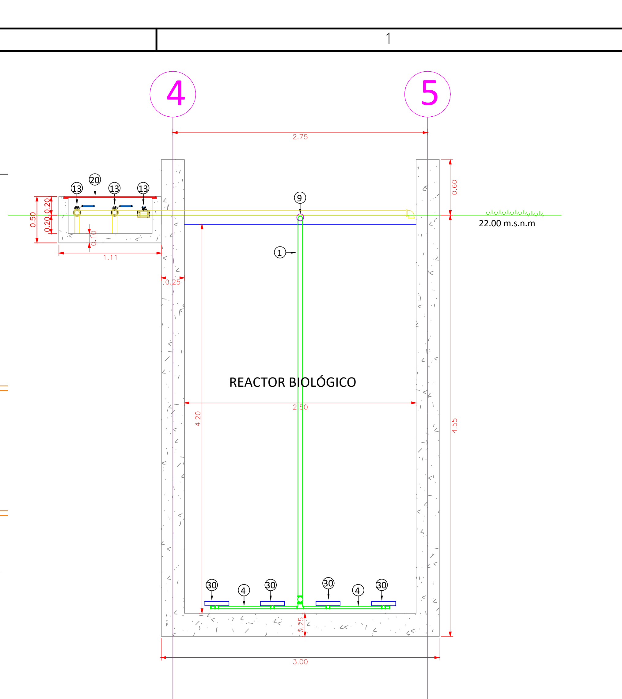
VISTA DE CORTE i' Esc. 1:25
