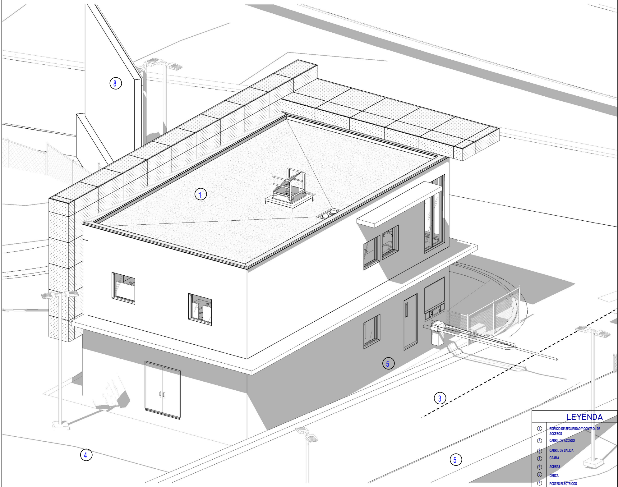
4 VISTA ISOMETRICA 4
