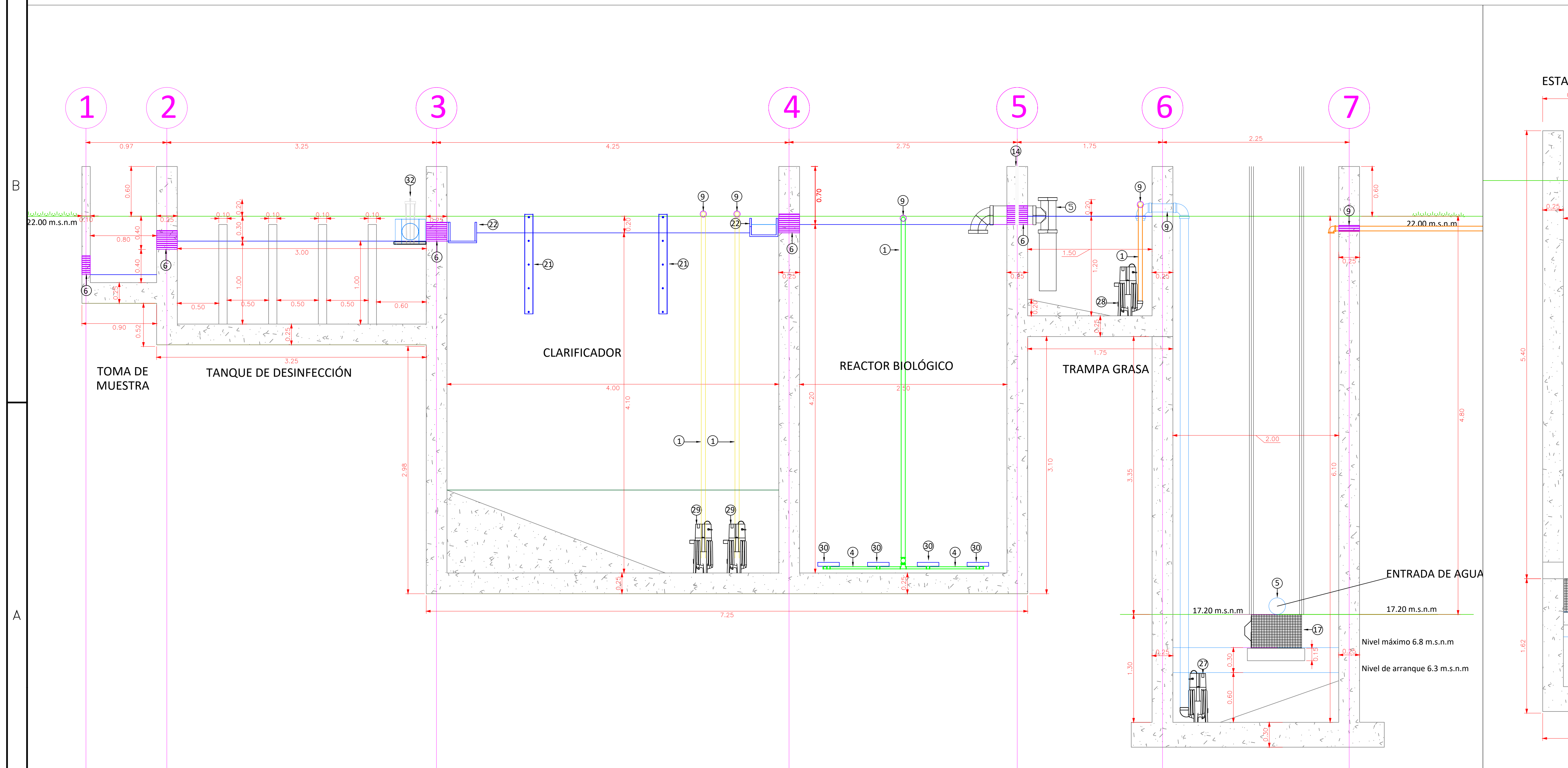
VISTA DE CORTE i Esc. 1:25
