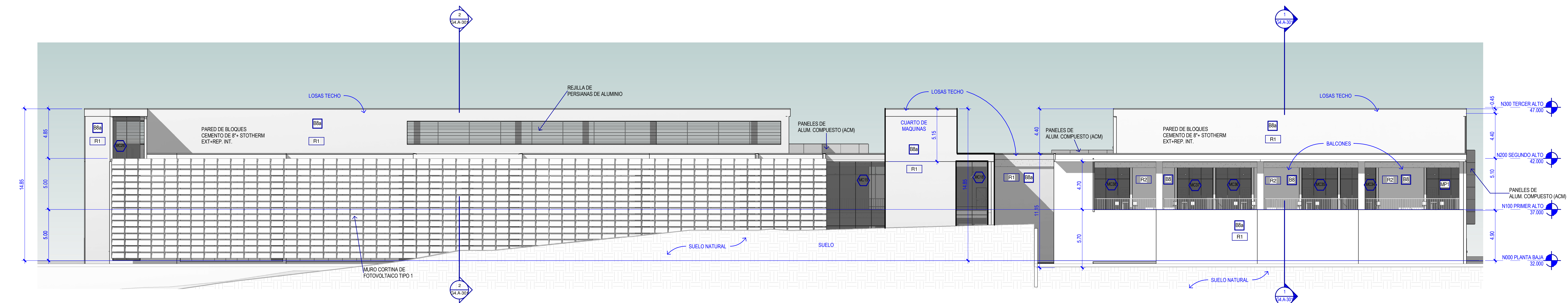
3 ELEVACION EXTERIOR - SUR 1:150
