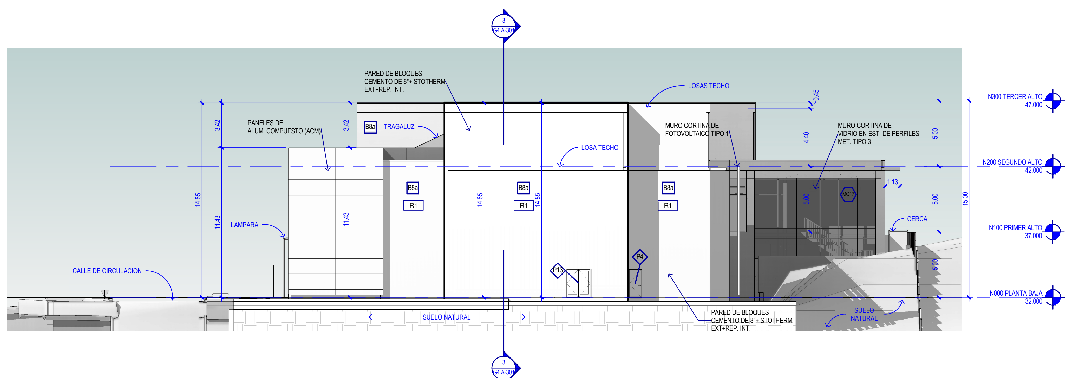
1 ELEVACION EXTERIOR - OESTE 1:150
