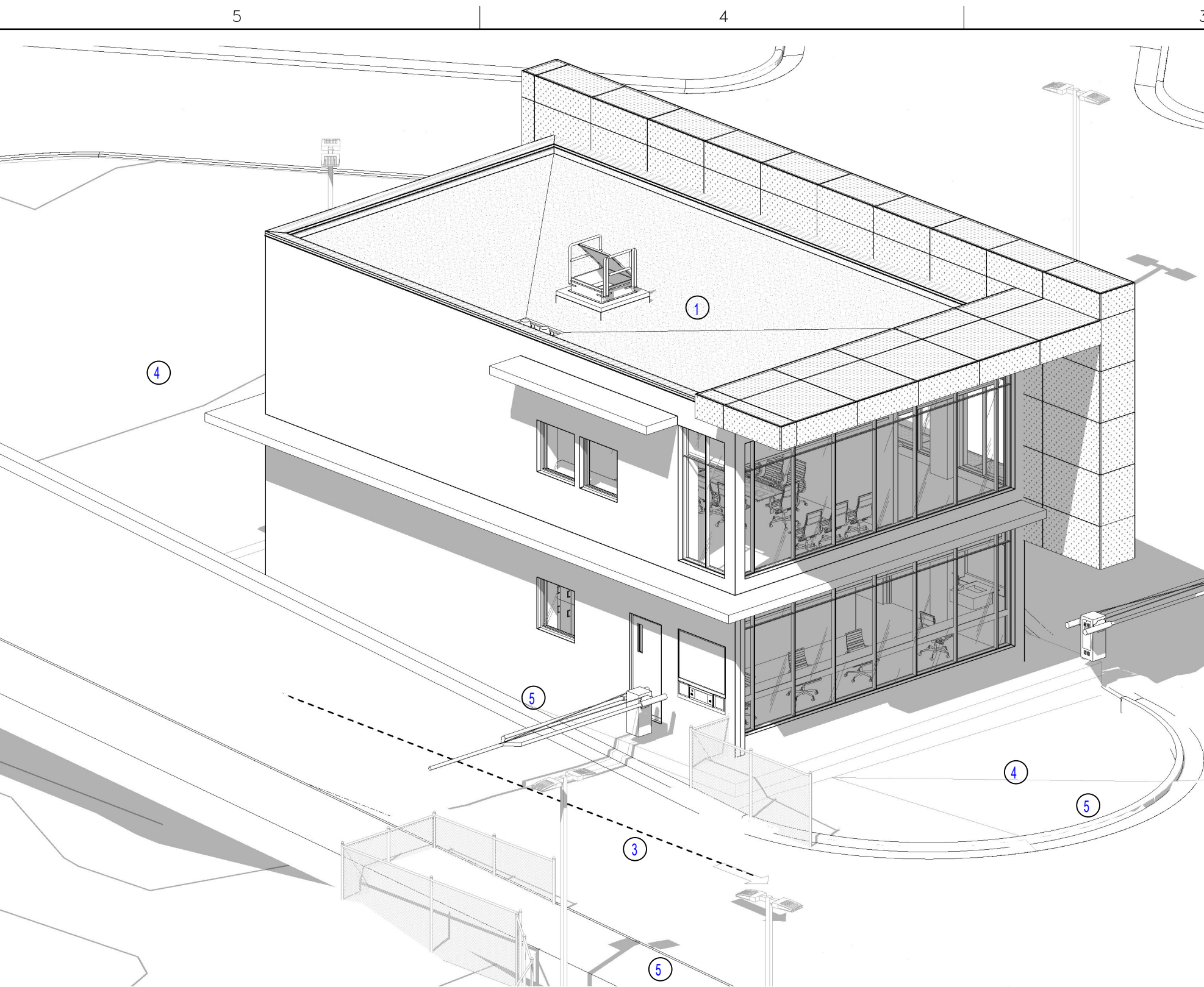
1 VISTA ISOMETRICA 1
