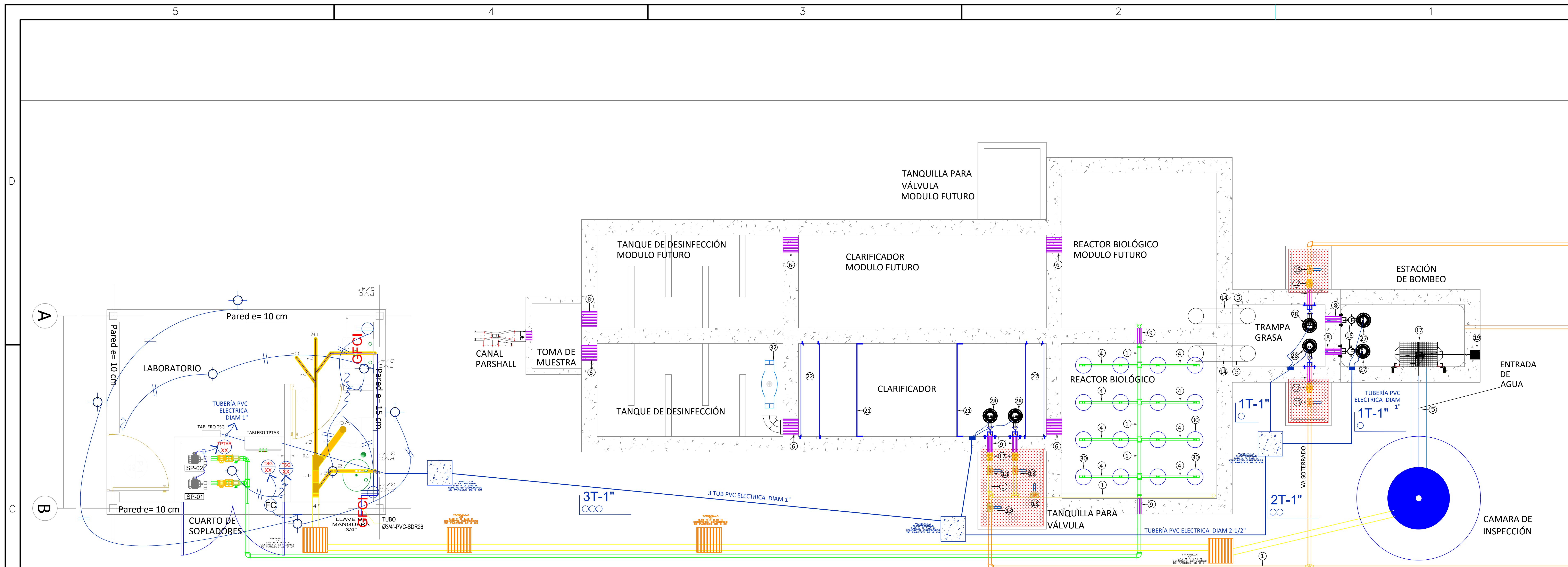
VISTA DE PLANTA PLANTA DE TRATAMIENTO DE AGUAS RESIDUALES Esc. 1:25
