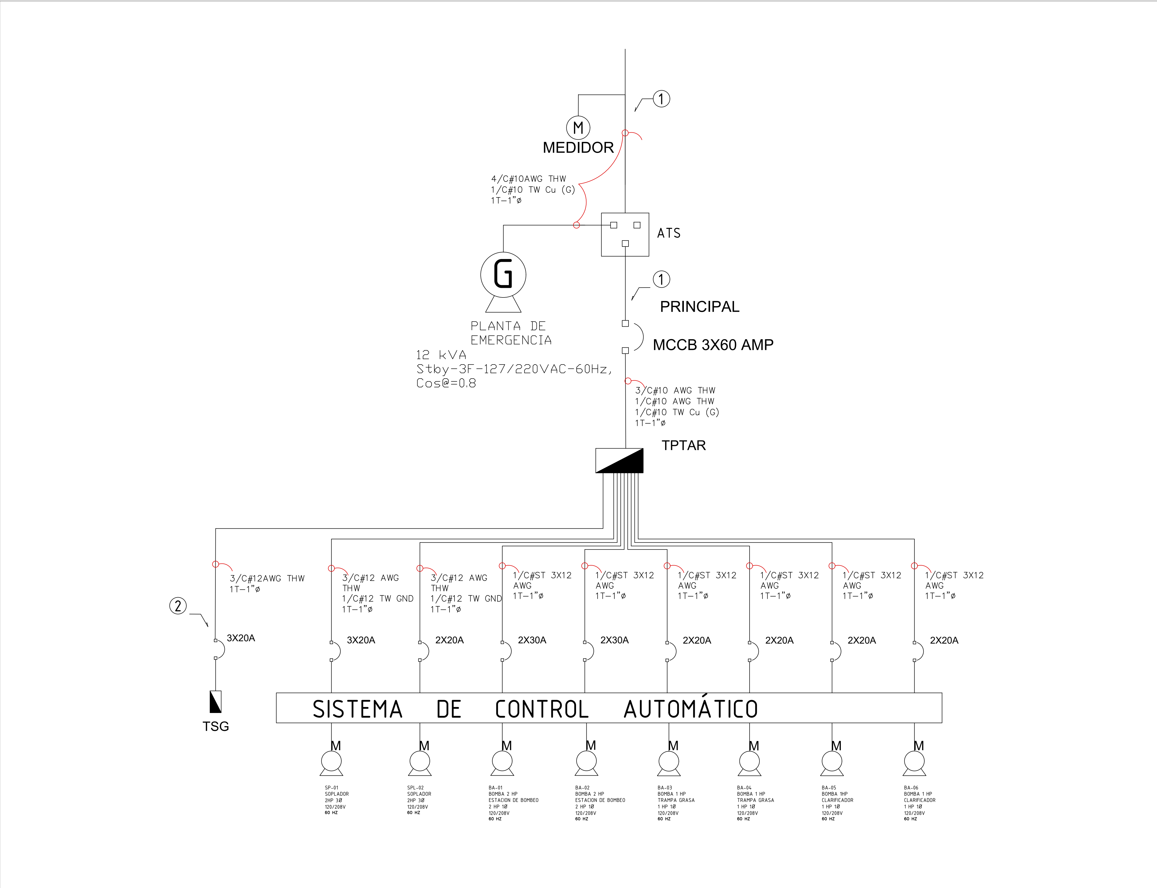
DIAGRAMA UNIFILAR Esc. S/E
