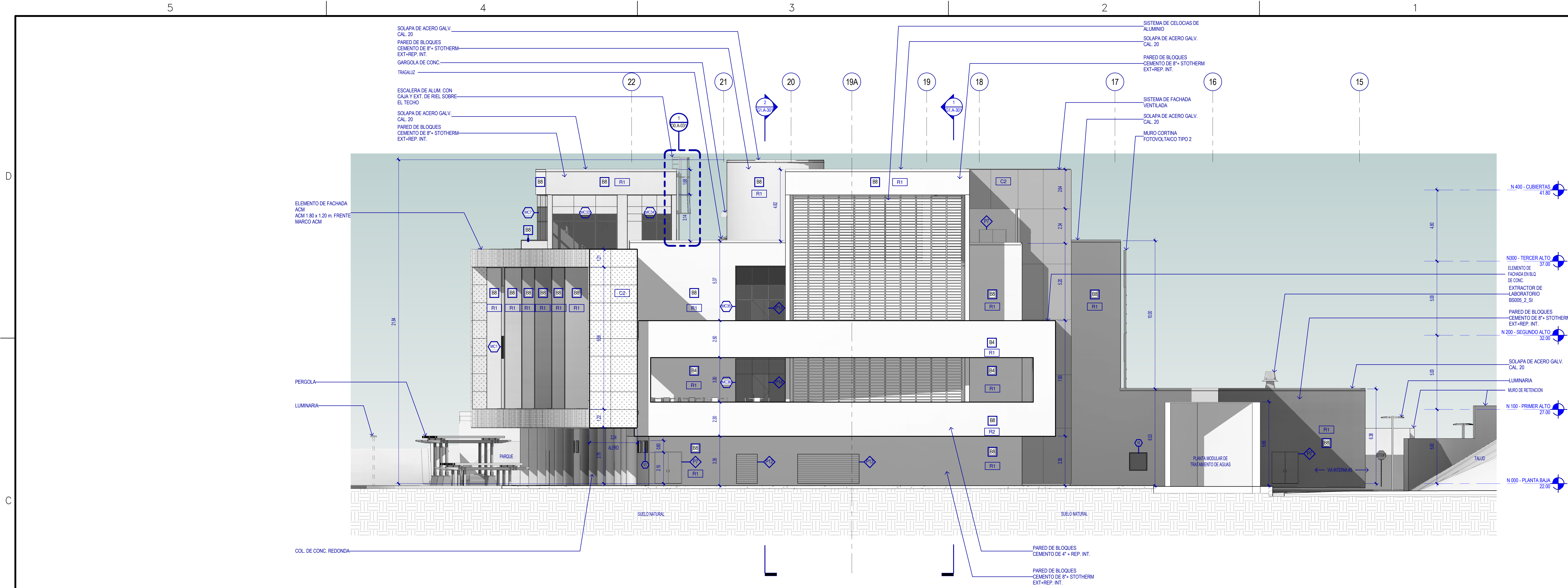
2 ELEVACION OESTE 1:100
