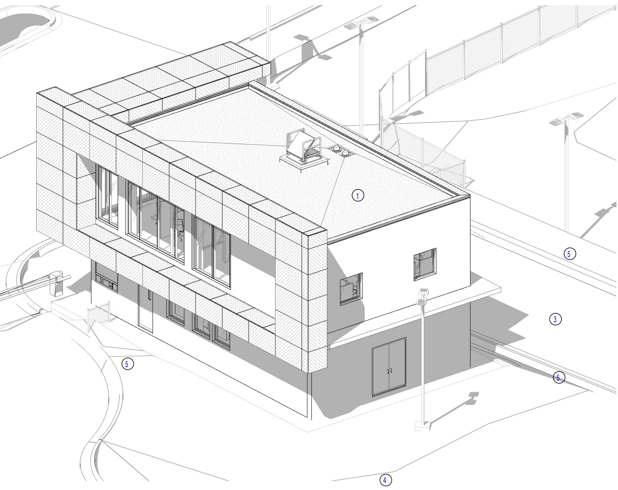
3 VISTA ISOMETRICA 3
