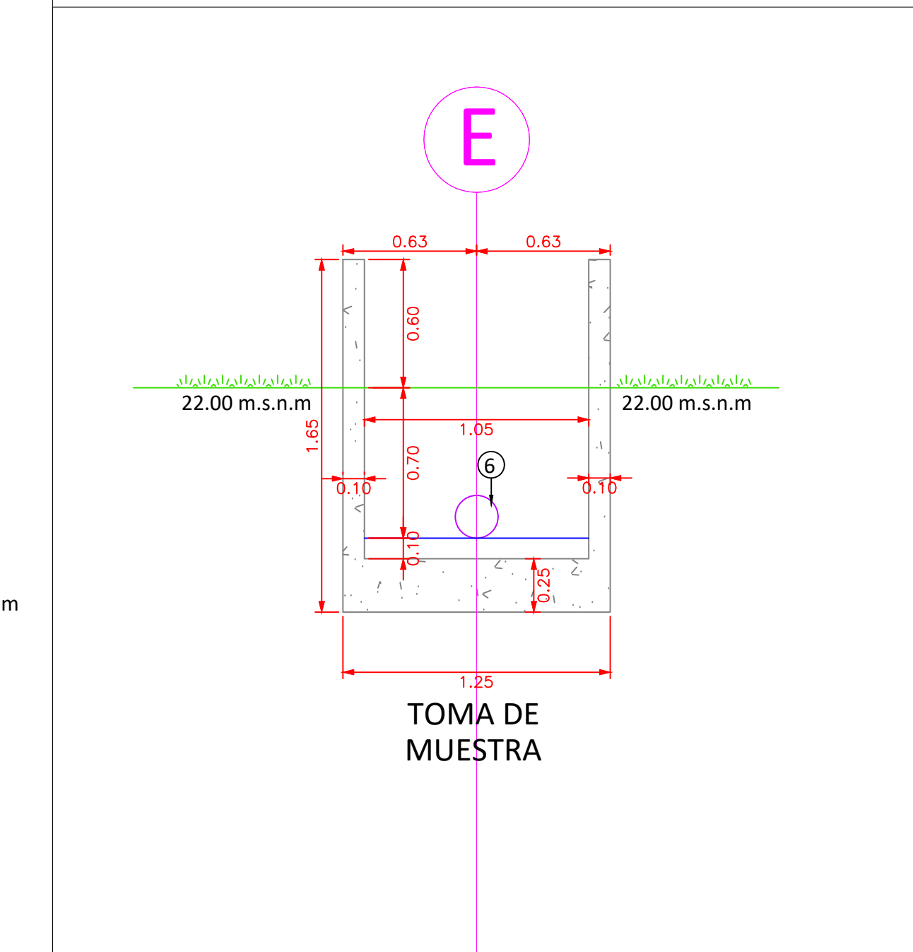
VISTA DE CORTE vii Esc. 1:25
