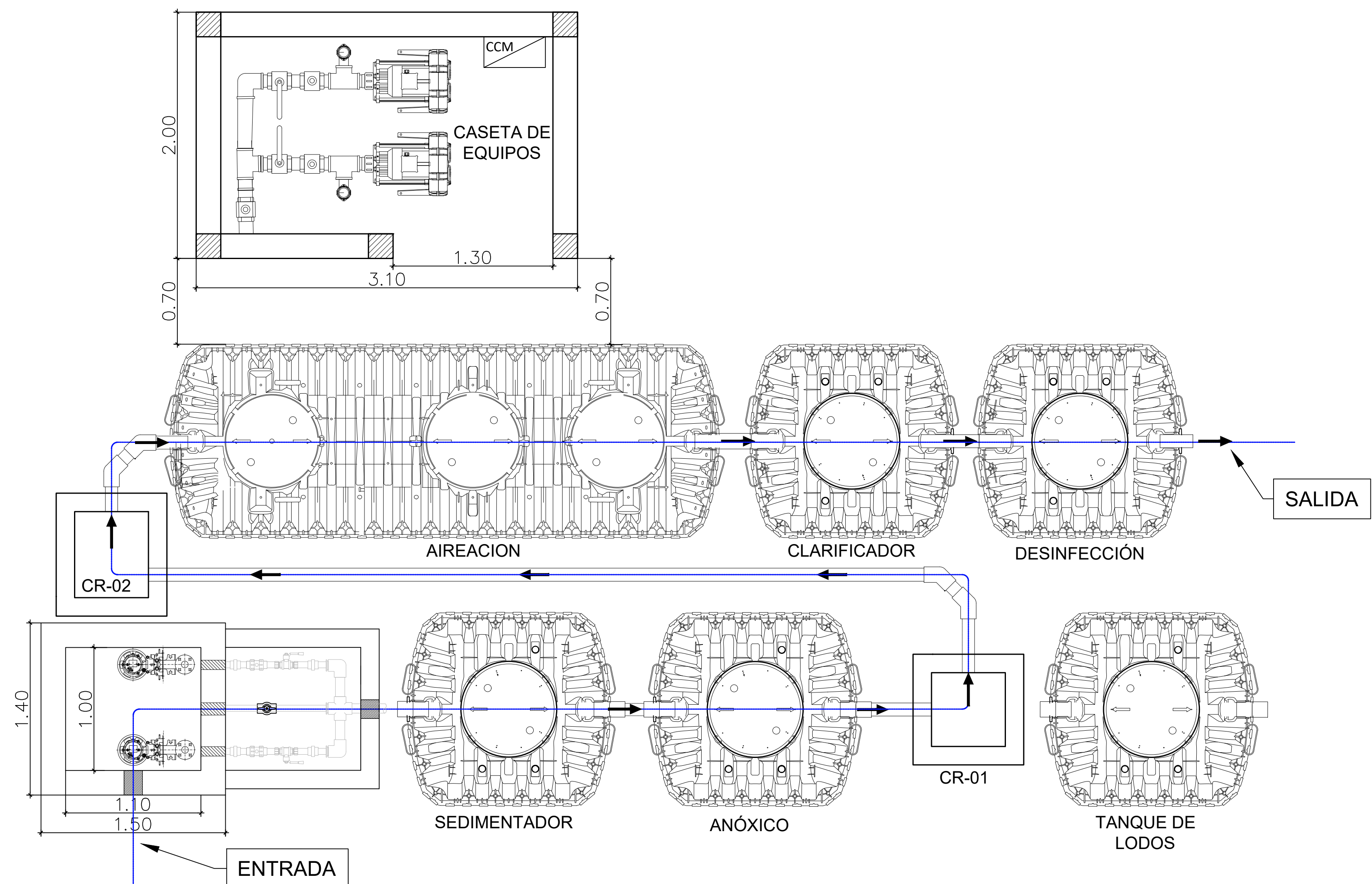
PLANTA DE TRATAMIENTO DE AGUAS RESIDUALES Escala 1:25
