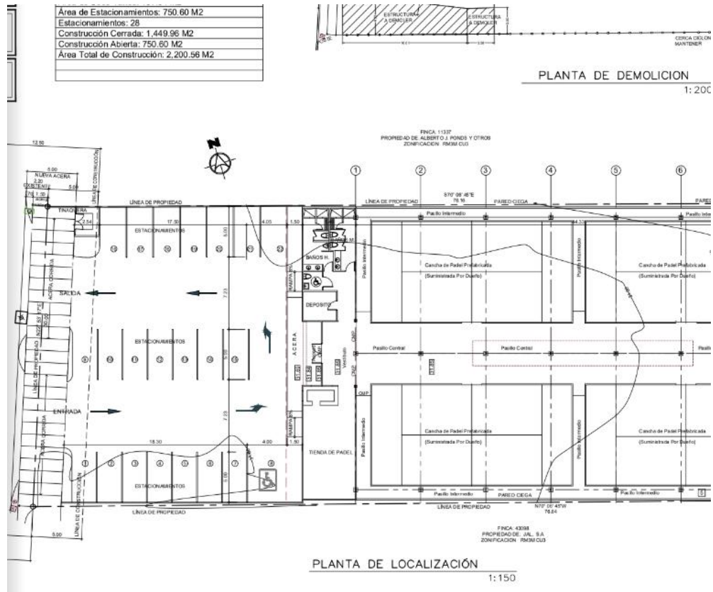
PLANO N° 1. Proyecto “COMPLEJO DEPORTIVO GUADALCANAL”
