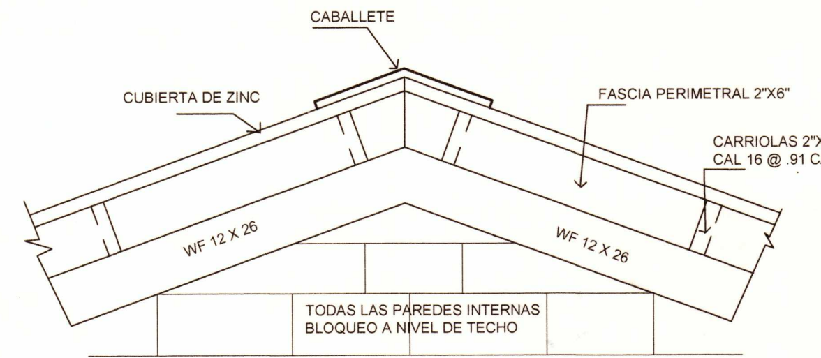
DETALLE DE TECHO - C ESC. 1/20
