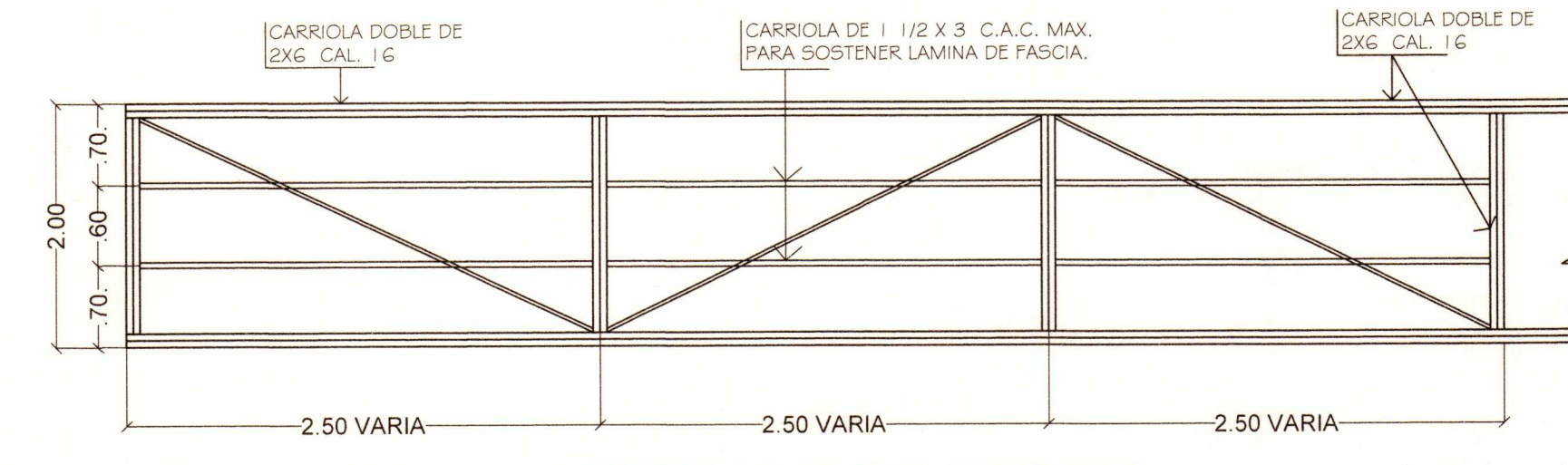
DETALLE DE FASCIA ESC. SIN/ESC
