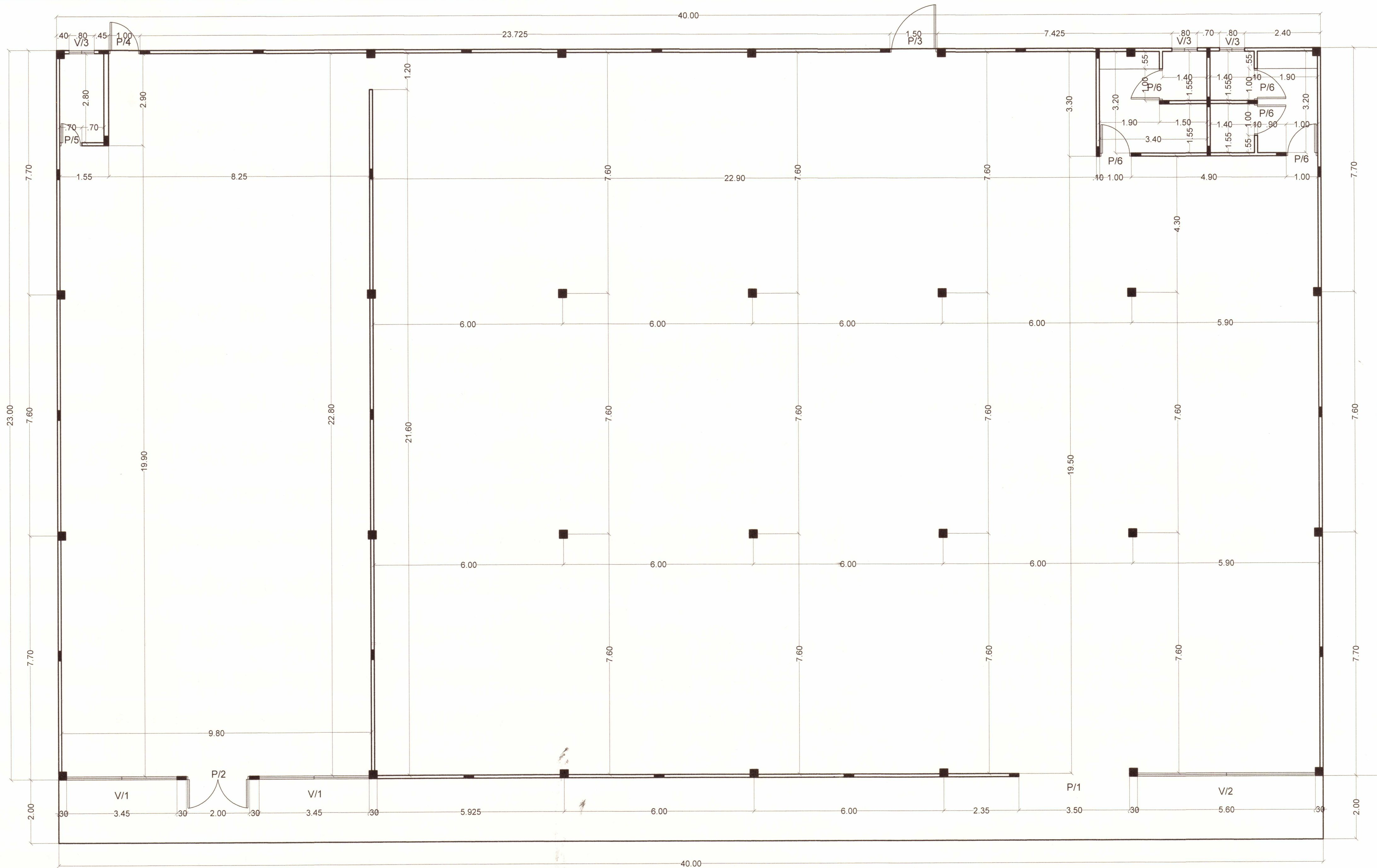
PLANTA ARQUITECTONICA BAJA
