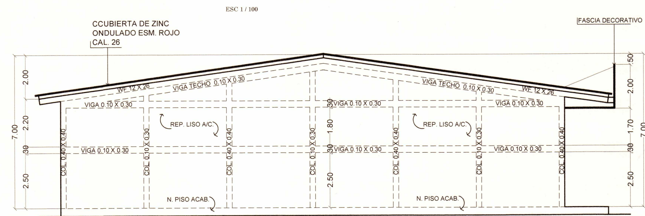
FACHADA LAT. IZQUIERDA ESC. 1/100
