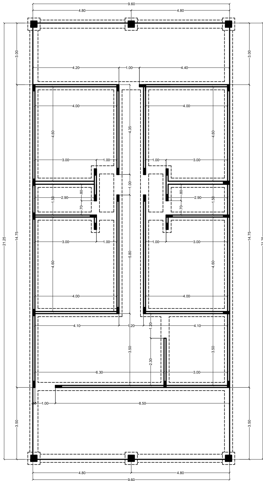
PLANTA DE FUNDACION ESC 1/50
