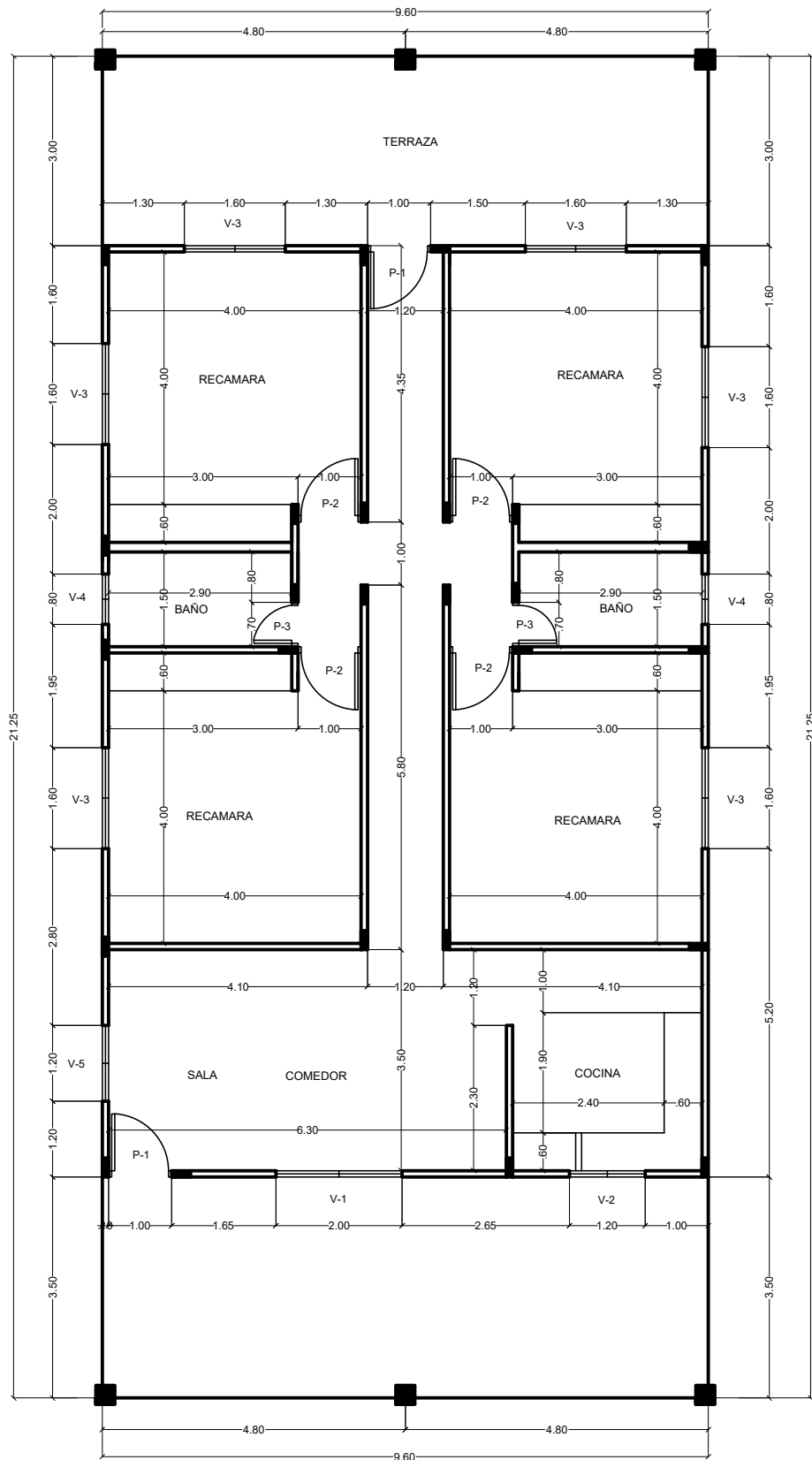
PLANTA ARQUITECTONICA ESC 1/50
