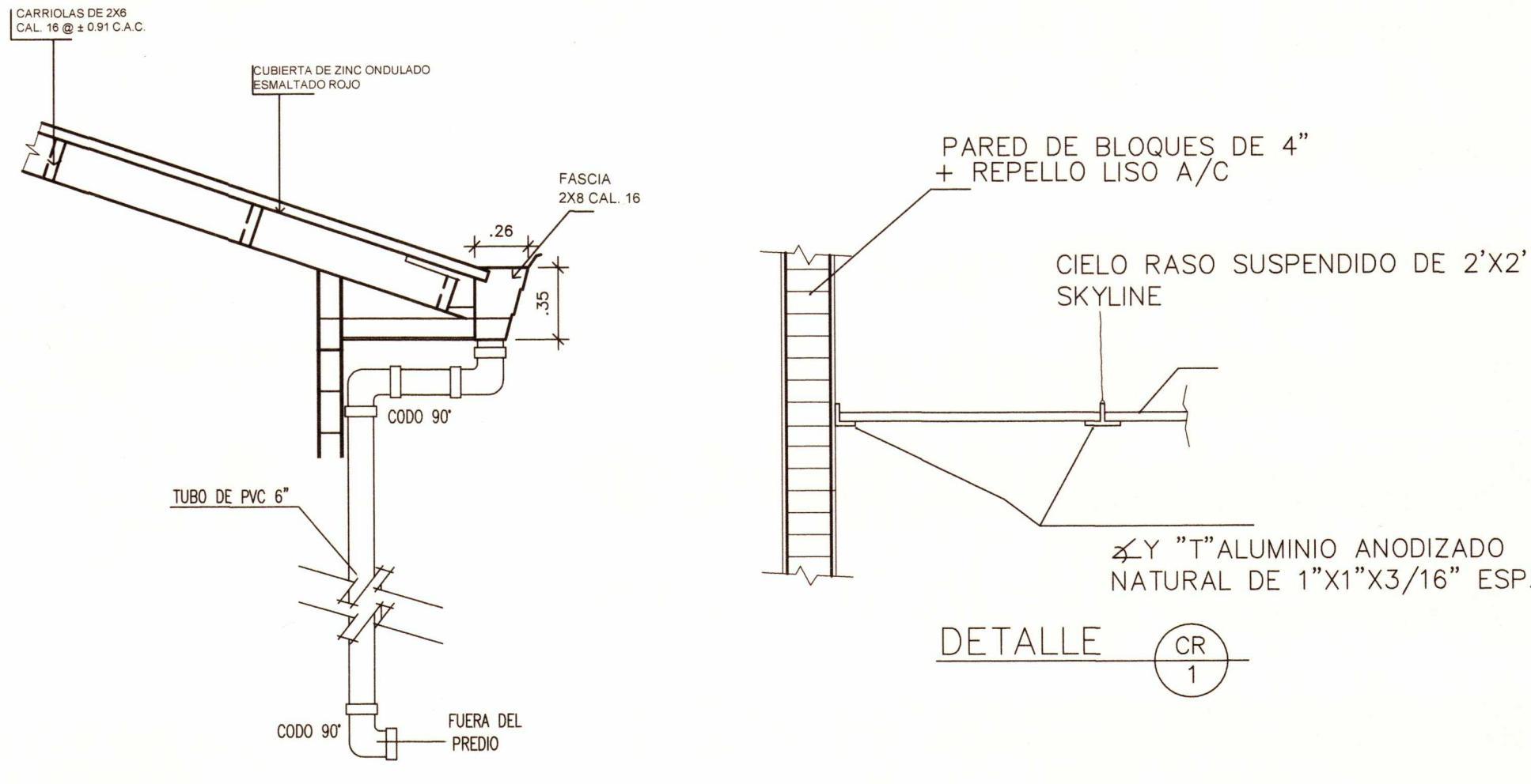
DETALLE DE TECHO T/1 ESC. 1/20
