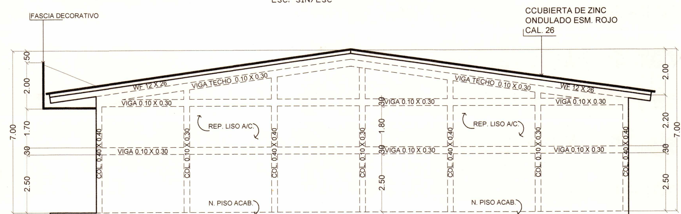
FACHADA LAT. DERECHA ESC. 1/100
