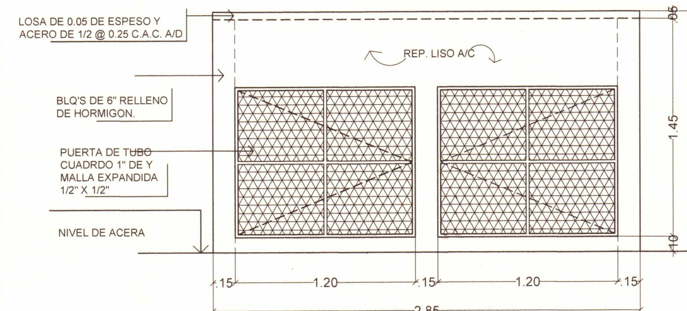
ELEVACION DE TINQUERA
