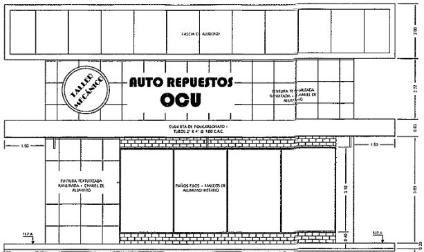
ELEVACIÓN FRONTAL
