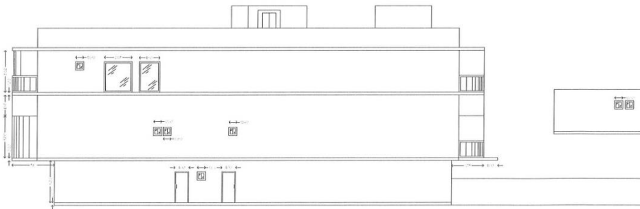
FACHADA LATERAL DERECHA ESC. 1:100
