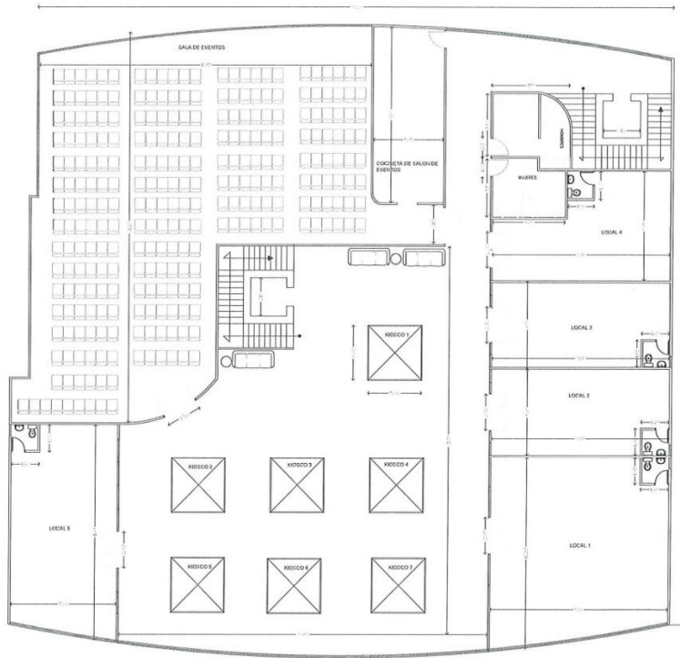
PLANTA ARQUITECTÓNICA 2º NIVEL ESC. 1:100
