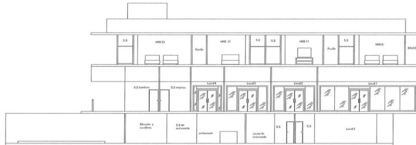
CORTE LONGITUDINAL B-B' ESC. 1:75
