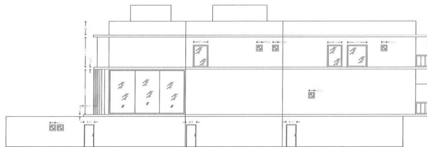
FACHADA LATERAL IZQUIERDA ESC. 1:100
