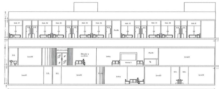
CORTE TRANSVERSAL A-A' ESC. 1:75
