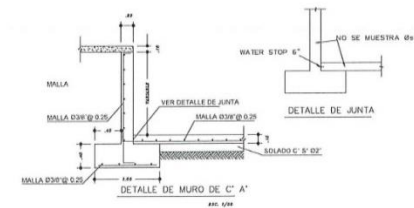
PLANO DE DETALLES PISCINA ESC. 1:50
