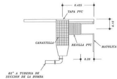
DETALLE DESNATADOR PLANO DE DETALLES PISCINA ESC. 1/25 ESC. 1:25
