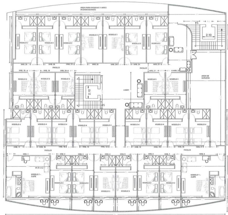
PLANTA ARQUITECTÓNICA 3° NIVEL ESC. 1:100
