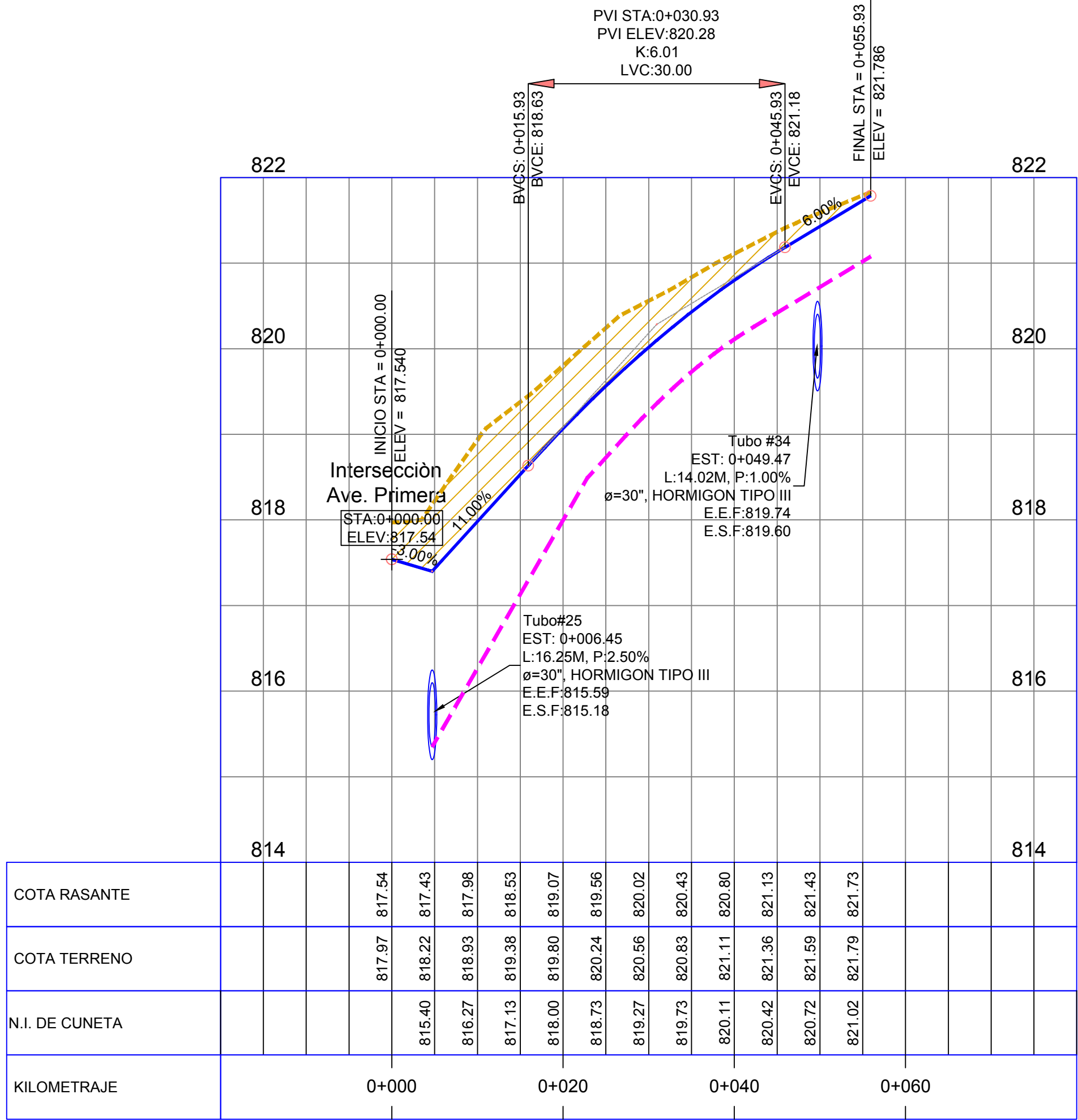
Plano Perfil - Calle D
