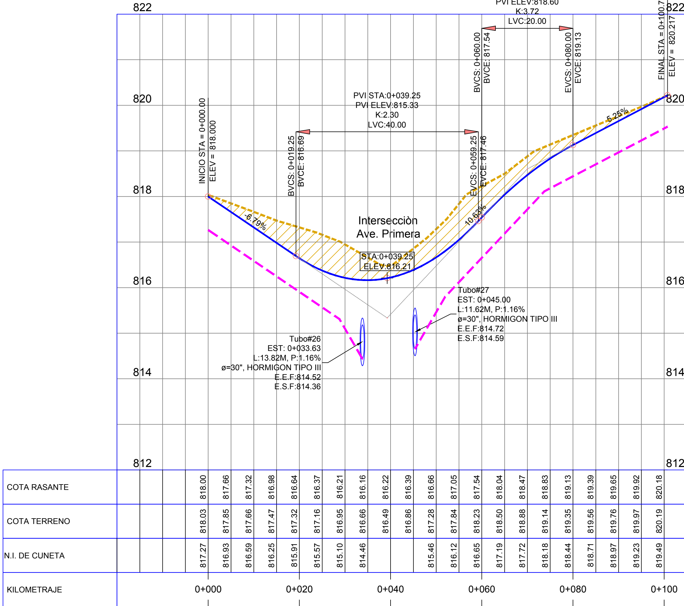
Plano Perfil - Calle C
