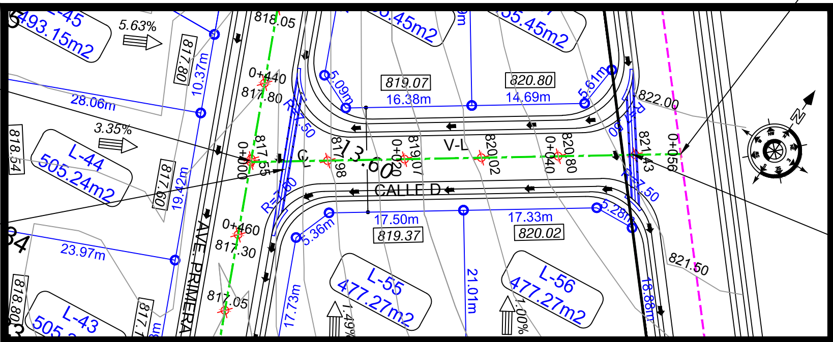
Plano Perfil - Calle D
