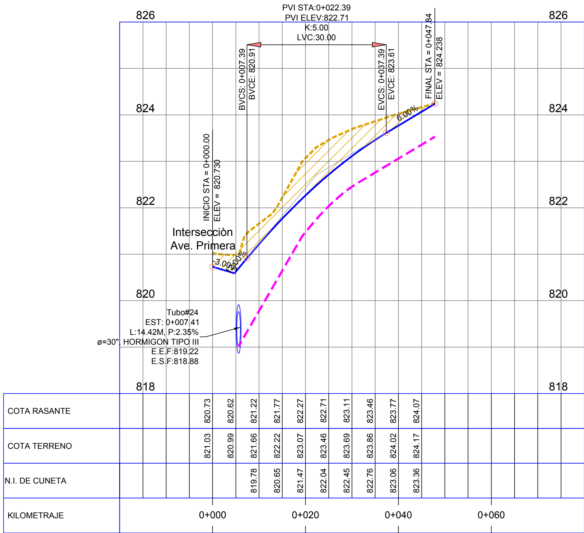
Plano Perfil - Calle E
