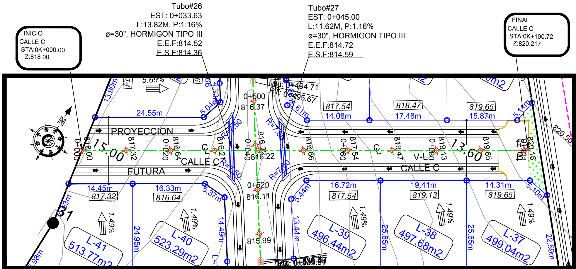
Plano Perfil - Calle C
