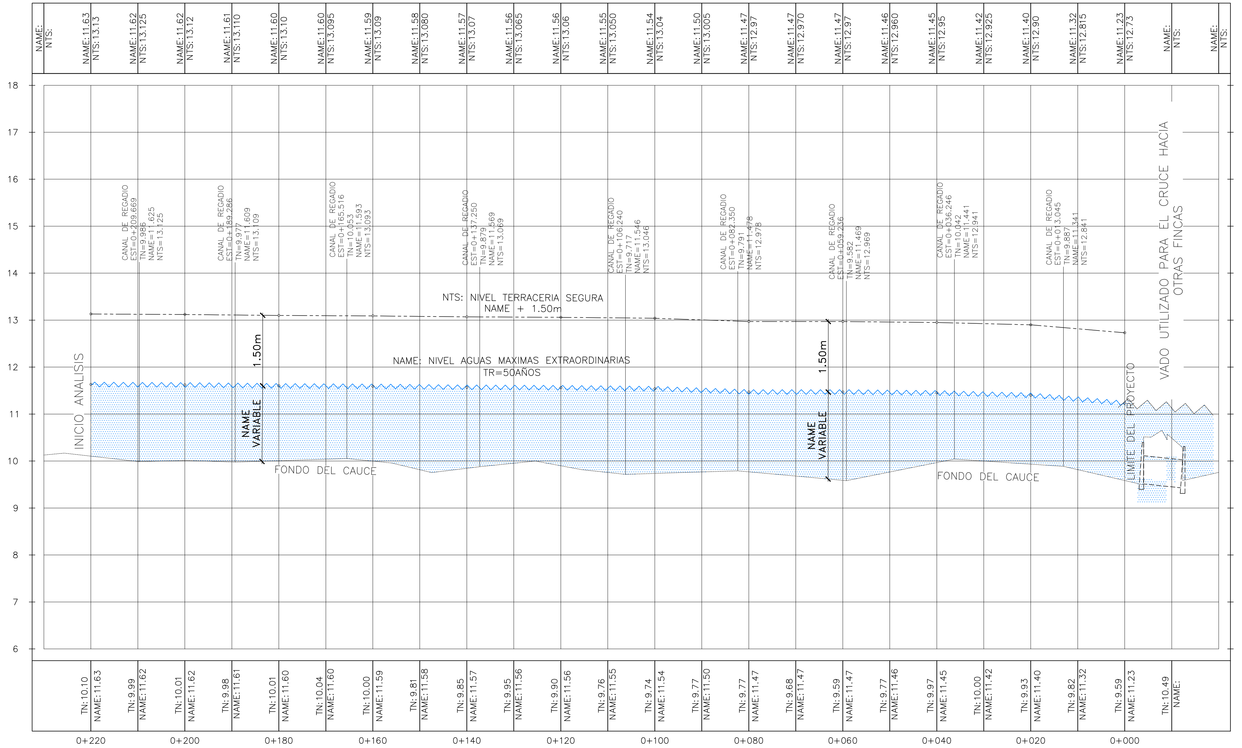
PERFIL- CANAL DE REGADIO ESC V. 1:50 ESC H. 1:500
