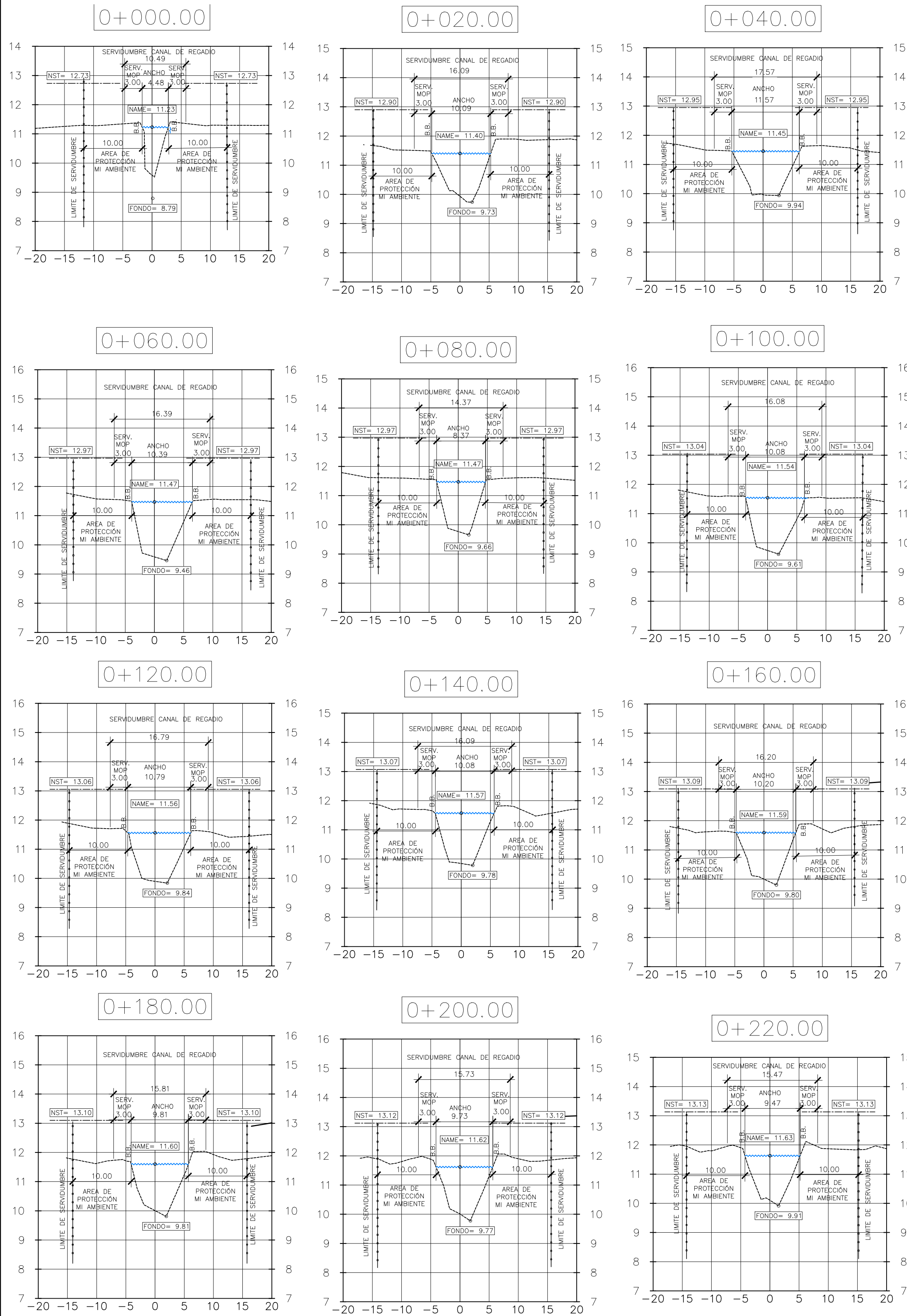
SECCIONES TRANSVERSALES- CANAL DE REGADIO ESC V. 1:50 ESC H. 1:500
