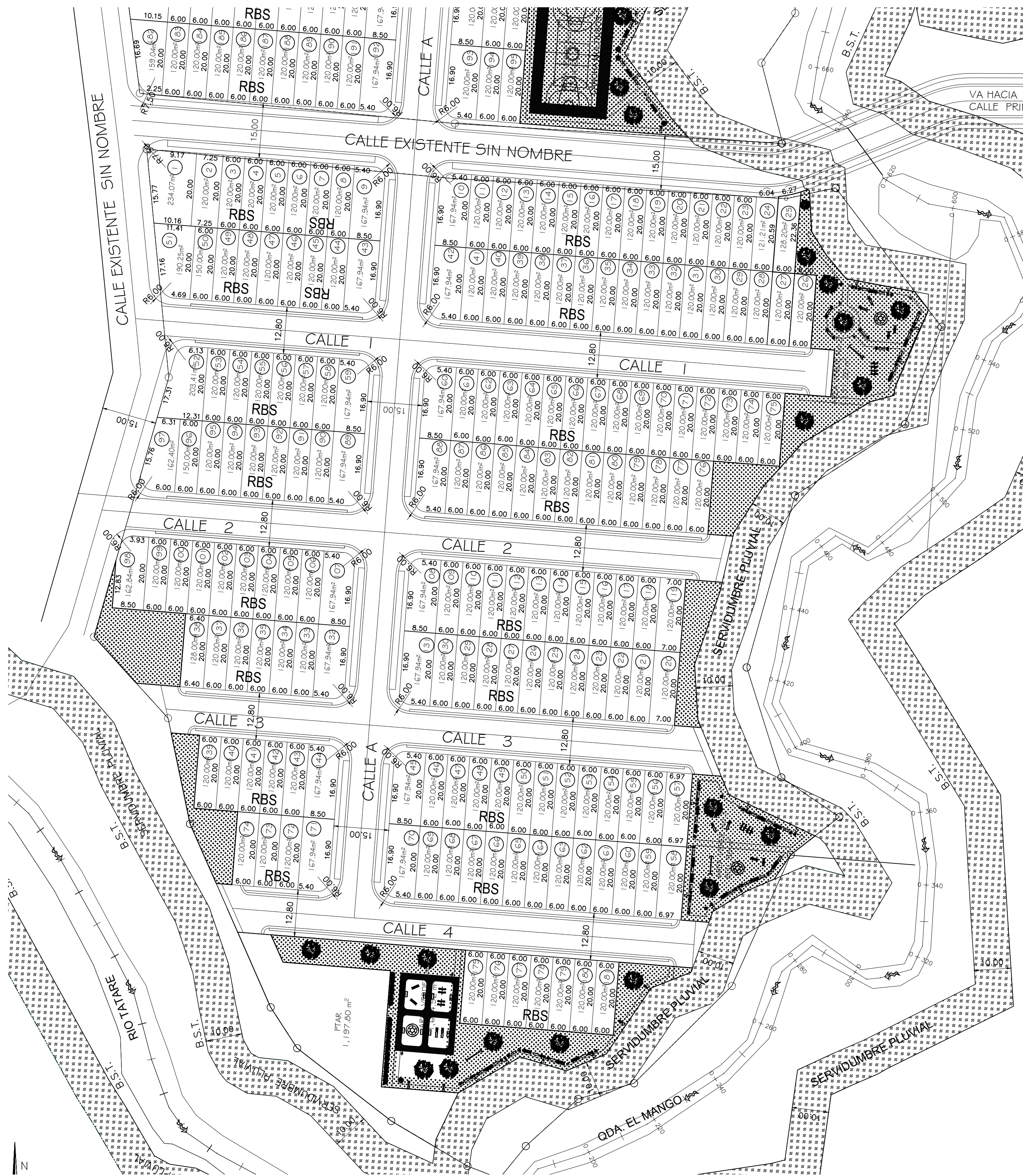
PLANTA DE LOTIFICACIÓN DEL ESTUDIO ORIGINAL
