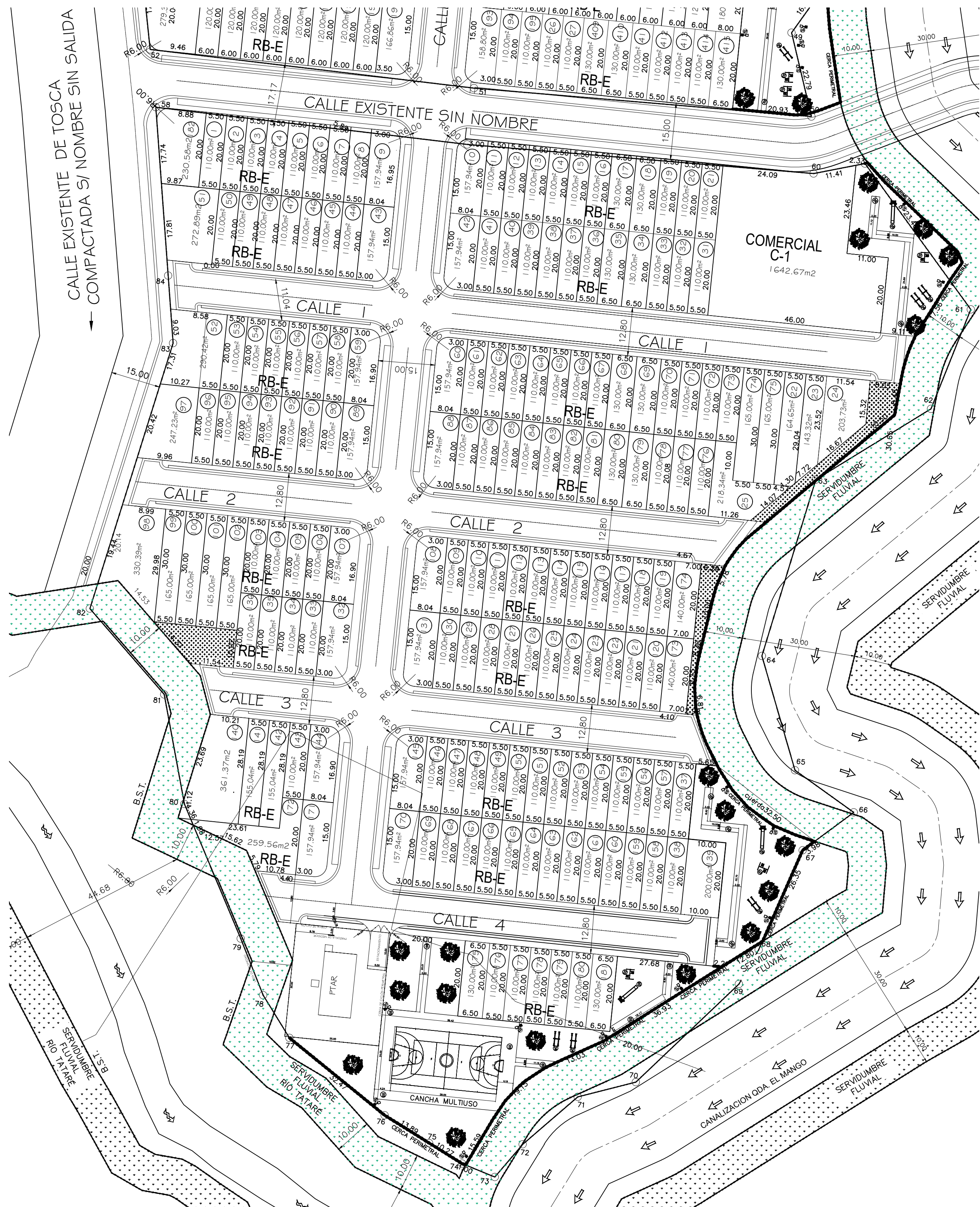
PLANTA DE LOTIFICACIÓN MODIFICADA
