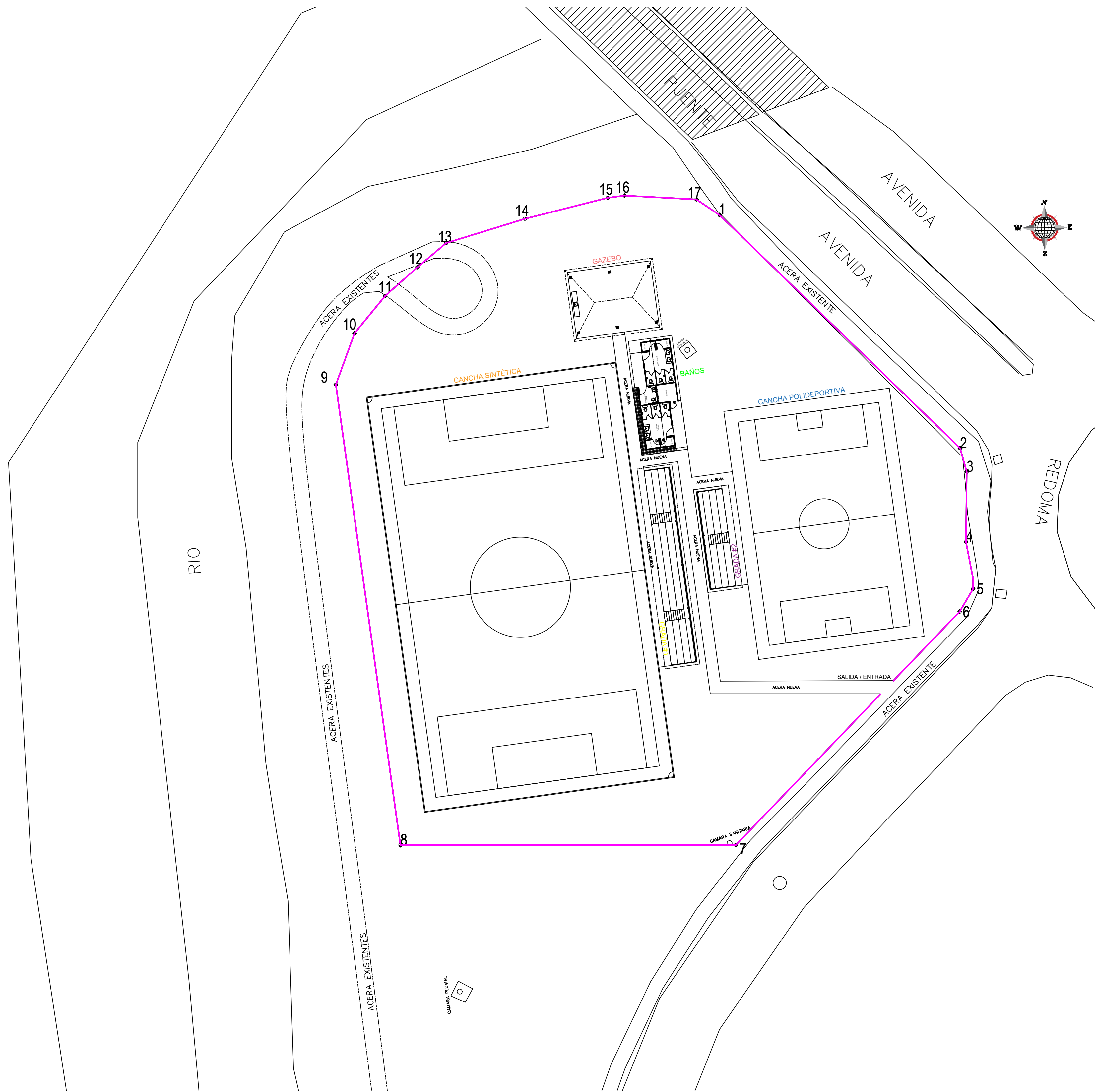
LOCALIZACION GENERAL - AREA A CONSTRUIR ESC.1:300
