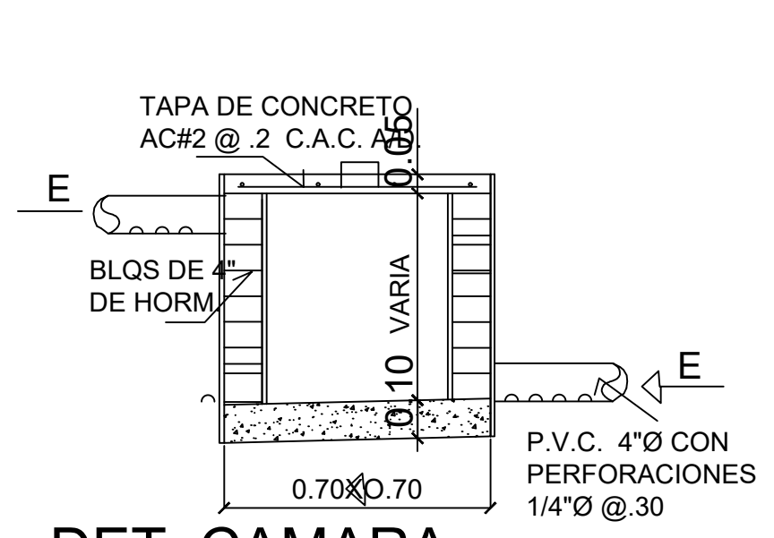
DET. CAMARA DE INSPECCION ESC. 1:20
