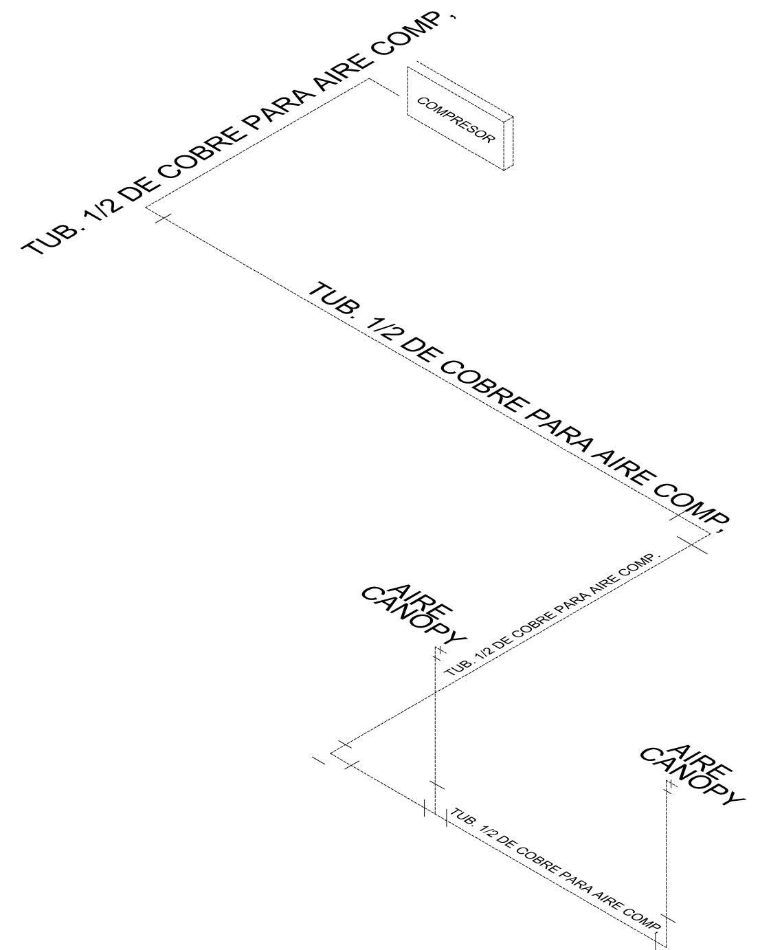
ISOMETRICO DE COMPRESOR DE AIRE
