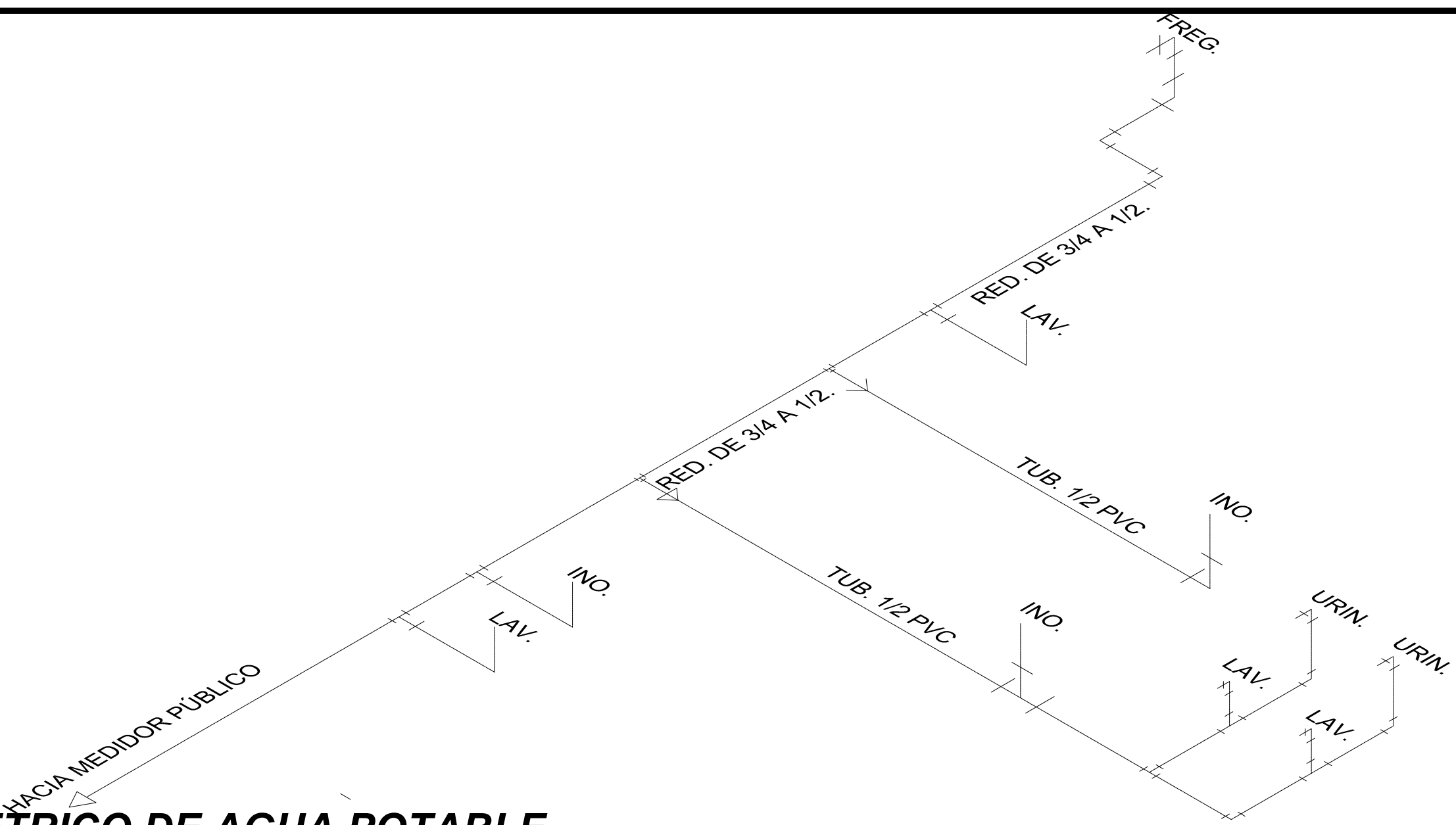
ISOMETRICO DE AGUA POTABLE
