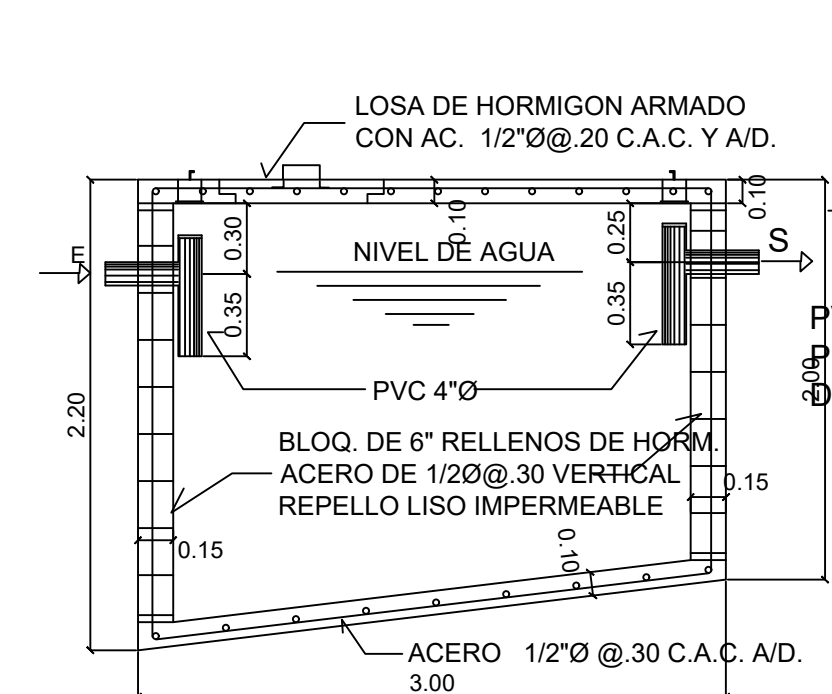
SECCION TANQUE SEPTICO ESC. 1:20
