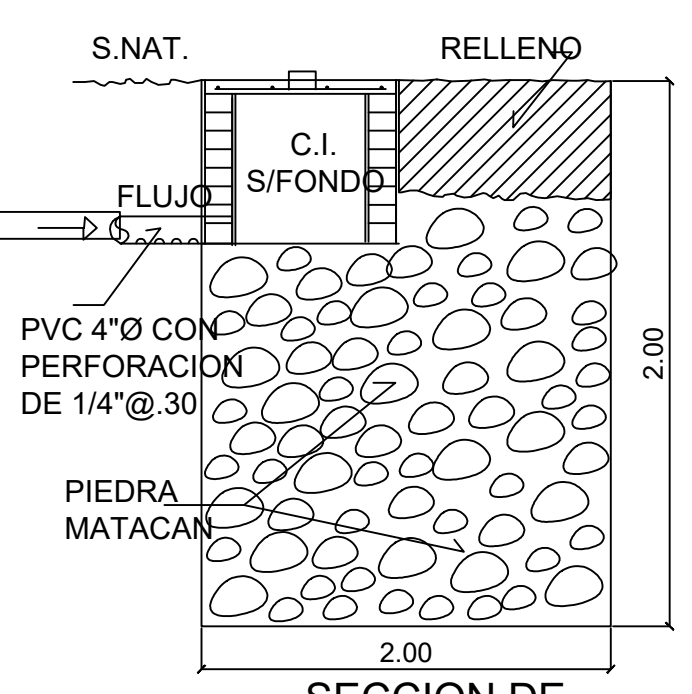
SECCION DE SUMIDERO ESC. 1:20
