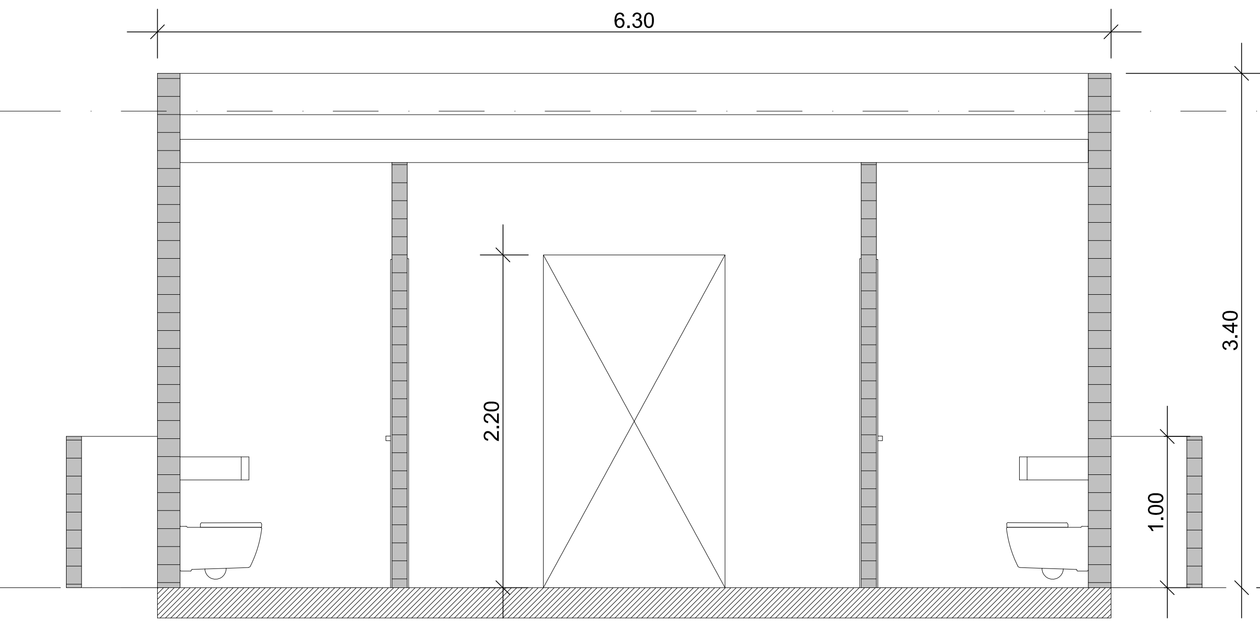
SECCIÓN LONGITUDINAL
