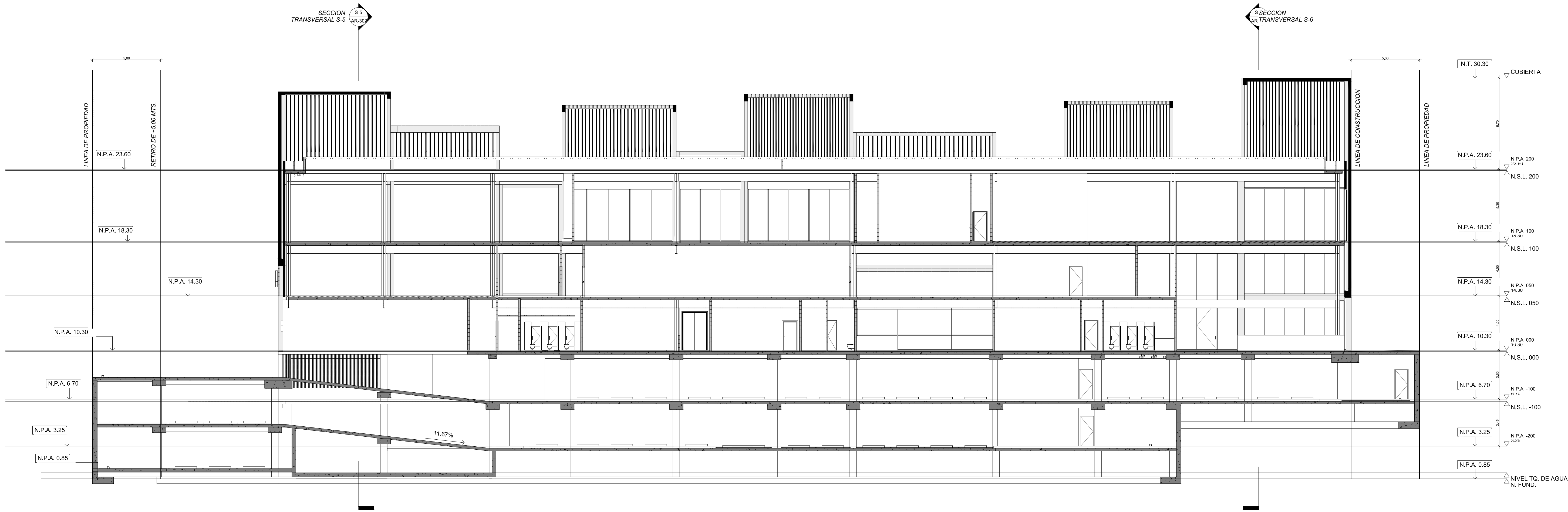
SECCIÓN LONGITUDINAL 1 ESC. 1:100
