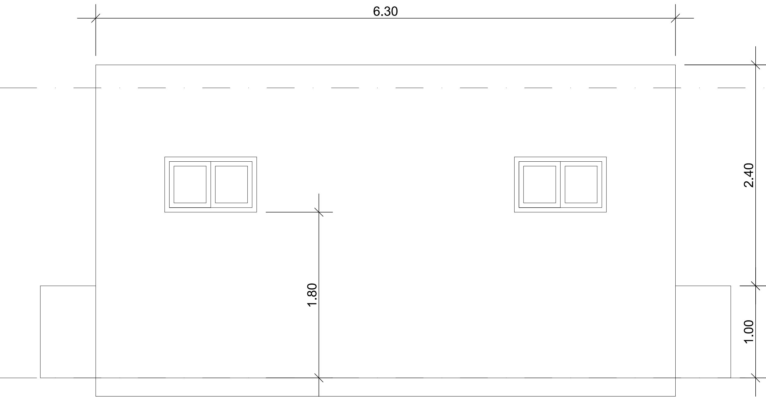
ELEVACIÓN POSTERIOR
