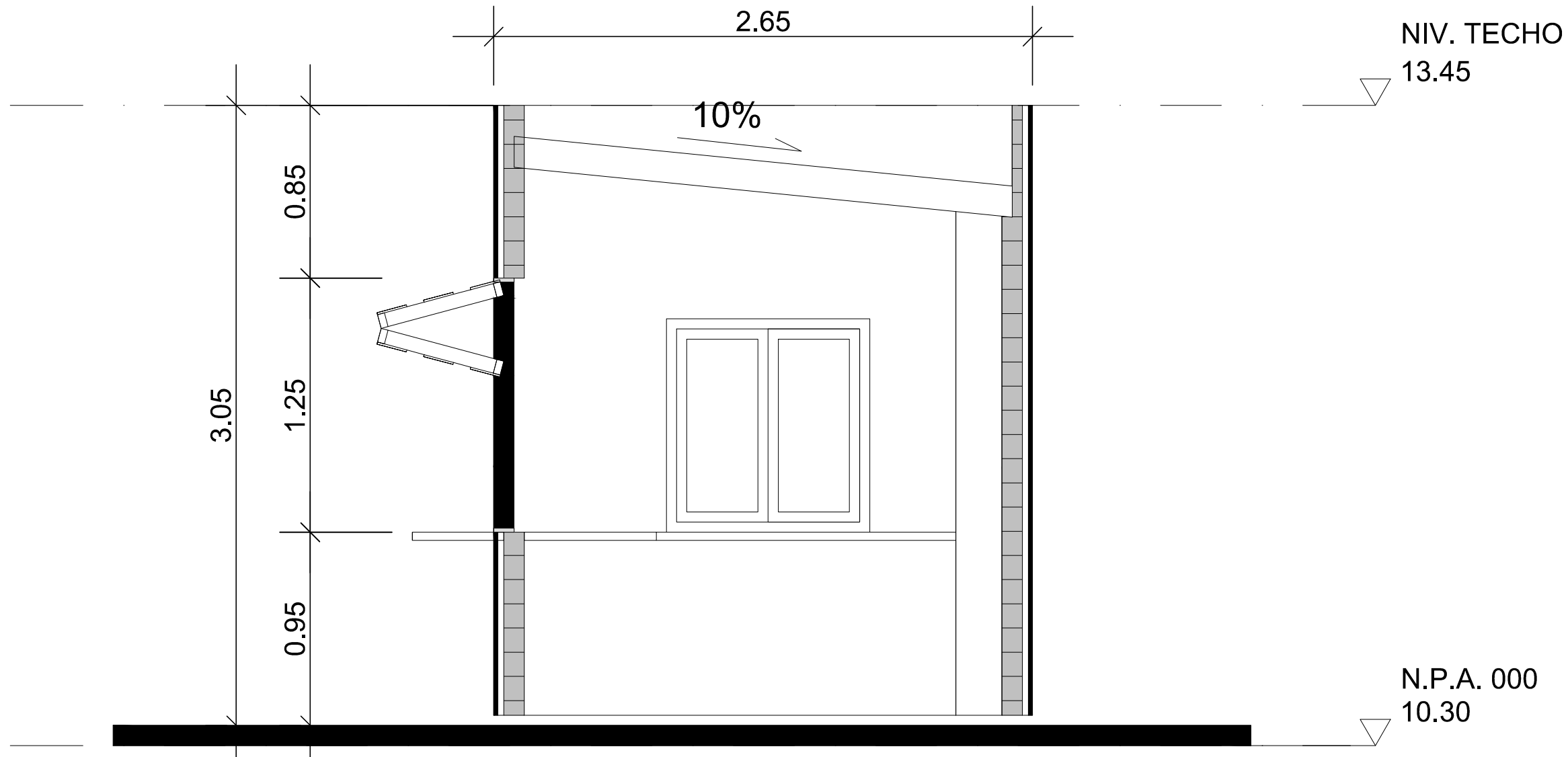
SECCIÓN LONGITUDINAL
