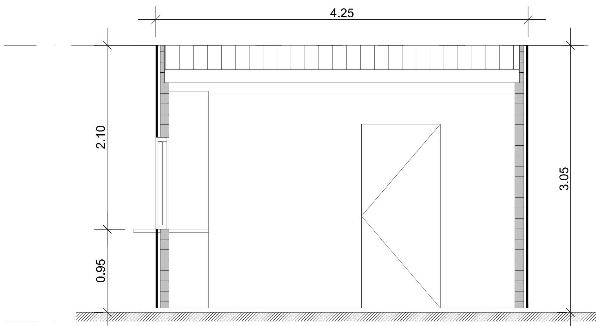
SECCIÓN TRANSVERSAL
