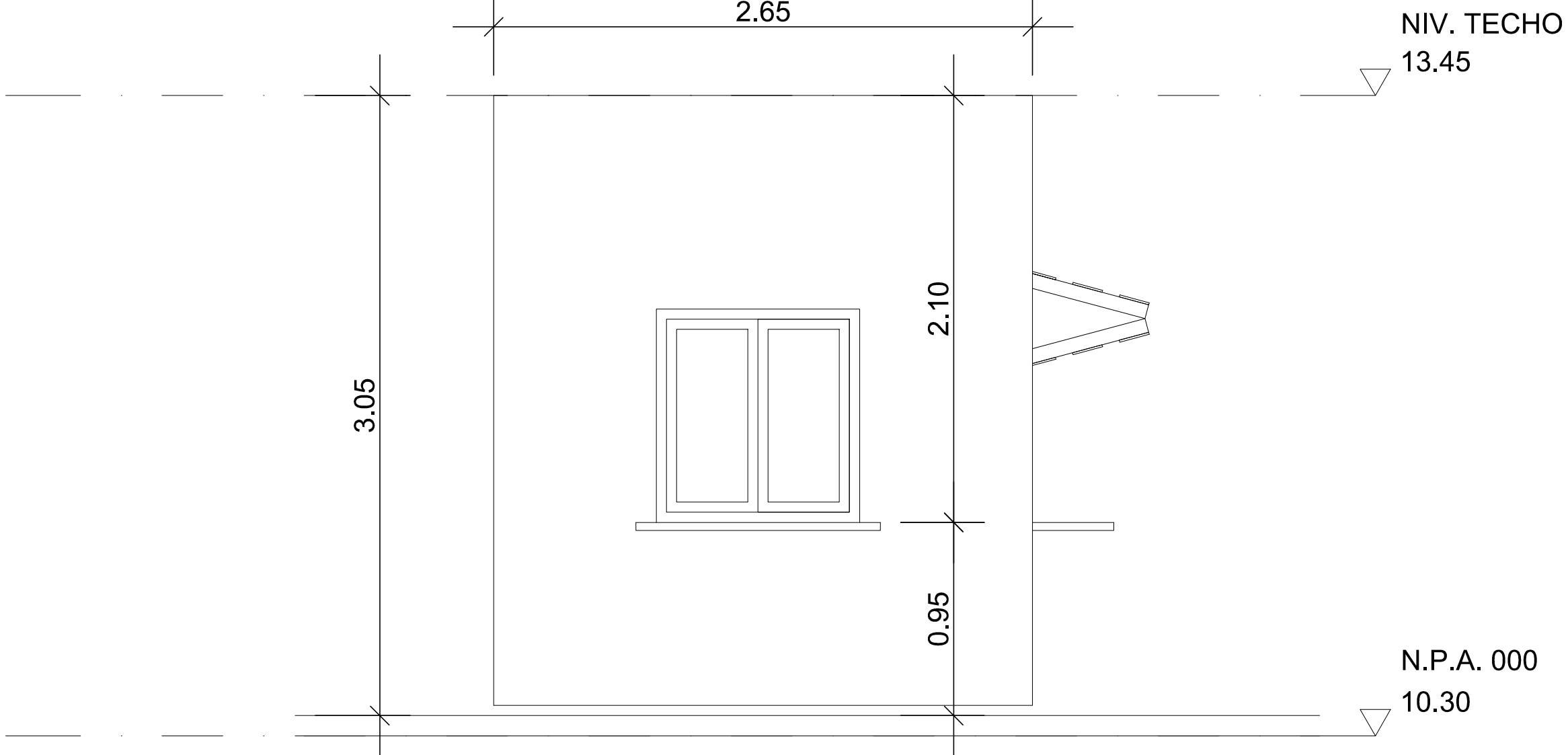
SECCIÓN TRANSVERSAL 1
