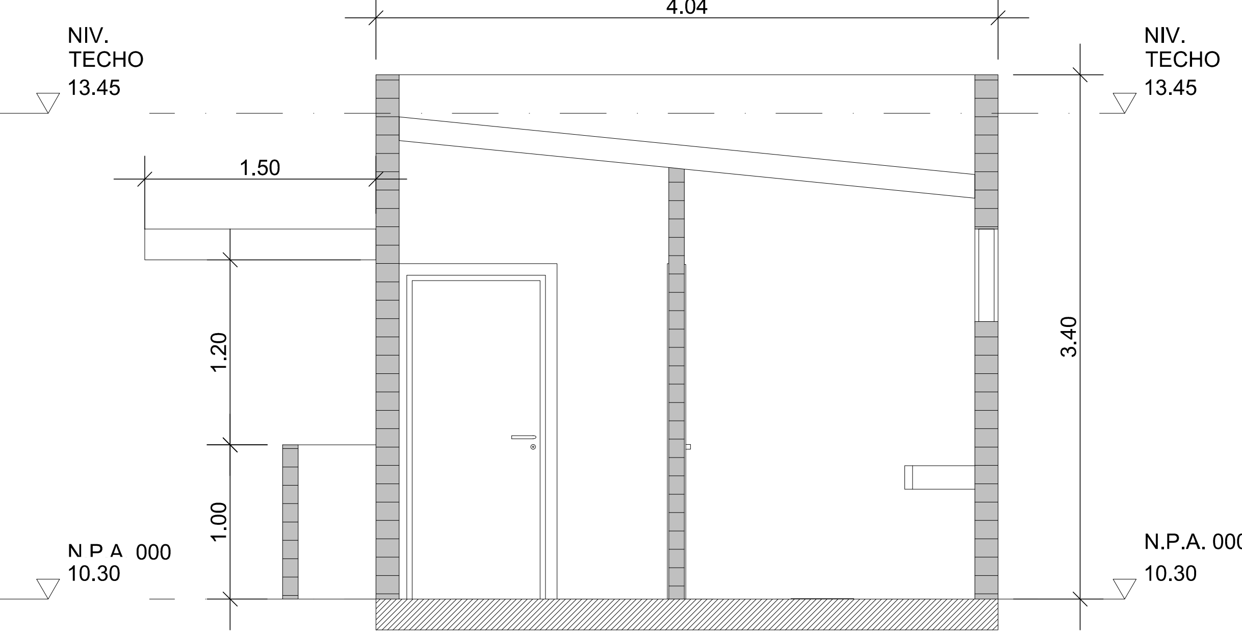
SECCIÓN TRANSVERSAL
