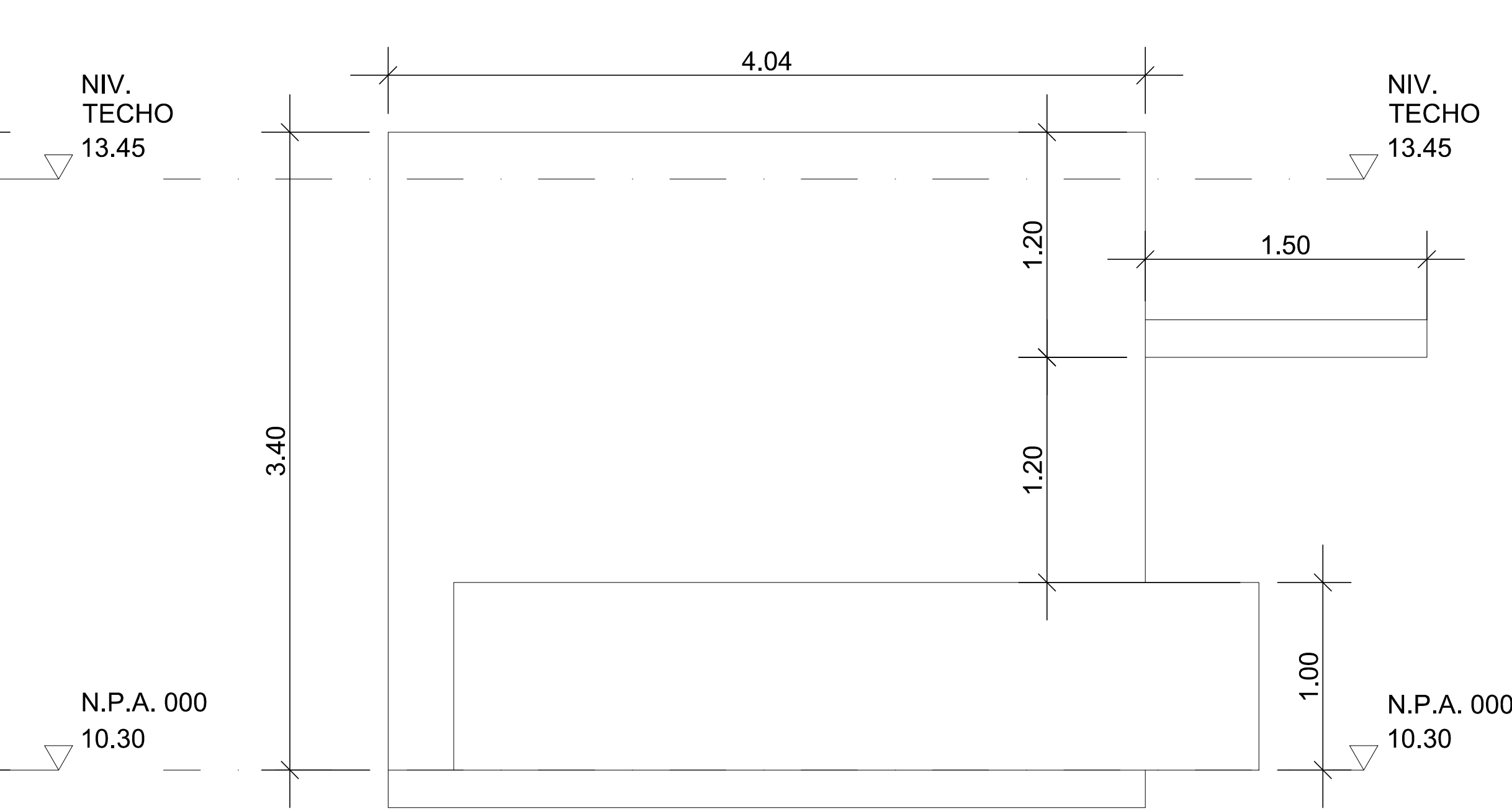
ELEVACIÓN LATERAL DERECHA
