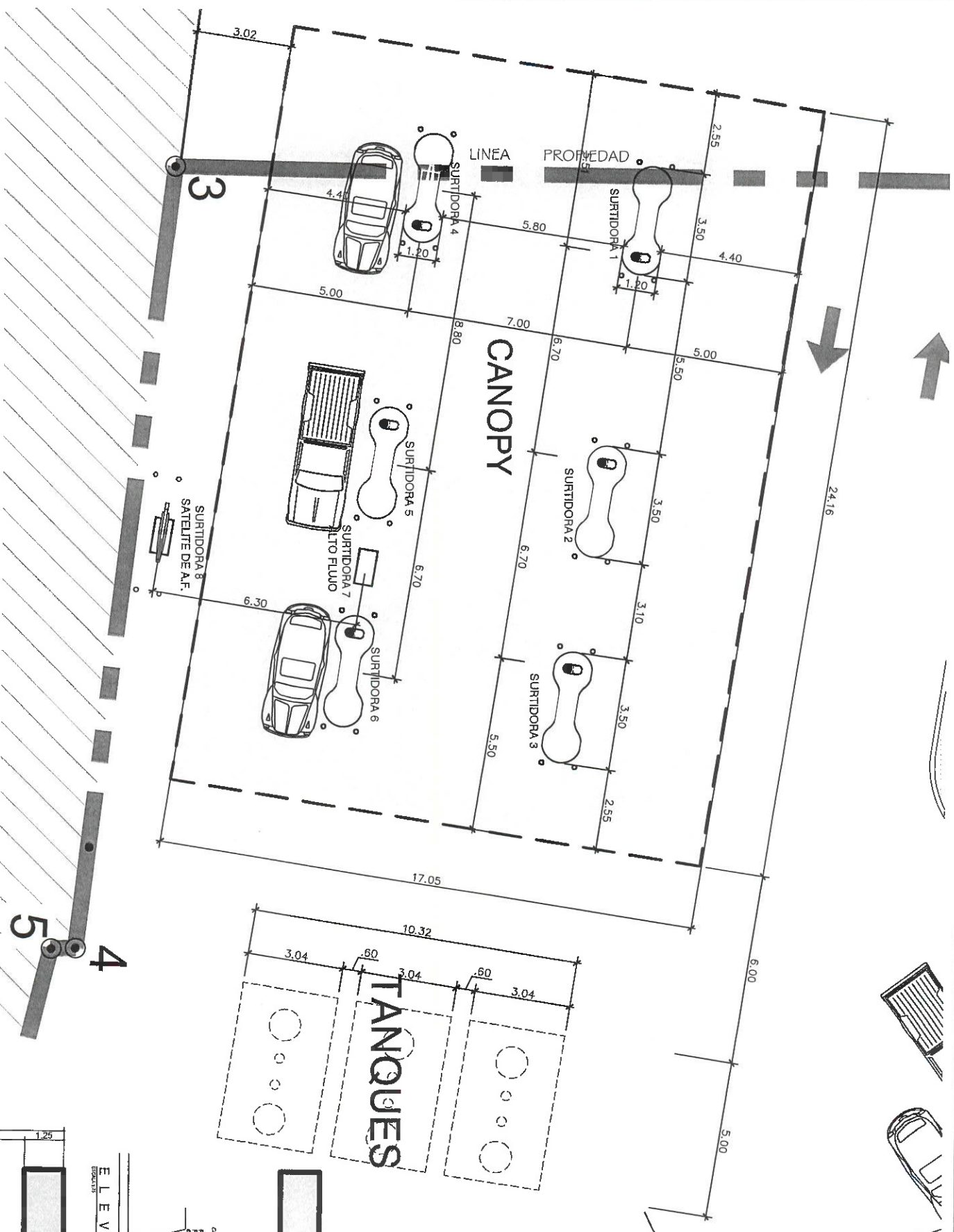
PLANTA DE CANOPY
