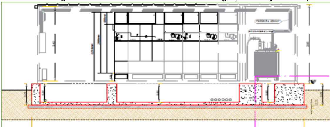
Imagen 4.1 Detalle de la estación de entrega ( Delivery Station)
