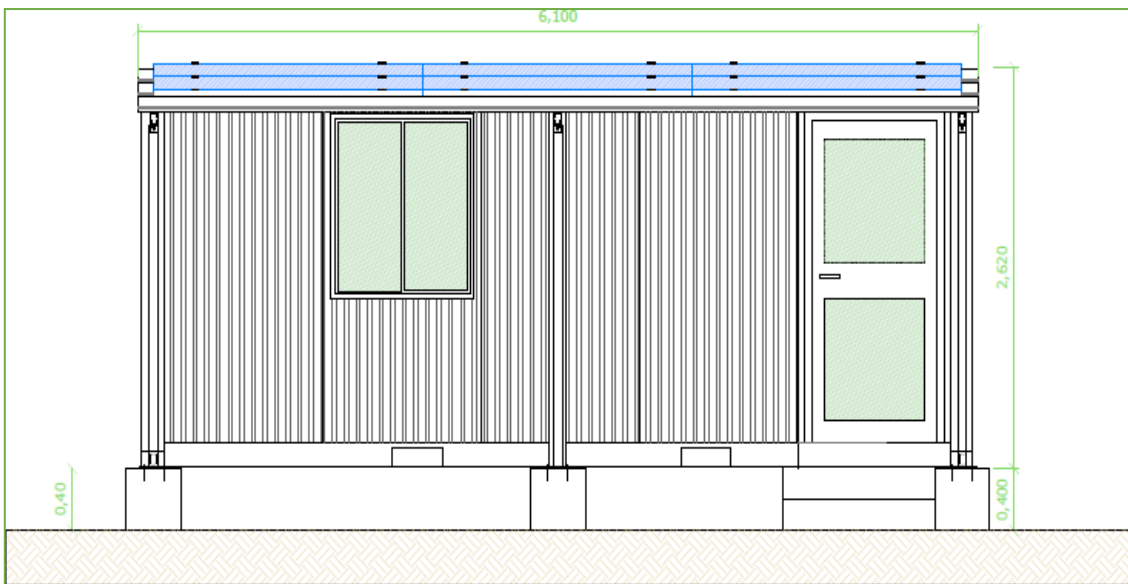
Imagen 4.13 Contenedor que alberga el sistema de control y monitoreo
