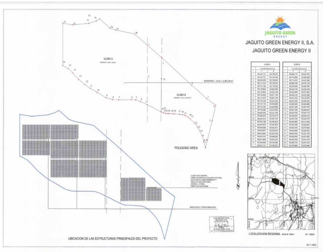
Plano N° 1. Proyecto “PLANTA FOTOVOLTAICA JAGÜTO GREEN ENERGY II”
